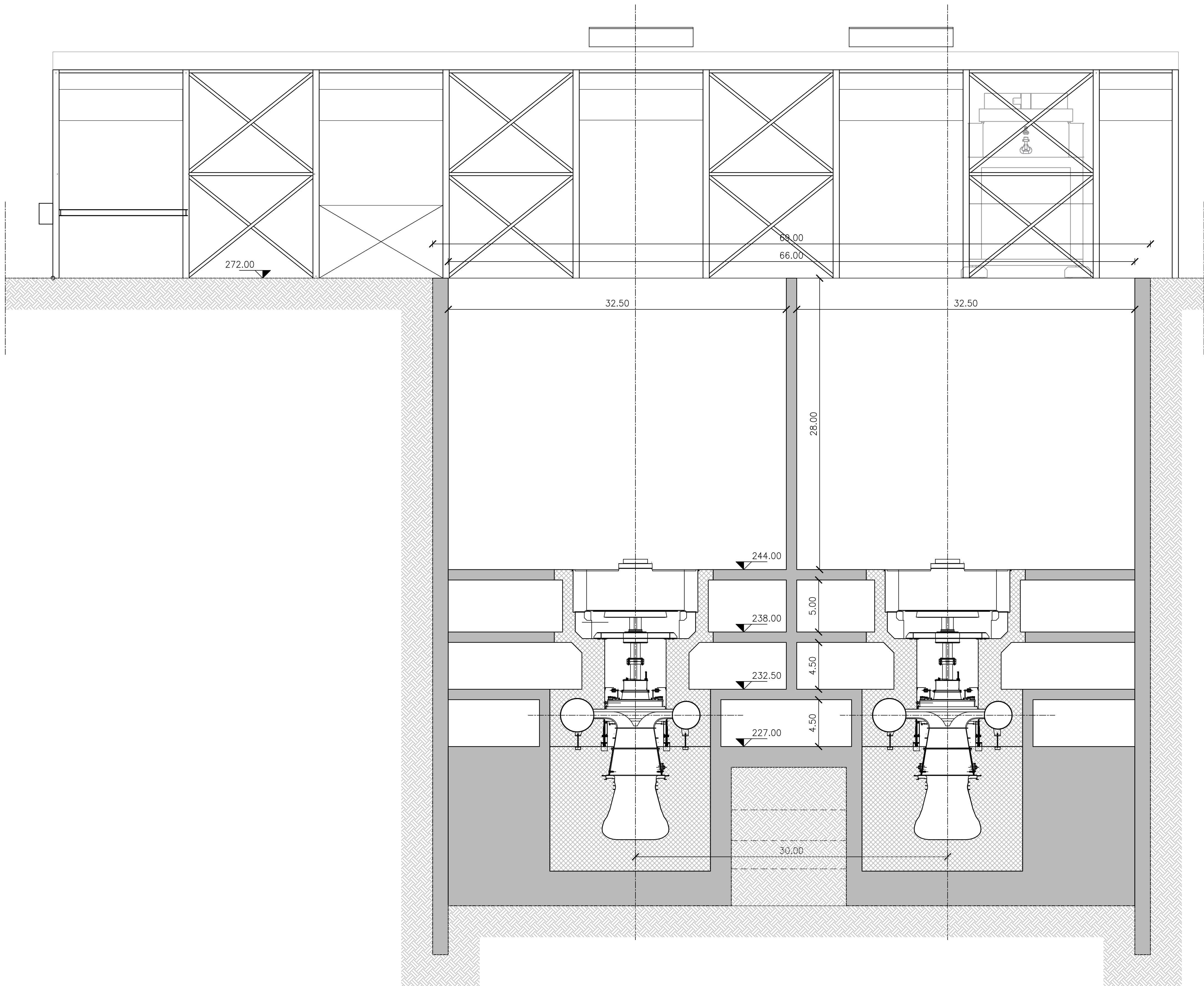
Sezione Longitudinale
