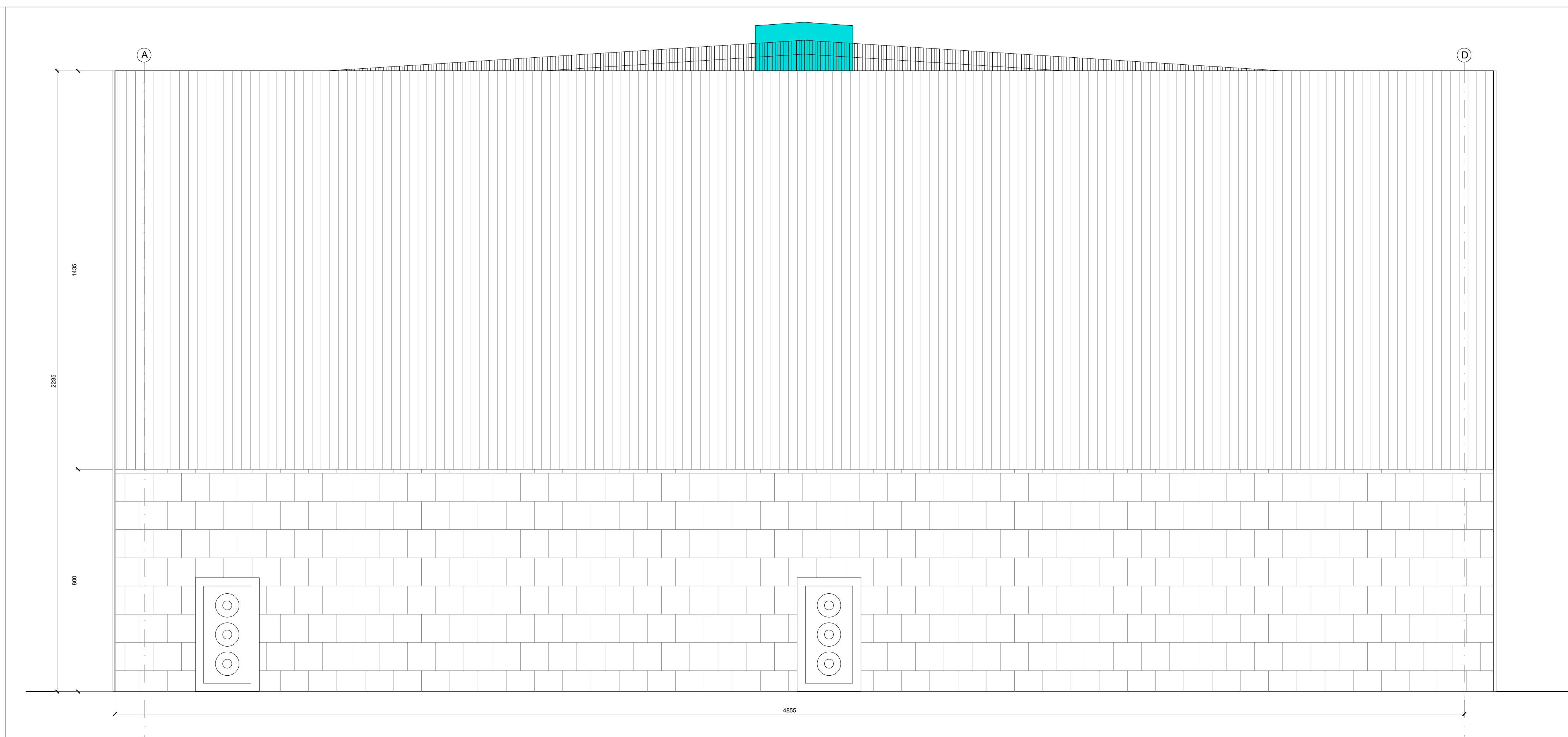
PROSPETTO ASSE 10
