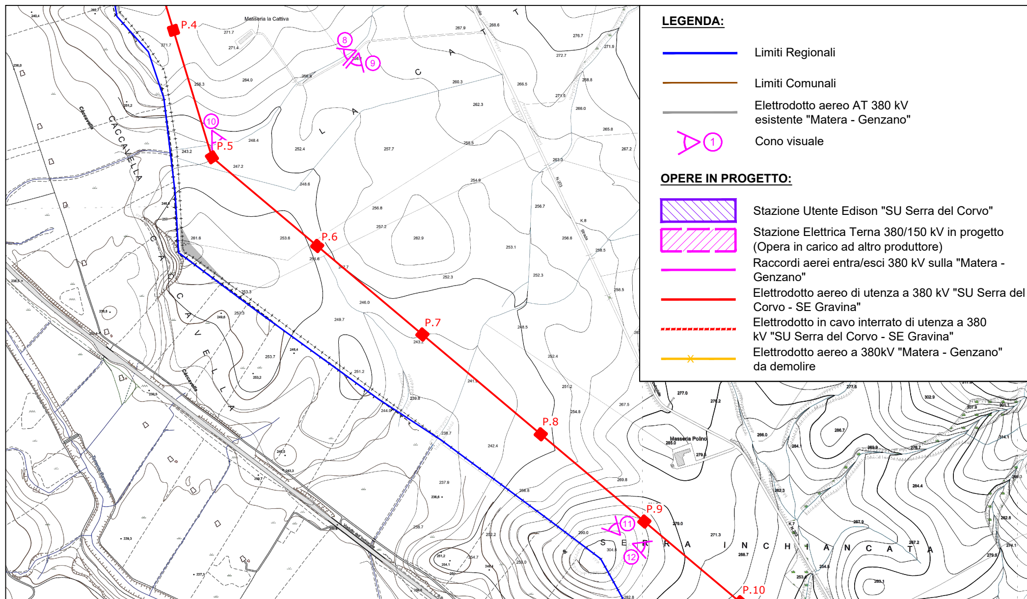
Planimetria coni visuale - rappresentazione non in scala
