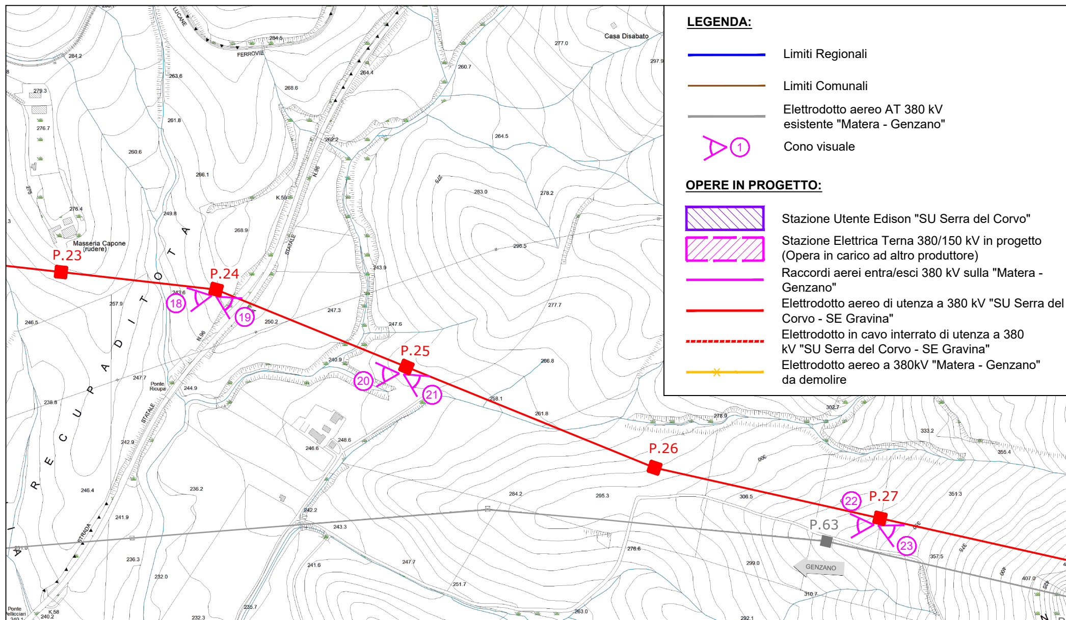
Planimetria coni visuale - rappresentazione non in scala
