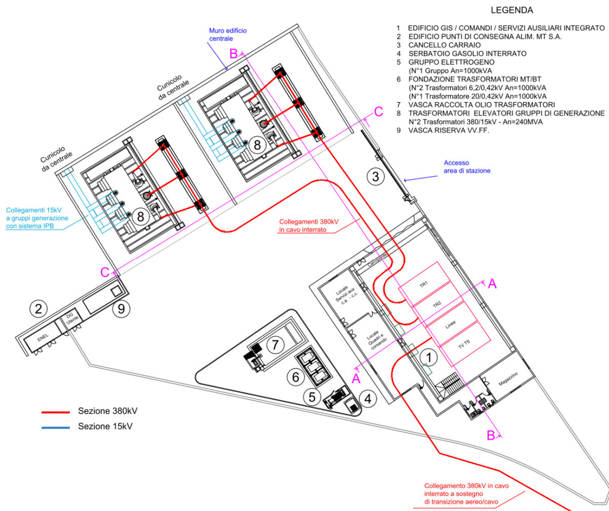
Planimetria elettromeccanica "SU Serra del Corvo"
