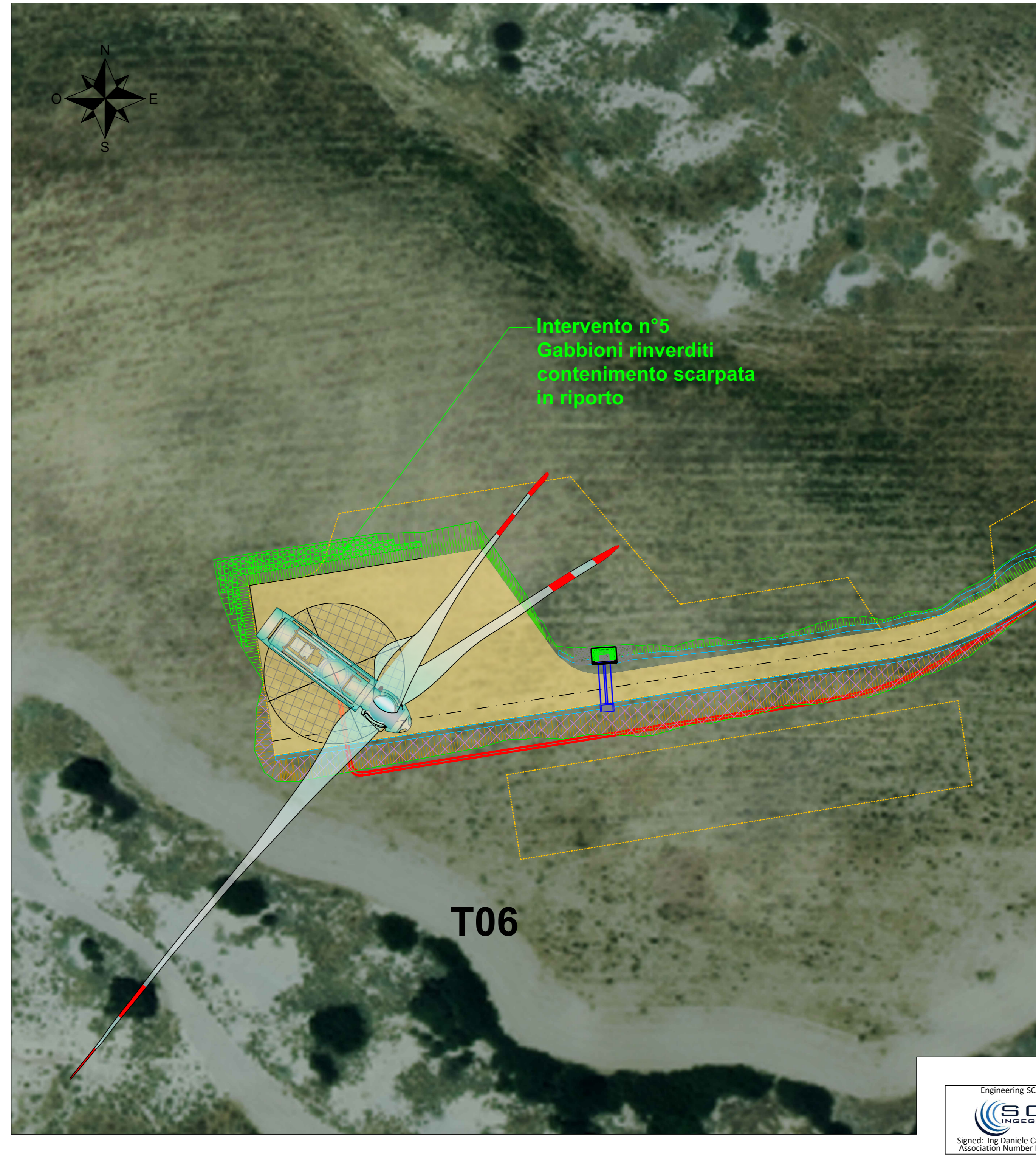
Intervento n°5 - Gabbioni rinverditi - Scala 1:500
