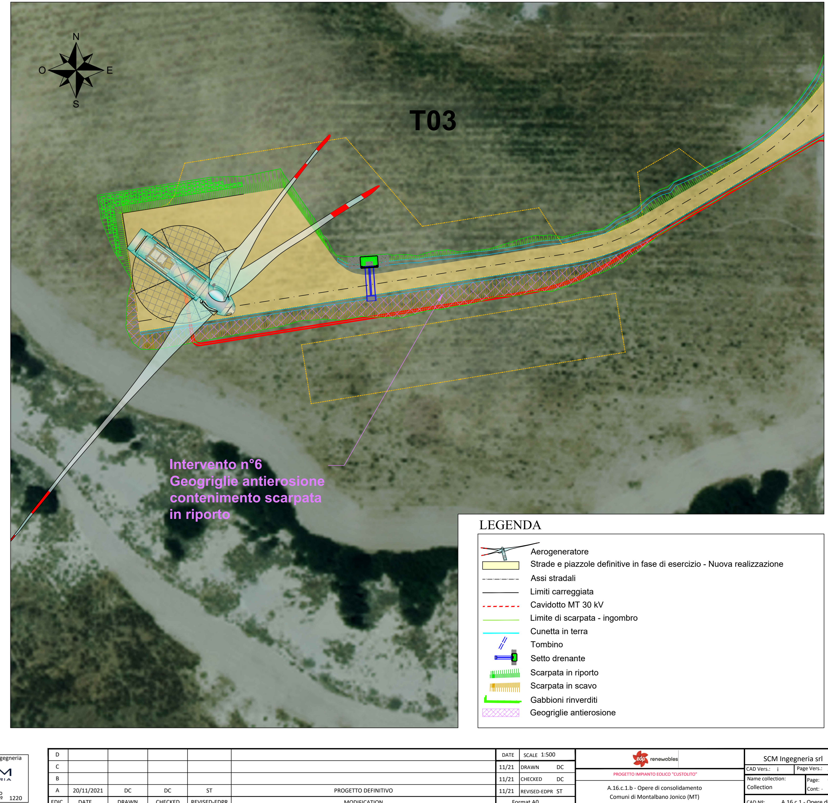
Intervento n°6 - Geogriglie antierosione - Scala 1:500
