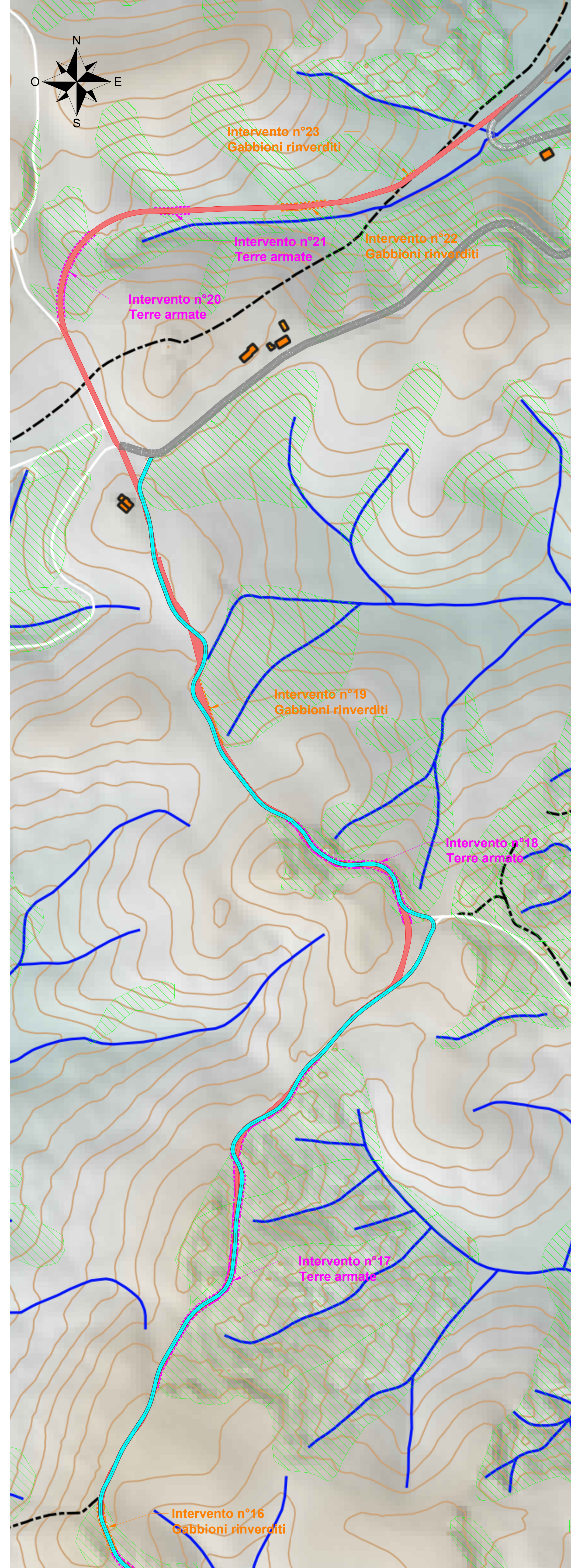
Inquadramento Vista D - Scala 1:2000
