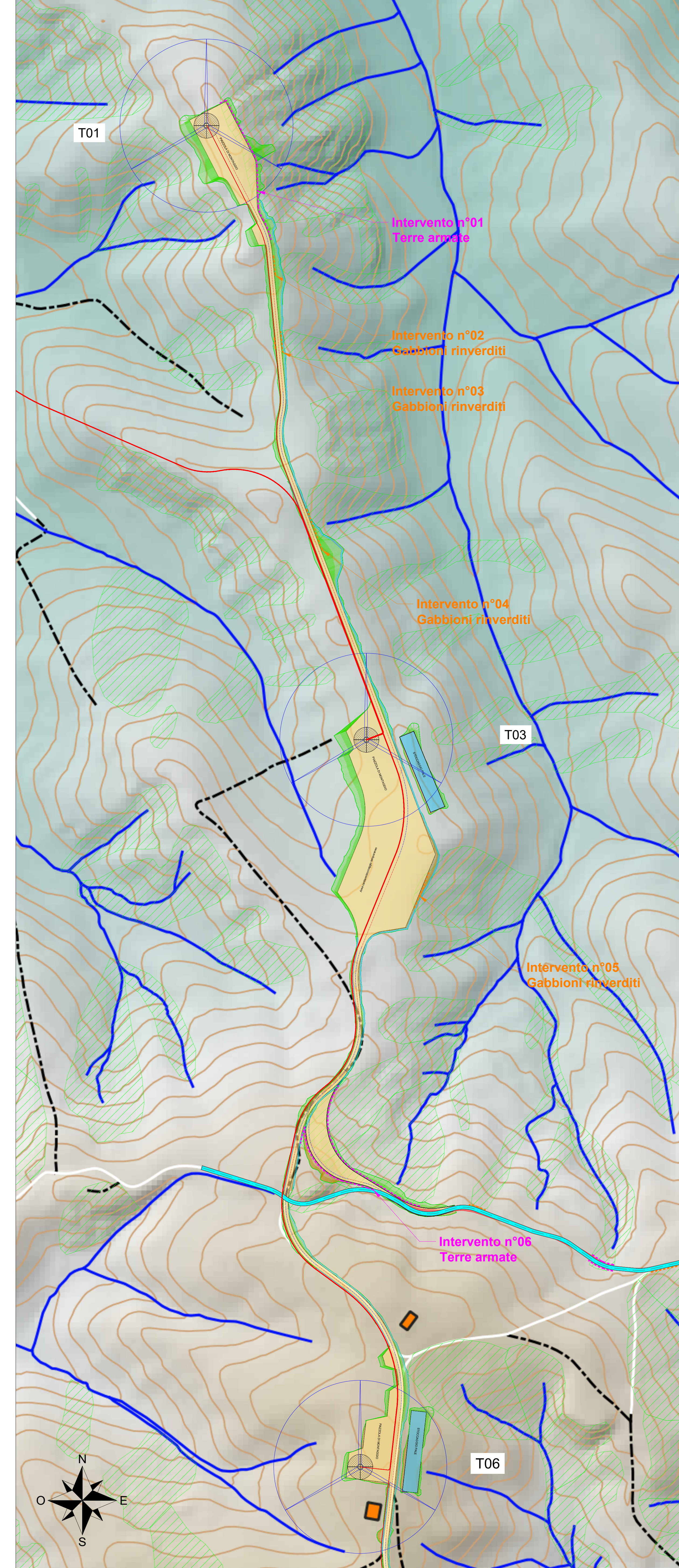
Inquadramento Vista A - Scala 1:2000
