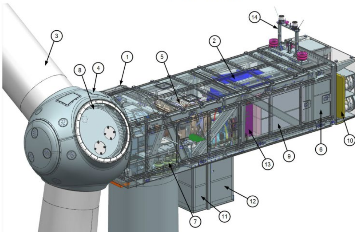
Figura 1: Schema descrittivo aerogeneratore
