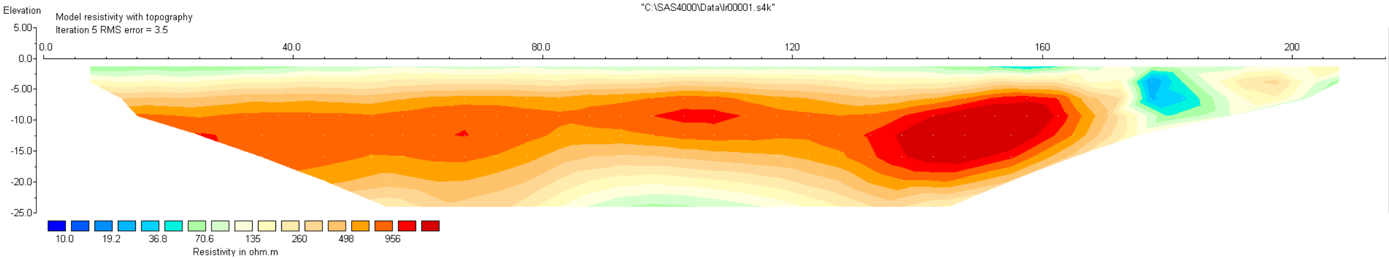
Fig. 26 SEZIONE ELETTROTOMOGRAFICA ERT1
