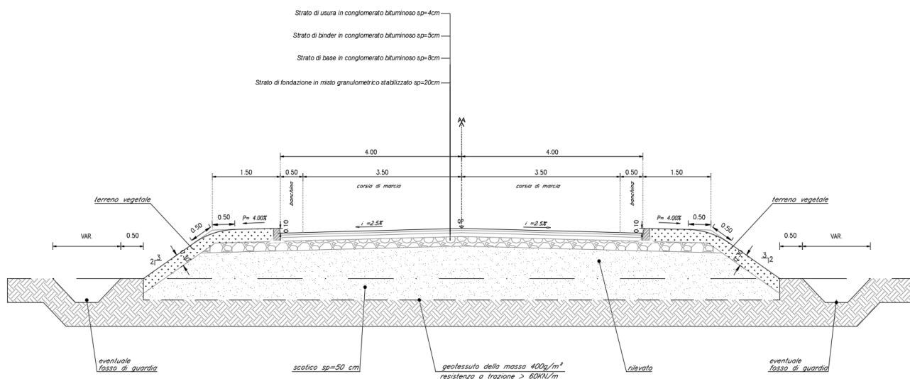
Figura 3 – Sezione tipo in rilevato Asse B
