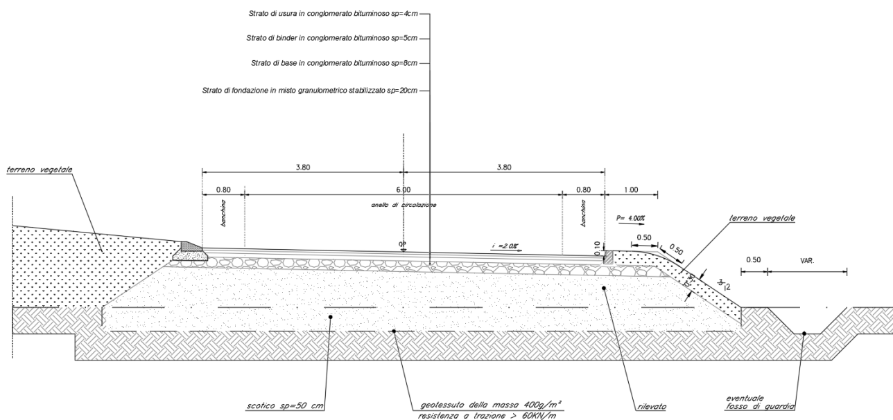
Figura 4 – Sezione tipo in rilevato rotatoria
