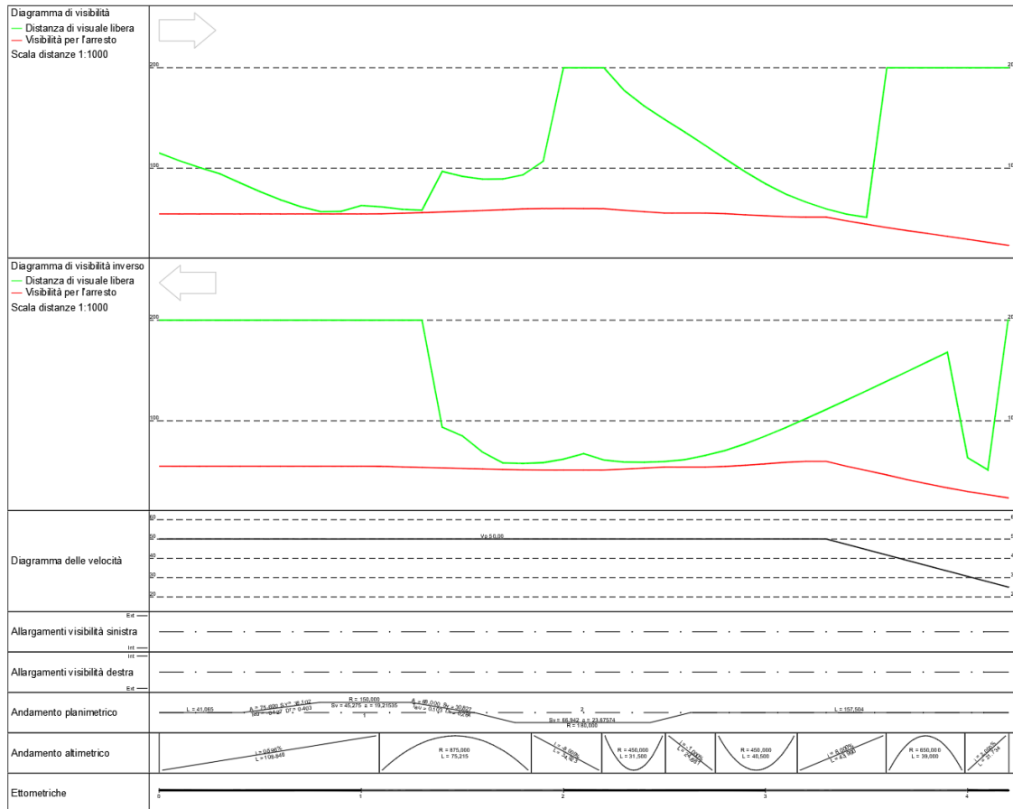
Figura 7 - Diagramma di visibilità - Asse A
