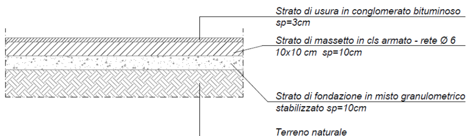
Figura 6 – Pacchetto pista ciclopedonale
