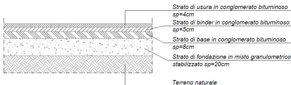
Figura 5 – Pacchetto pavimentazione stradale asse A e asse B
