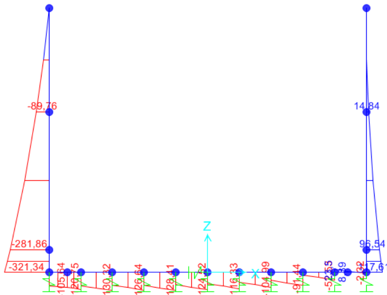
Figura 26: T - SISMA
