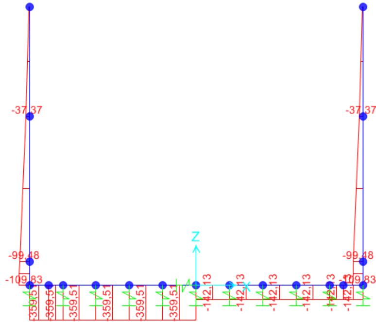
Figura 25: N - SISMA
