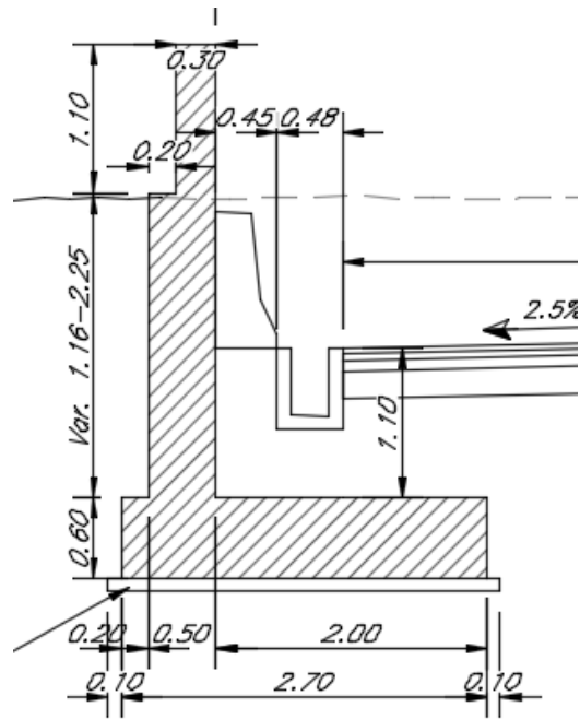
Figura 3: Sezione trasversale
