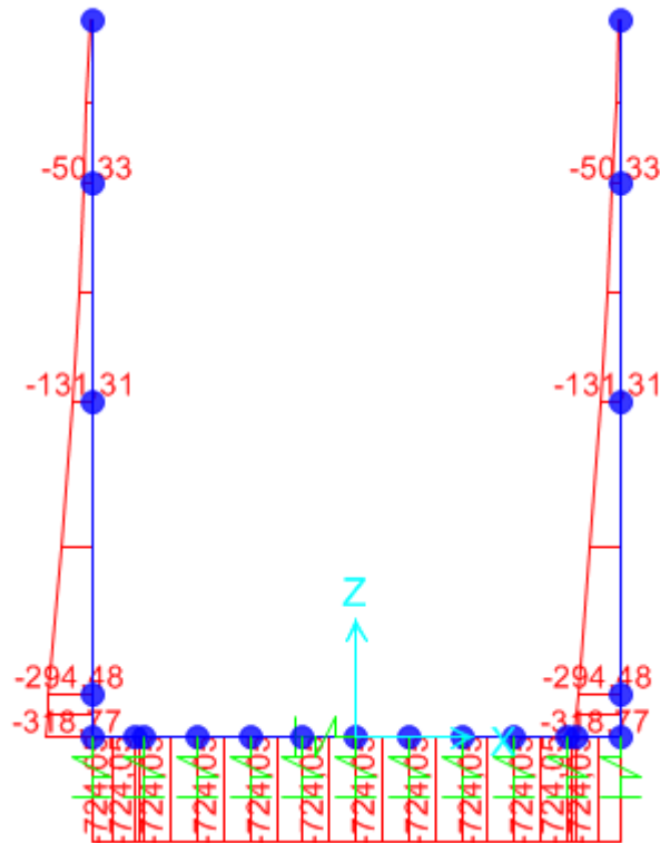
Figura 10: N - SLU
