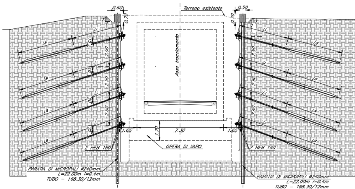
Figura 1: Sezione di studio paratia
