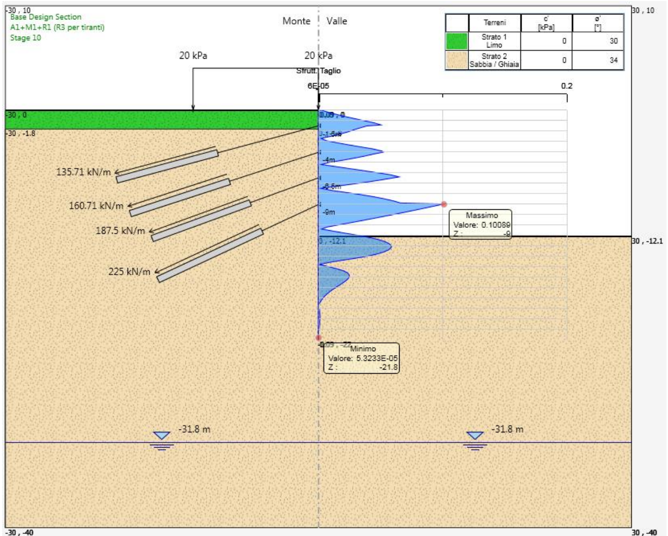
Figura 17 – Diagramma di sfruttamento a taglio (involoppo)
