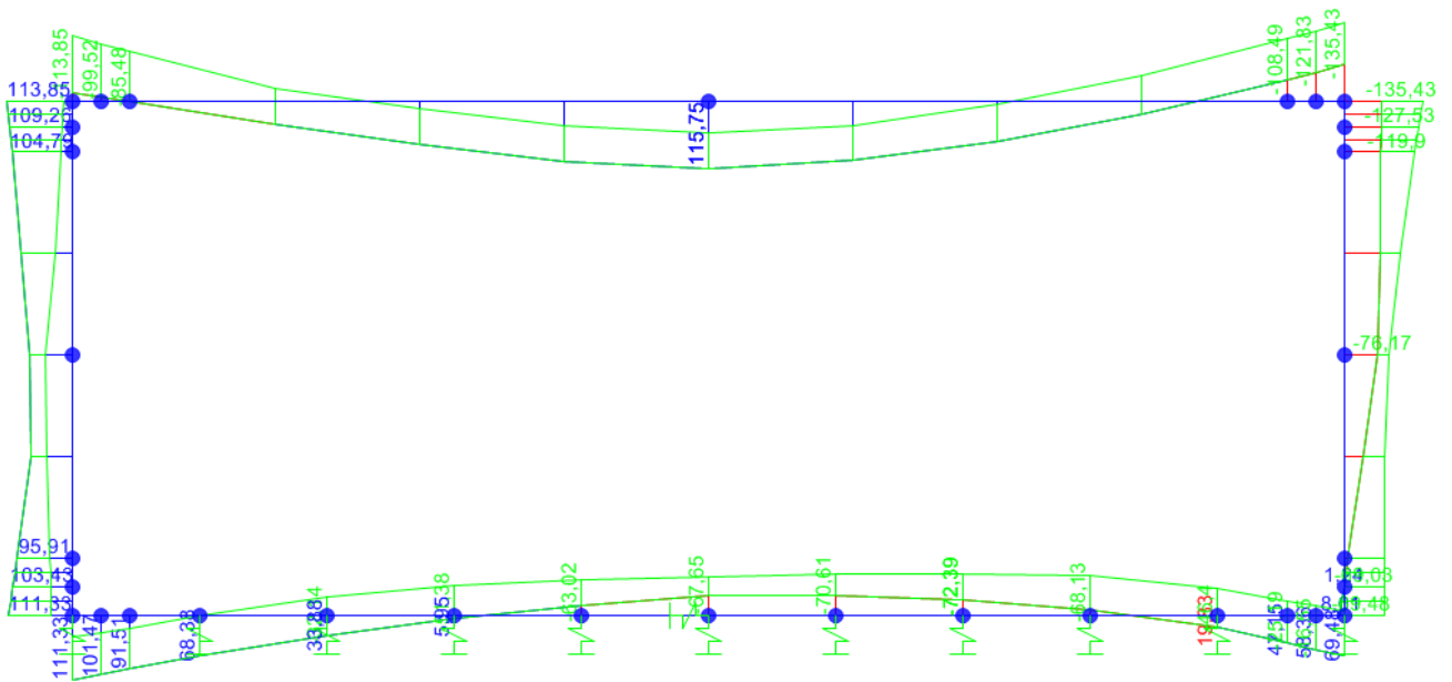
Figura 27: Involuppo M – SLE RARA
