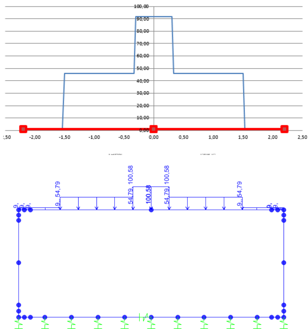
Figura 13: Carico dal traffico (TANDEM + carico distribuito da 9kN/m2)( Caso ACC1)
