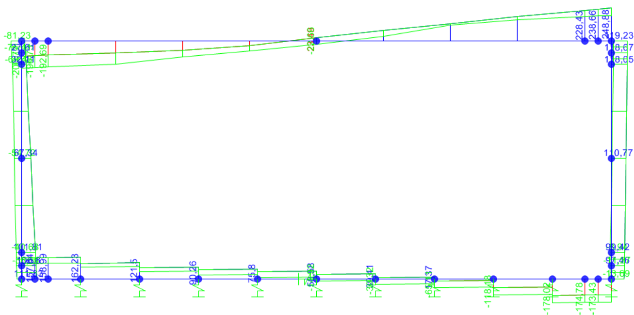
Figura 21: Involuppo N - SLU
