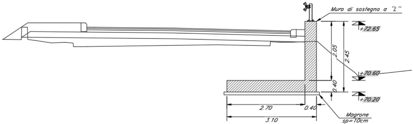
Figura 2: Sezione trasversale muro di sostegno
