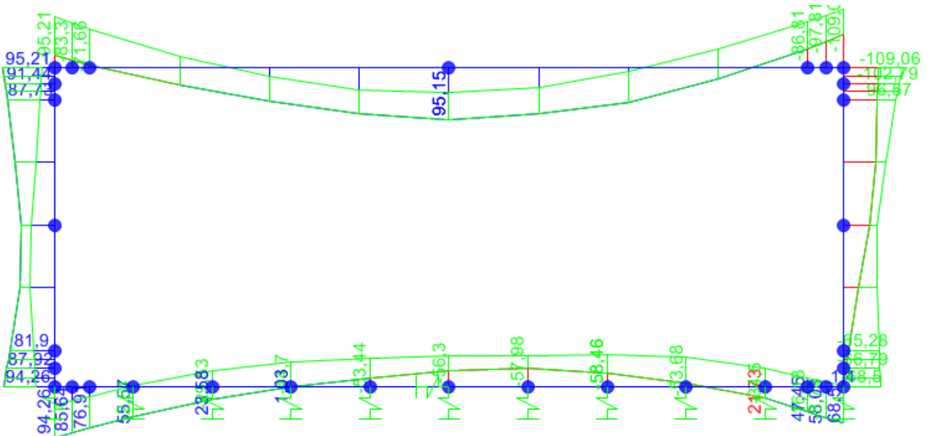
Figura 29: Involuppo M – SLE FREQ
