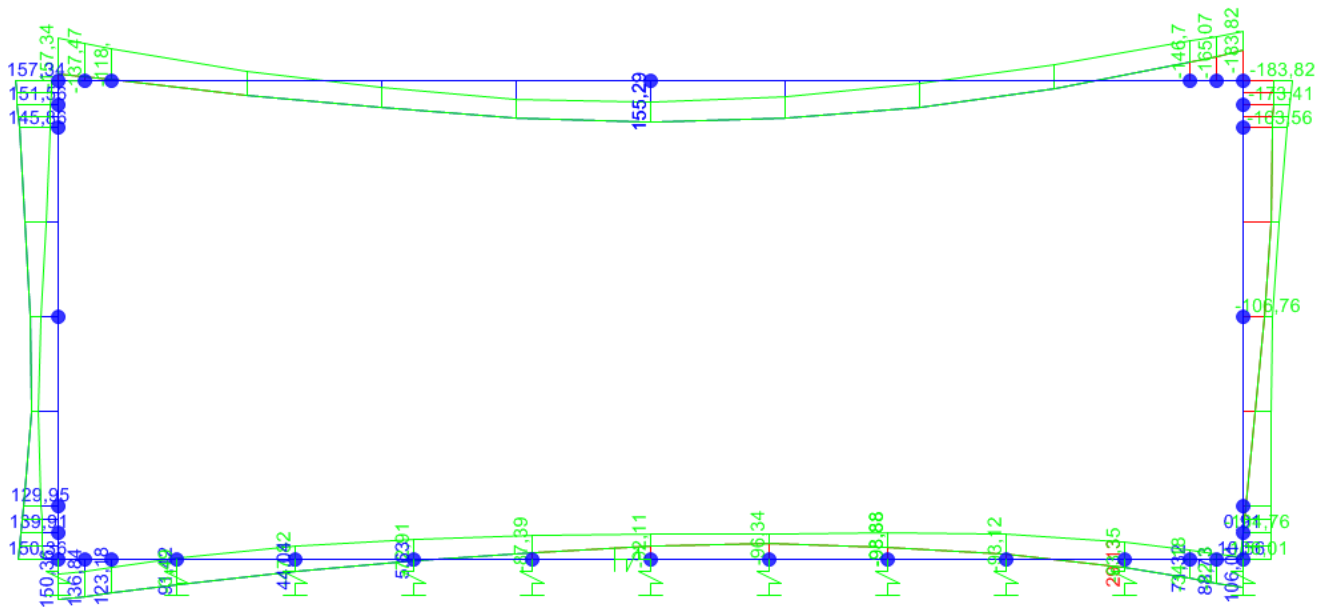
Figura 26: Involuppo M - SLU
