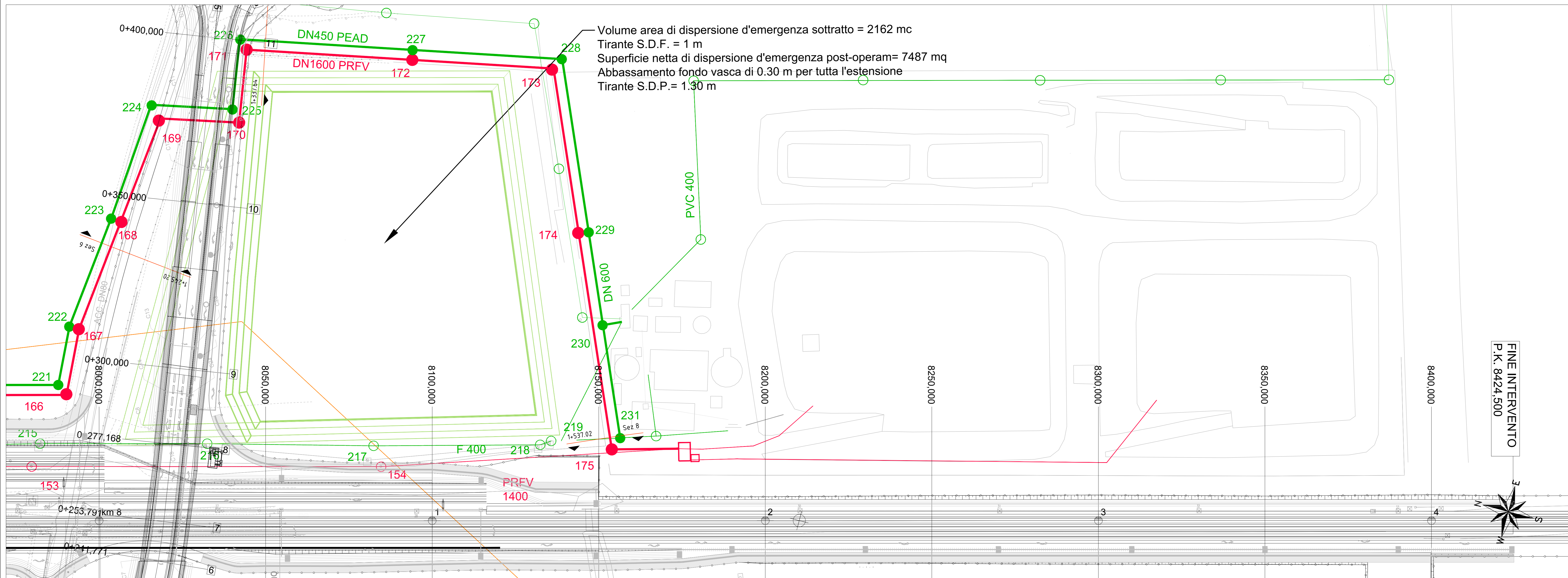
PLANIMETRIA FOGNATURA BIANCA E NERA - STATO DI PROGETTO - 4/4 - SCALA 1:500
