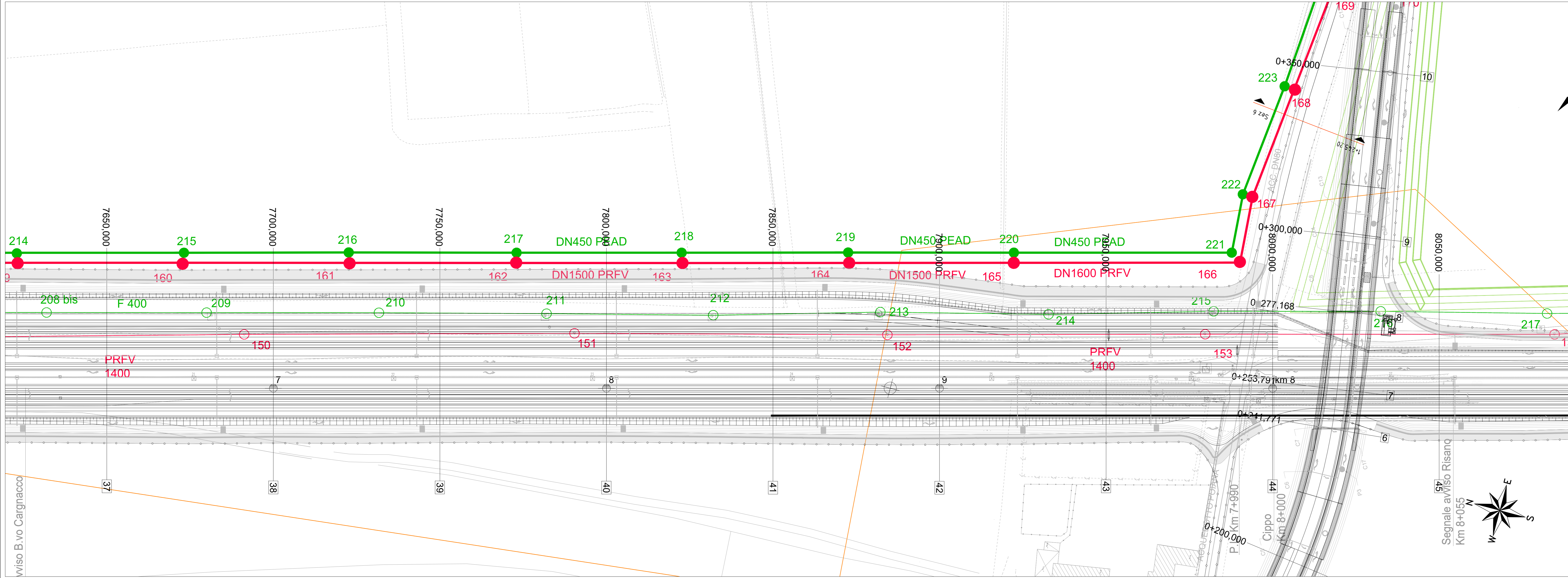
PLANIMETRIA FOGNATURA BIANCA E NERA - STATO DI PROGETTO - 3/4 - SCALA 1:500
