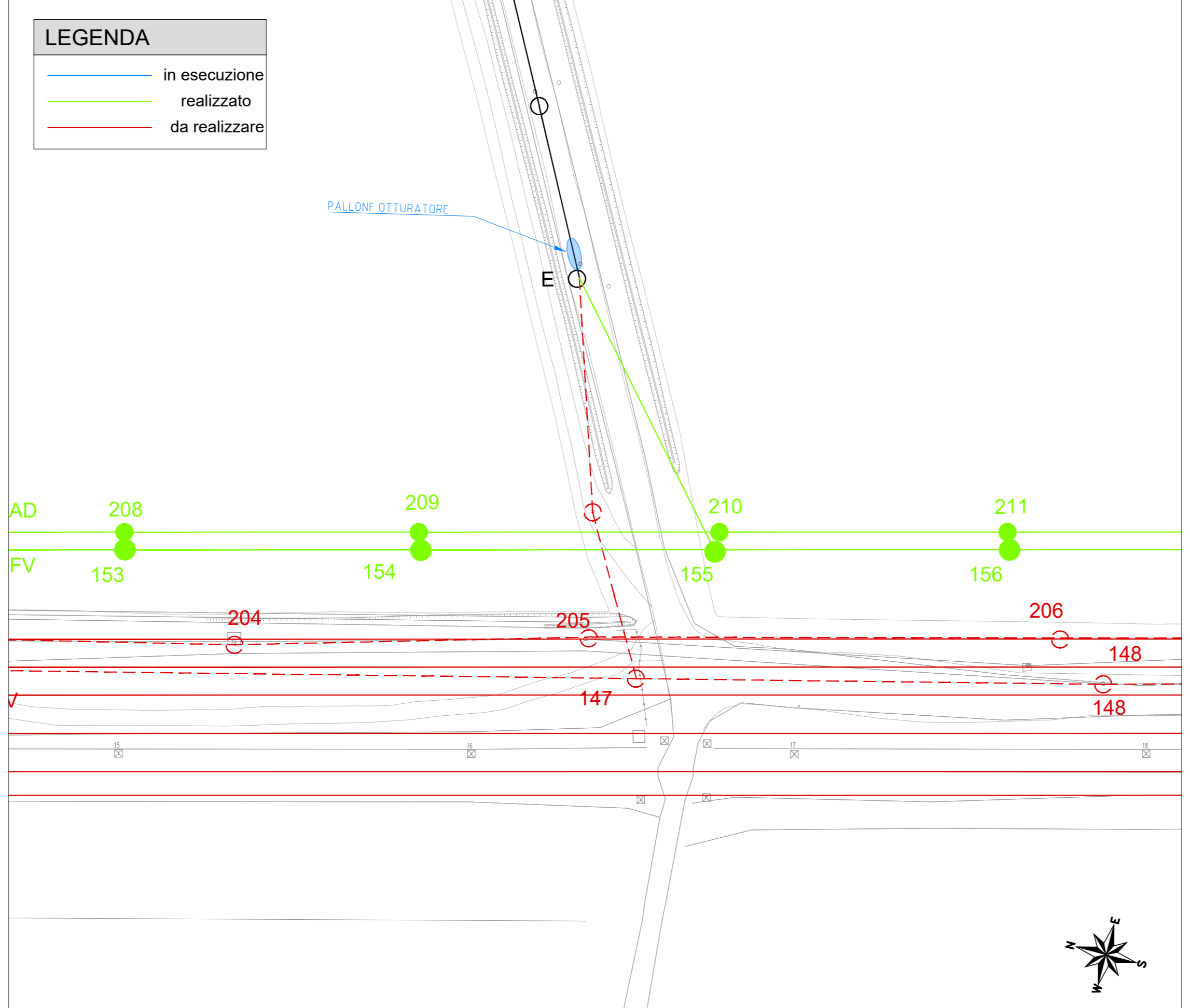
PLANIMETRIA FASI DI REALIZZAZIONE FOGNATURA BIANCA E NERA - SCALA 1:2000
