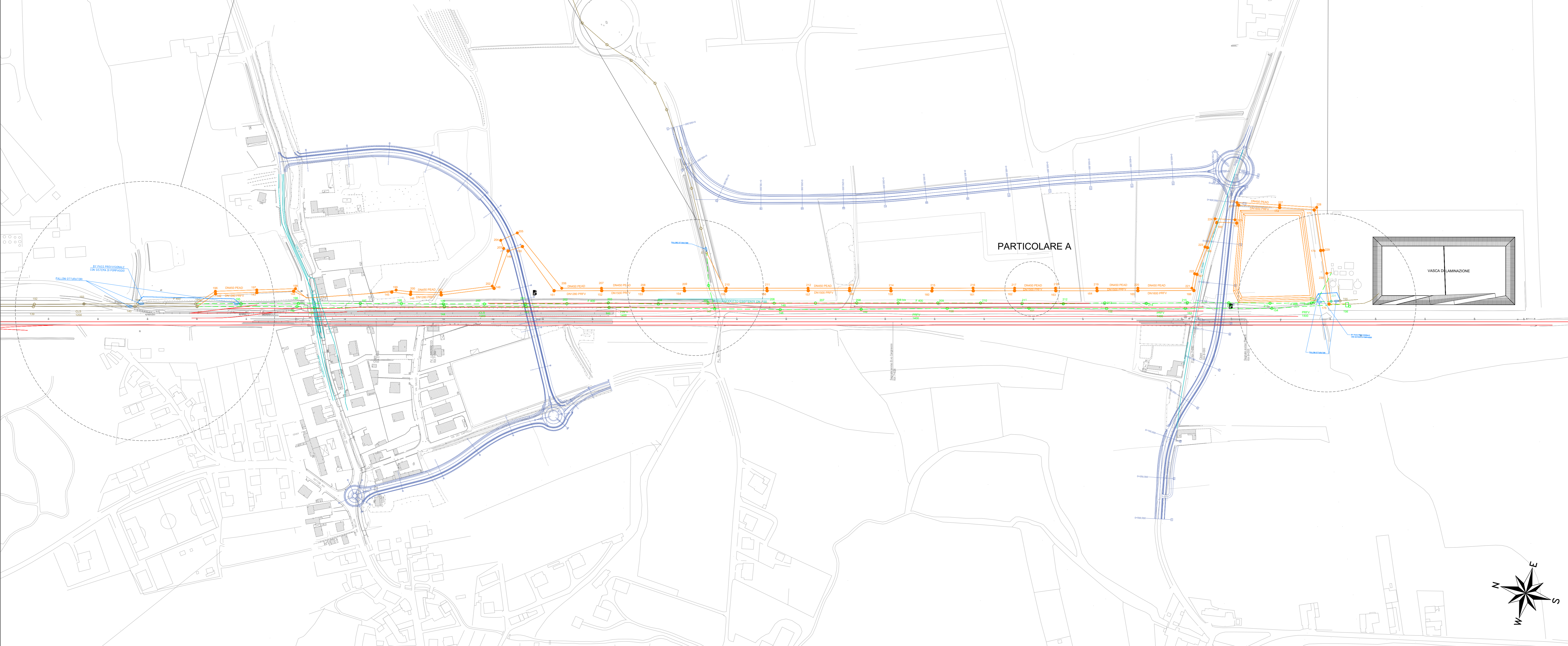
PLANIMETRIA FASI DI REALIZZAZIONE FOGNATURA BIANCA E NERA - SCALA 1:2000
