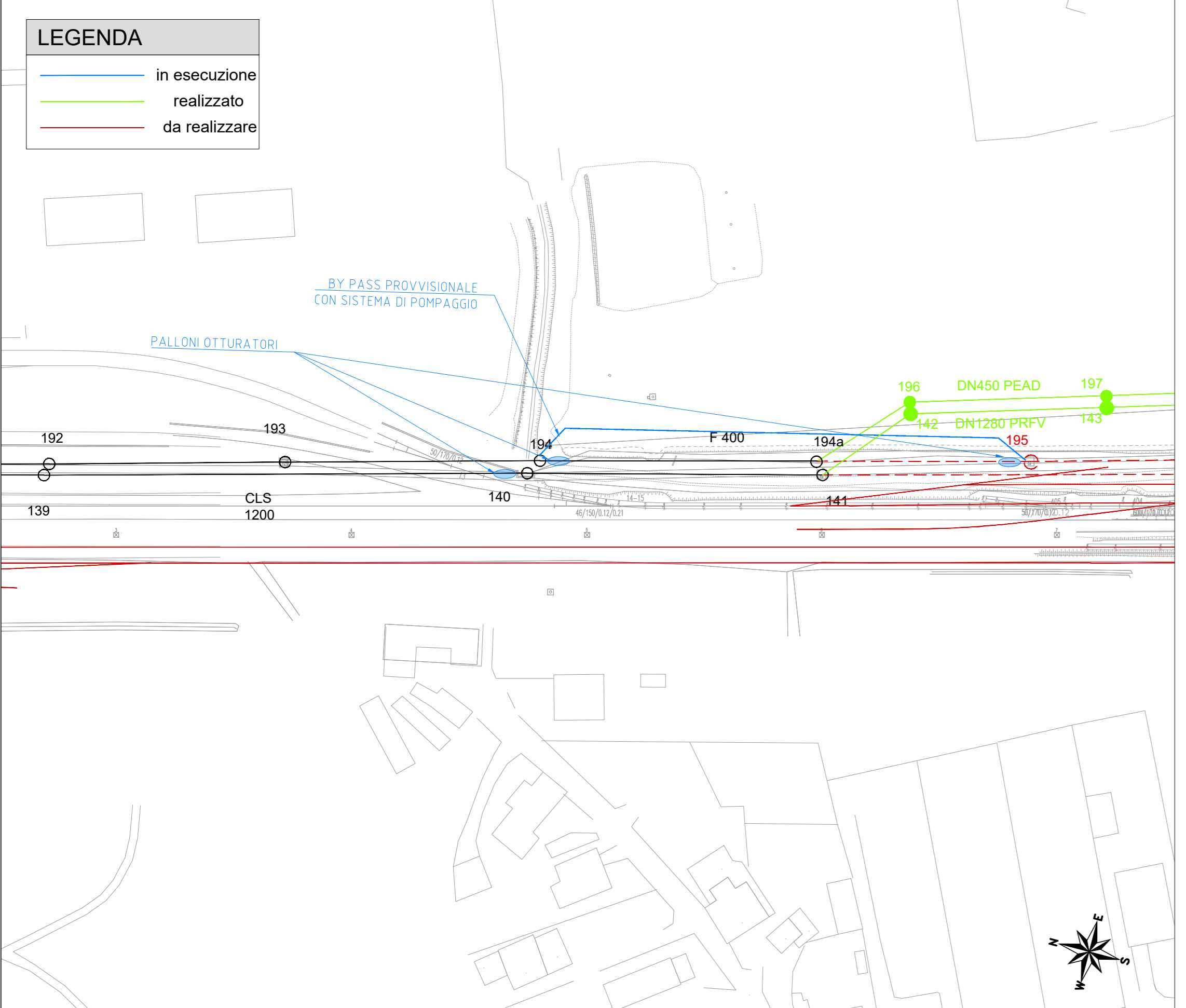
FASE DI REALIZZAZIONE 2 - ZONA NORD
