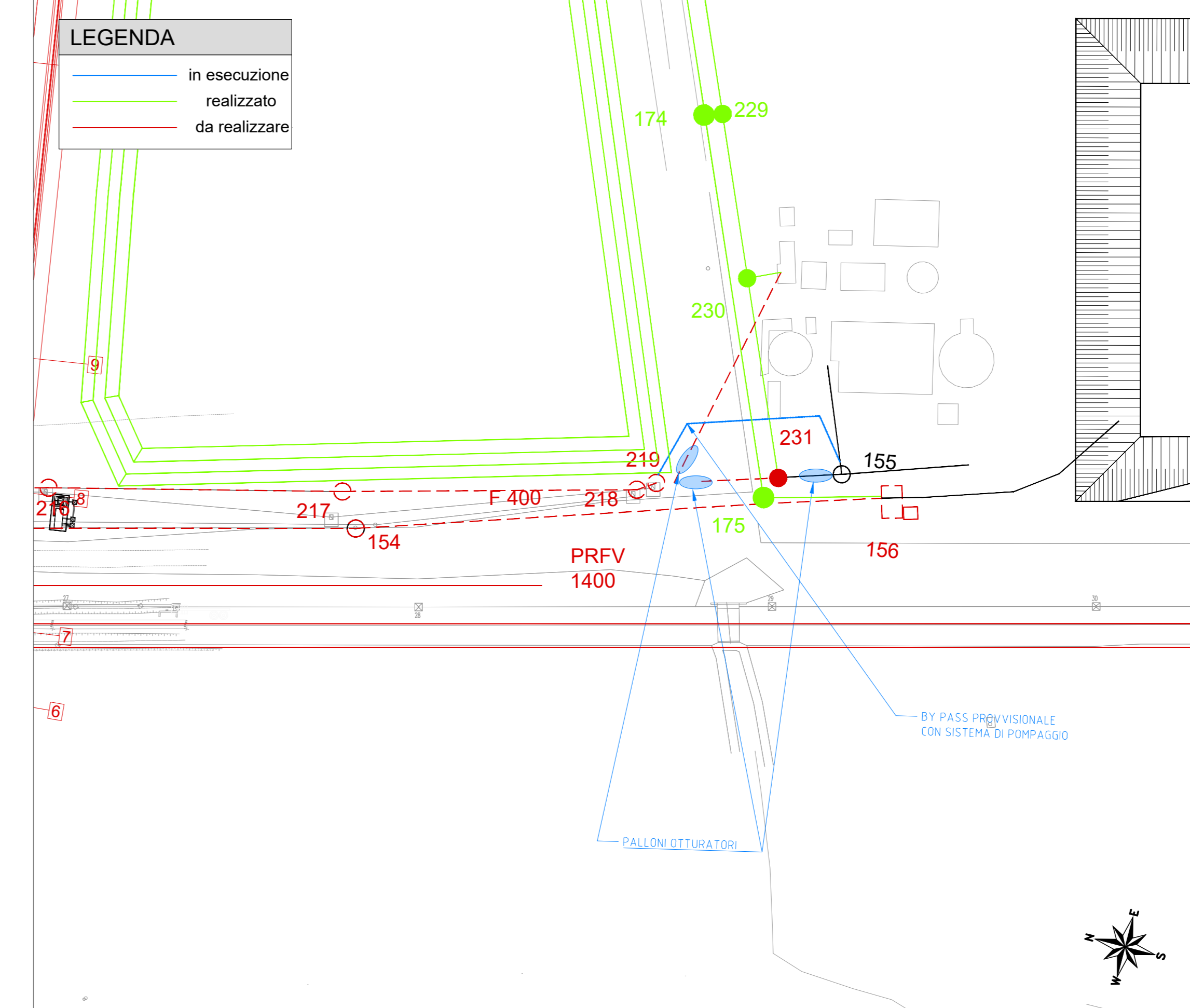
FASE DI REALIZZAZIONE 2 - ZONA SUD
