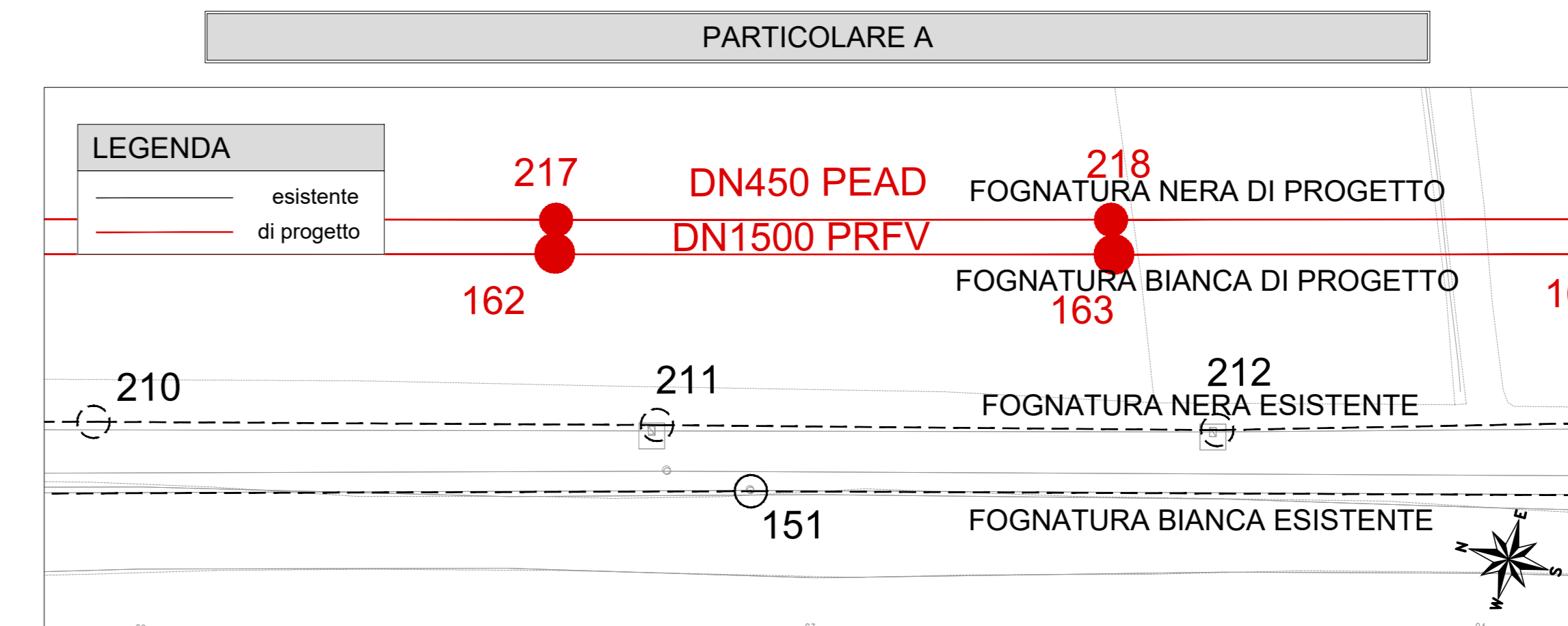
FASE DI REALIZZAZIONE 2 - ZONA SUD
