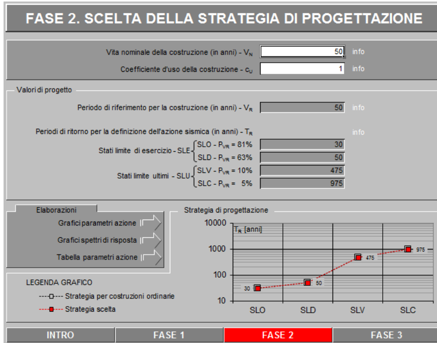
Figura 8 - Scelta della strategia di progettazione (Fase 2)
