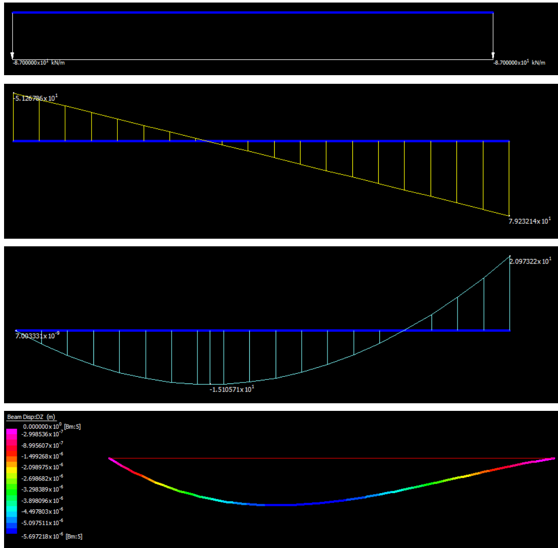
Figura 16 - Sollecitazioni derivanti dal modello della fondazione
