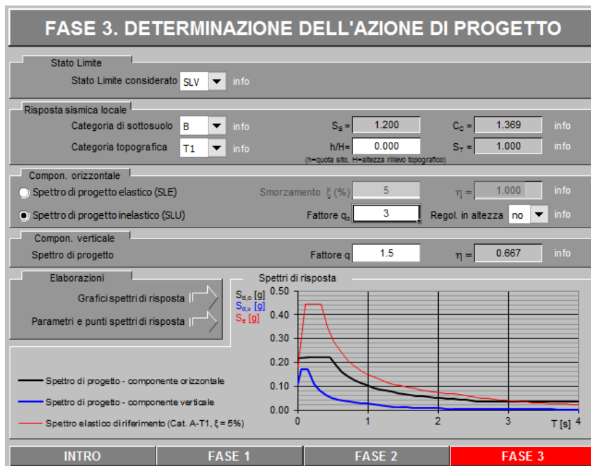
Figura 9 - Determinazione dell'azione di progetto (Fase 3)
