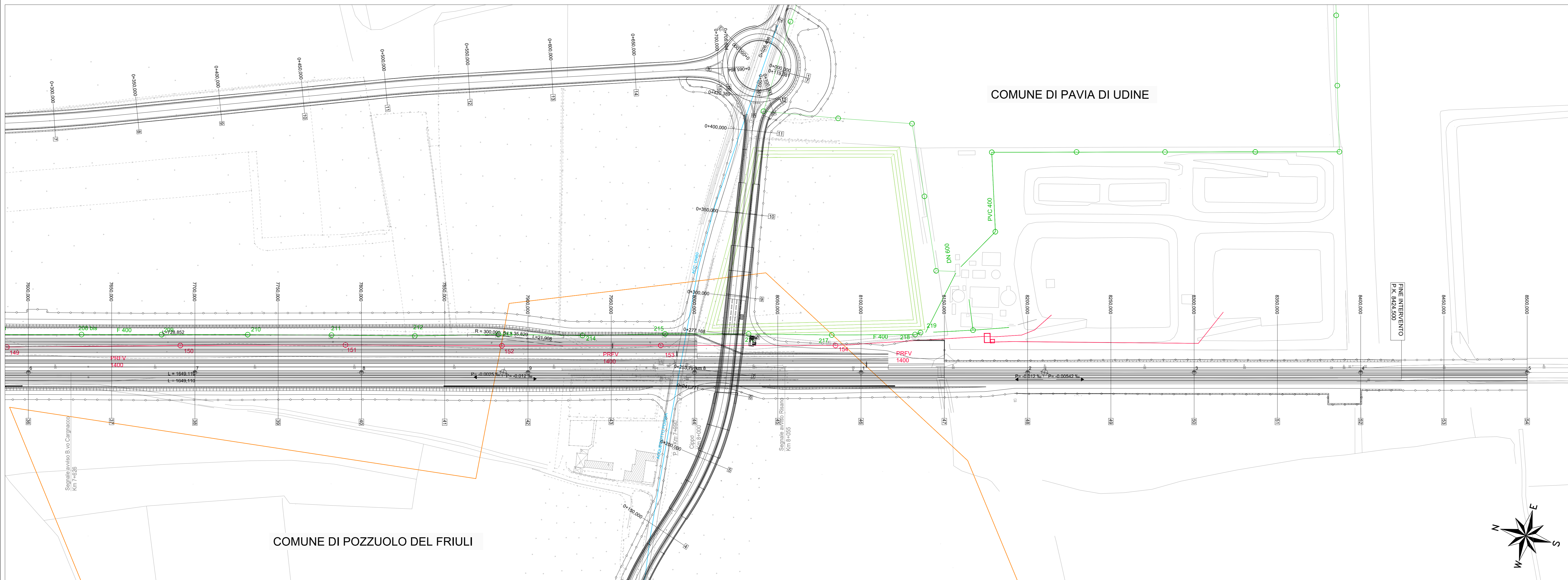
PLANIMETRIA DEI SOTTOSERVIZI 2/2 - SCALA 1:1000
