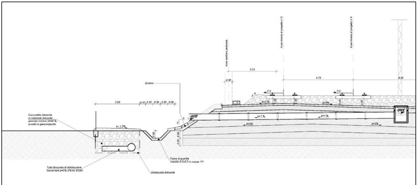
Figura 6-2- Sezione A-A illustrativa del recapito delle acque di piattaforma al cassetto drenante in rilevato.
