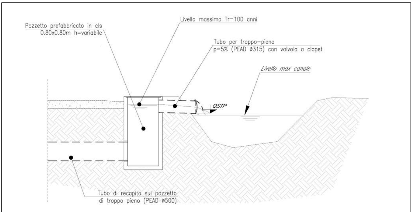
Figura 6-3- Sezione B-B illustrativa del recapito delle acque dal cassetto drenante al canale irriguo più vicino.
