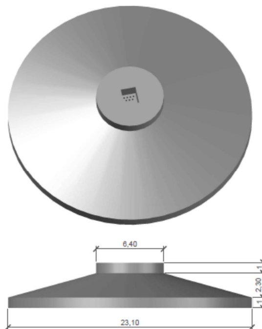
Figura 1 Fondazione Tipo
