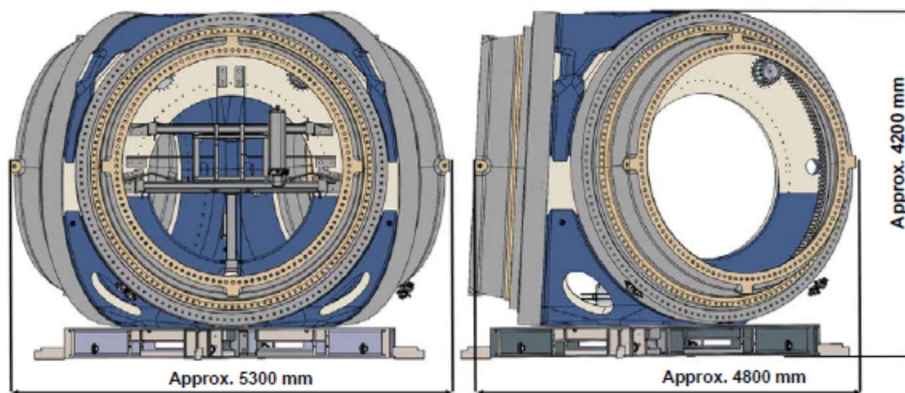
Figura 9 Mozzo (Hub)
