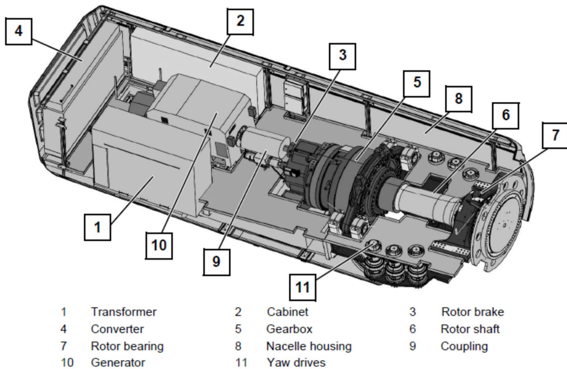
Figura 11 Navicella e sua composizione interna tipo Vestas V162 o similare
