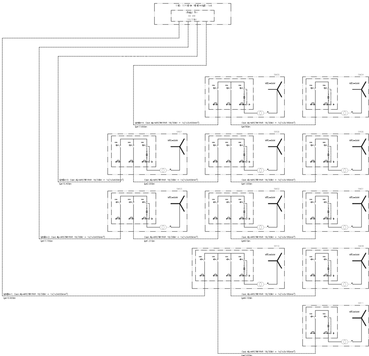
Figura 12 Schema elettrico MT aerogeneratori di progetto
