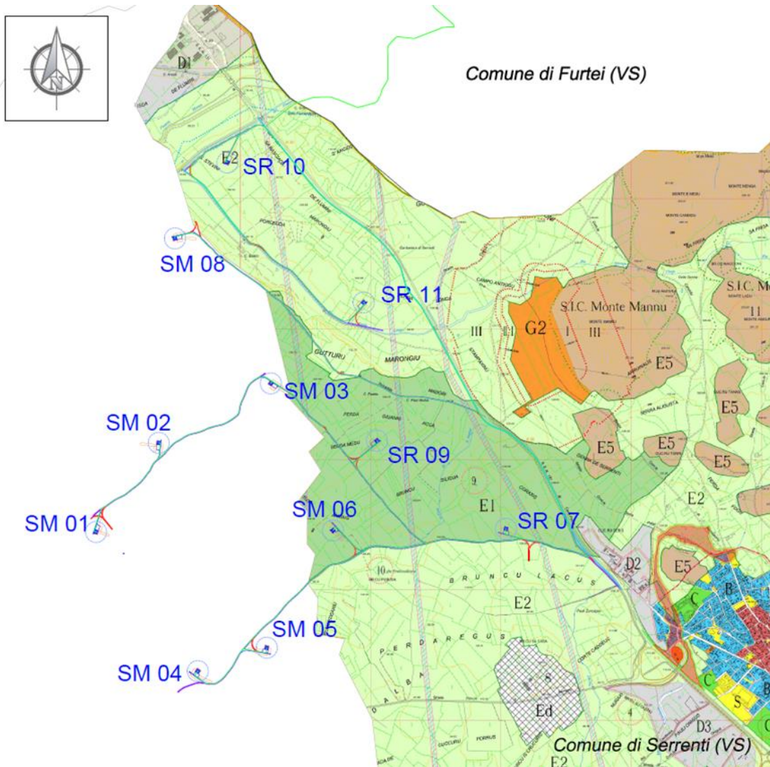
Figura 37 - Tav.Os.PPR.B1-Territorio (Particolare Area di impianto) del Piano Urbanistico Comunale di Serrenti
