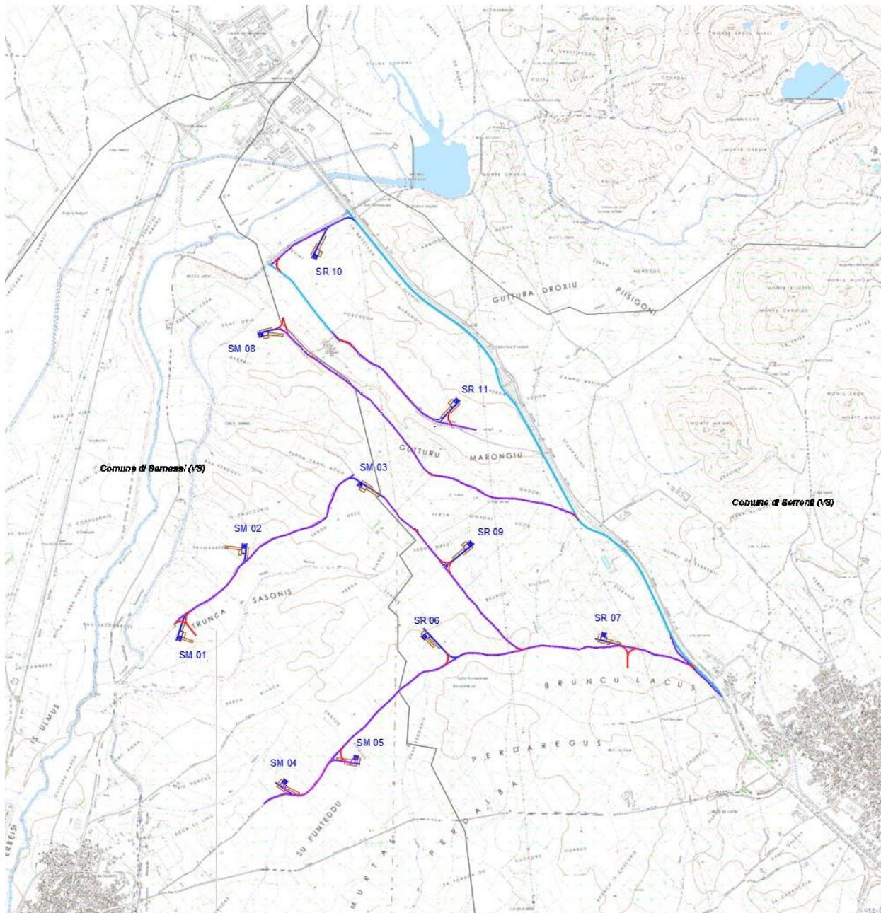
Figura3c - Inquadramento impianto eolico su CTR
