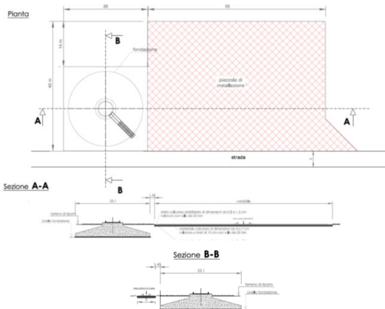
Figura 2 – Piazzola definitiva tipo (pianta e sezioni)
