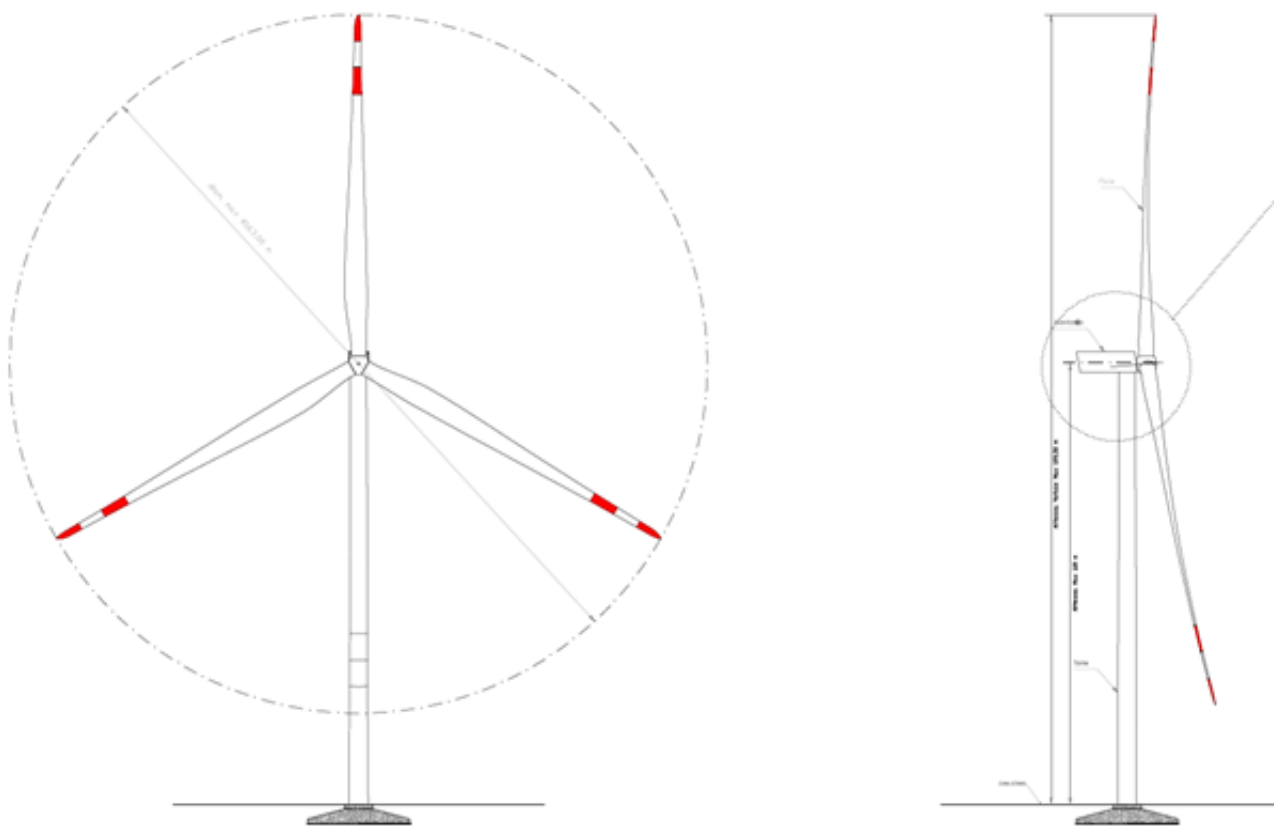
Figura 1 – Aerogeneratori tipo
