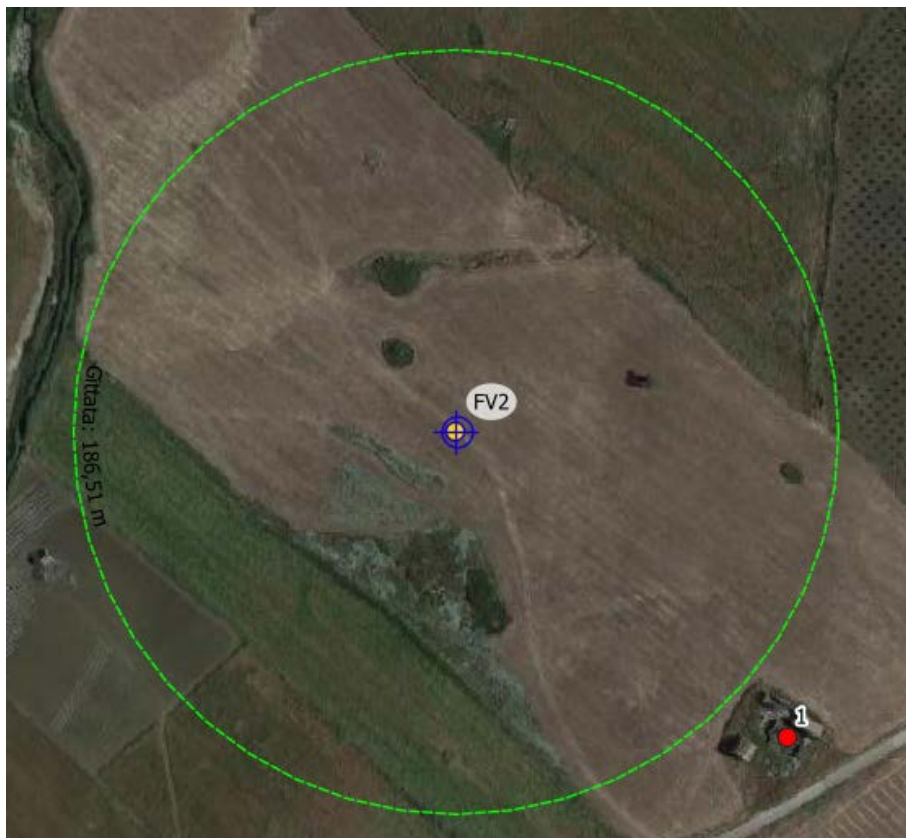
Figura 7-2 – Analisi degli effetti della rottura degli organi rotanti, aerogeneratore FV2
