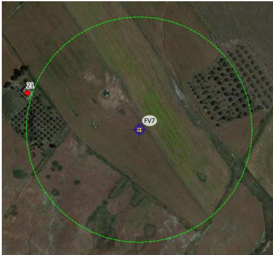
Figura 7-7 – Analisi degli effetti della rottura degli organi rotanti, aerogeneratore FV7
