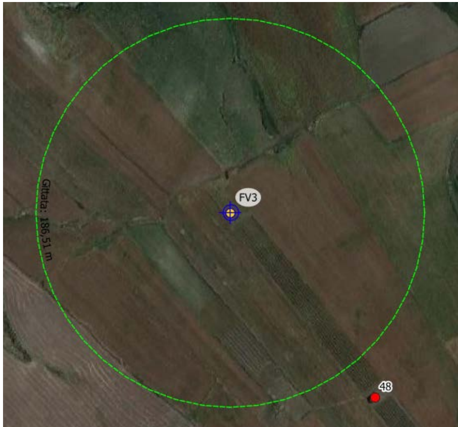
Figura 7-3 – Analisi degli effetti della rottura degli organi rotanti, aerogeneratore FV3
