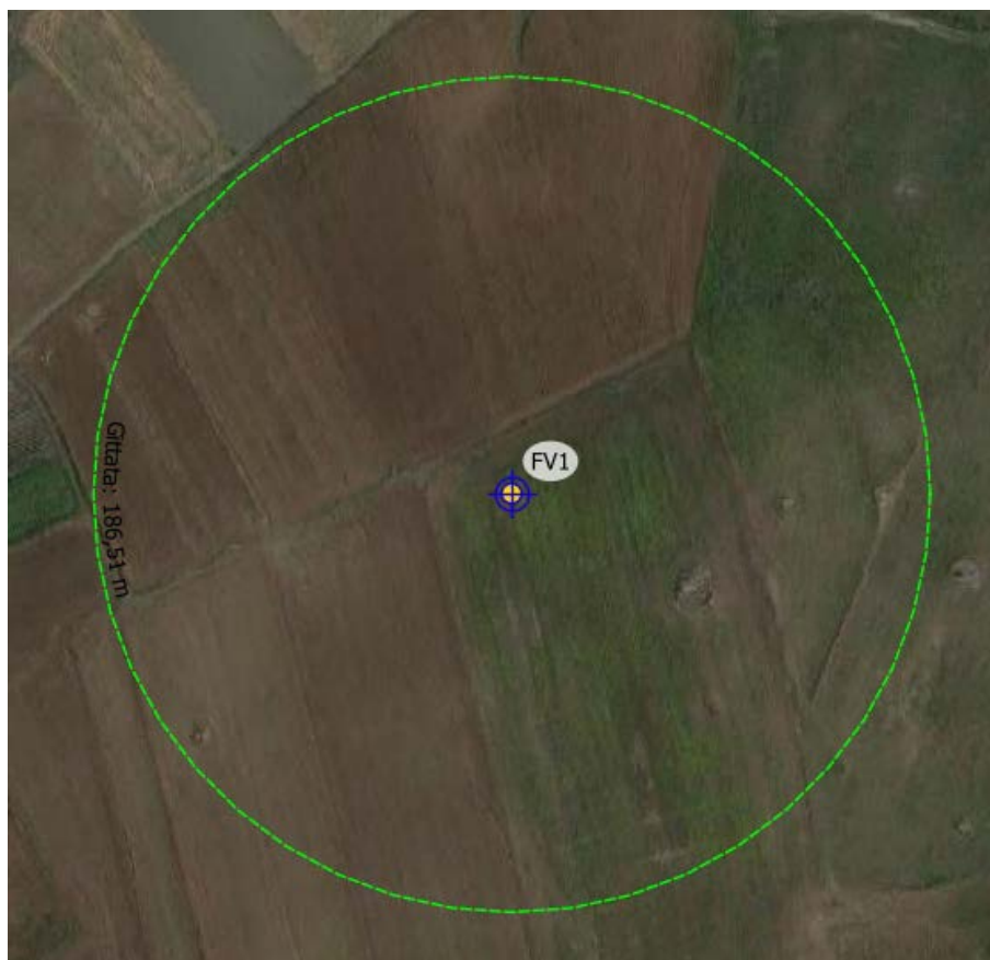
Figura 7-1 – Analisi degli effetti della rottura degli organi rotanti, aerogeneratore FV1
