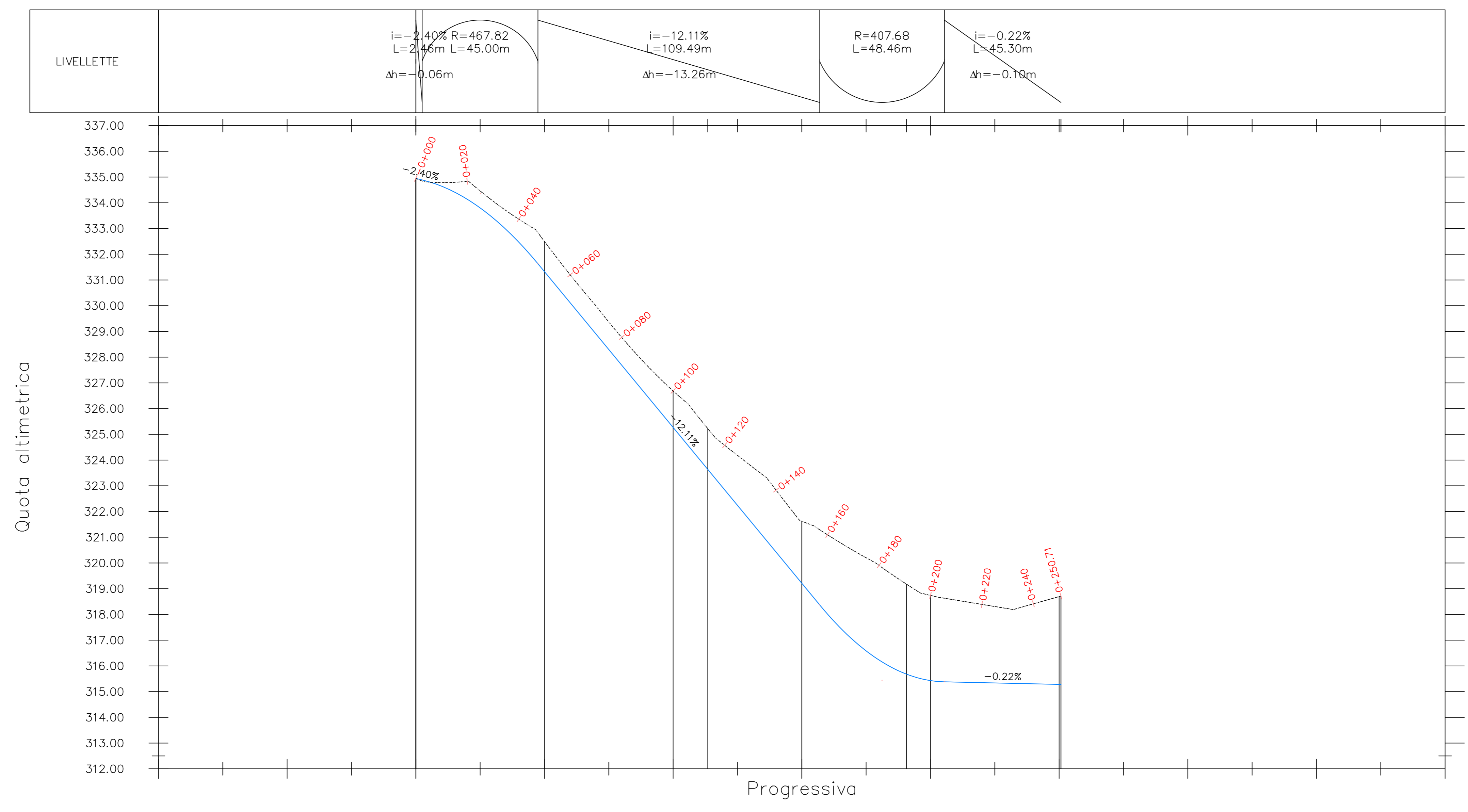
Vista profilo Strada FV2
