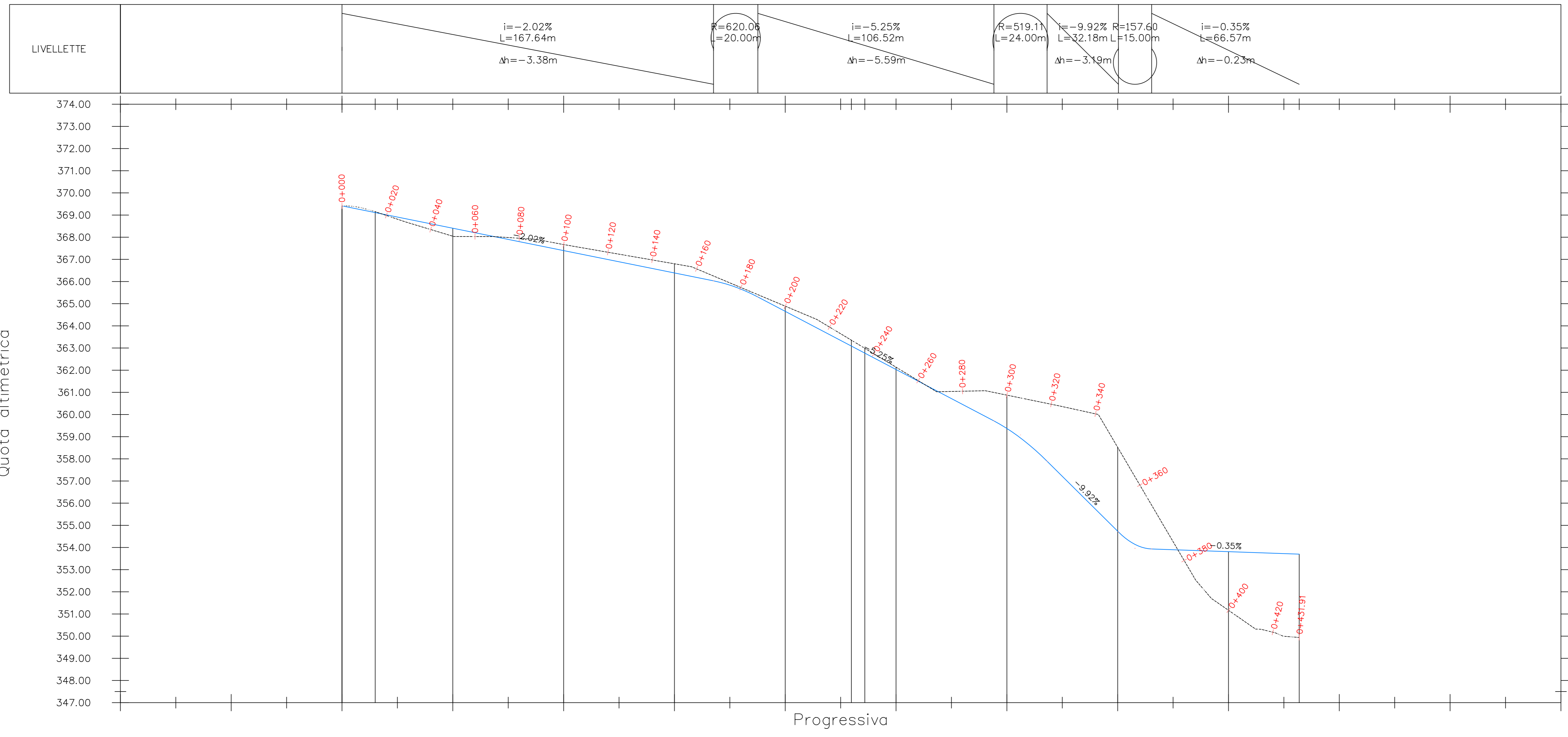
Vista profilo Strada FV3
