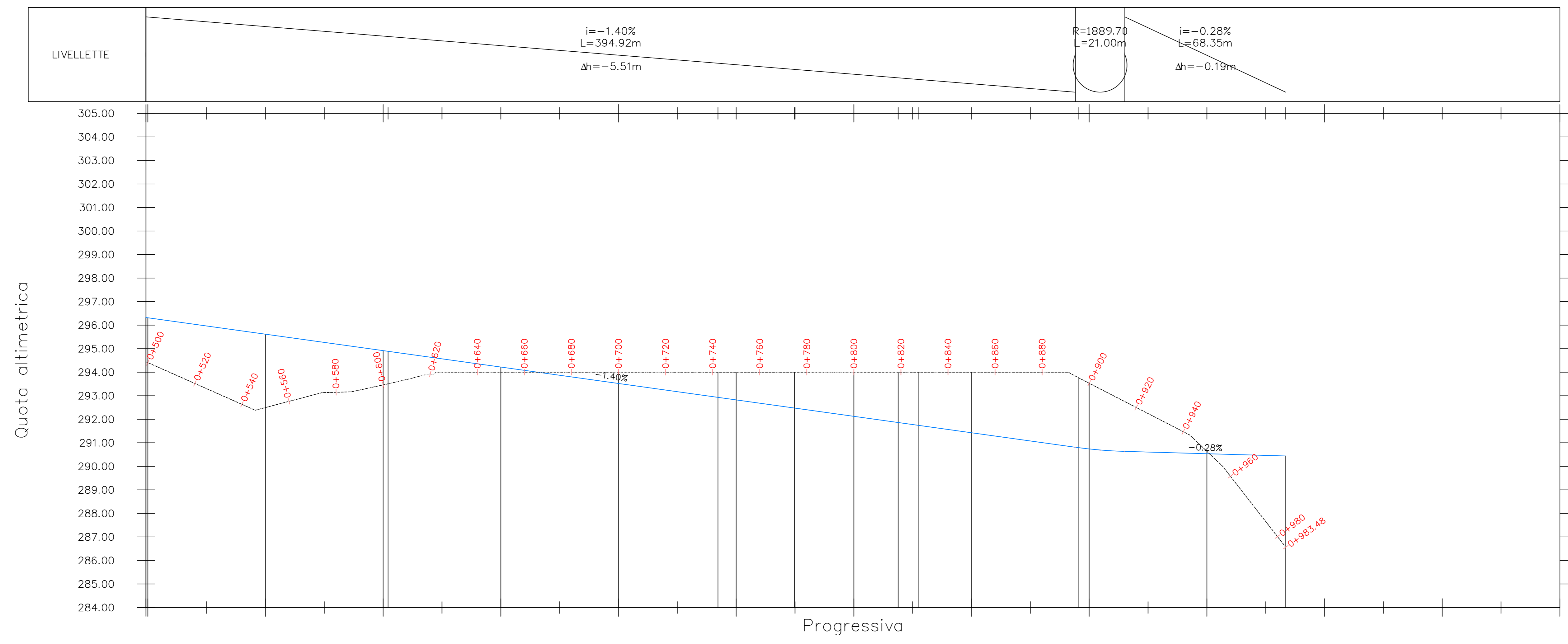
Vista profilo Strada FV8
