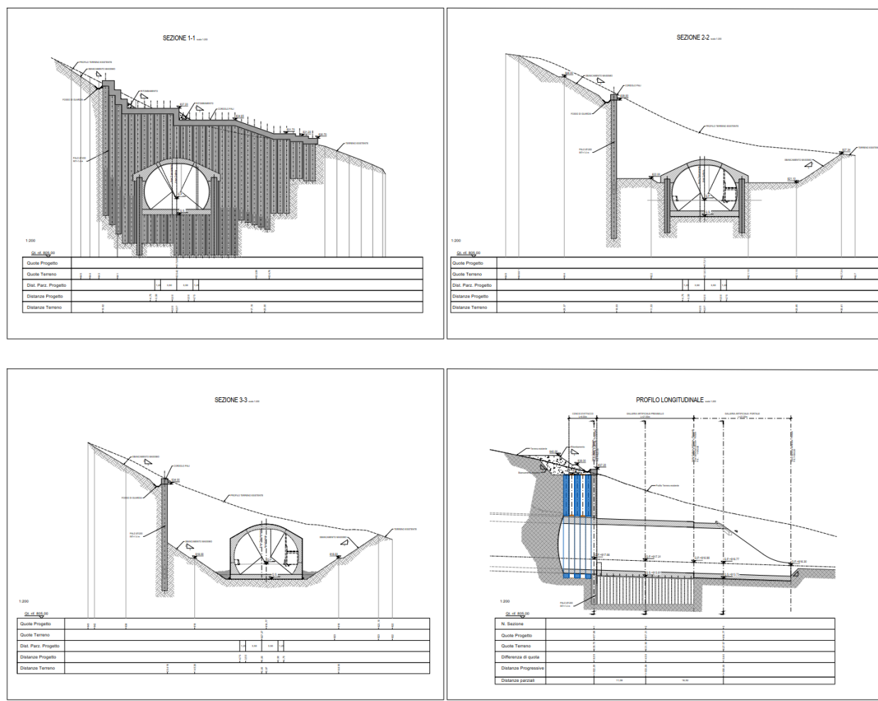
Figura 12 - Imbocco Est: sezioni e profili Progetto Esecutivo
