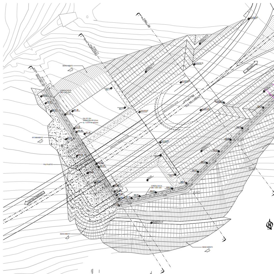
Figura 11 - Planimetria imbocco Est Progetto Esecutivo
