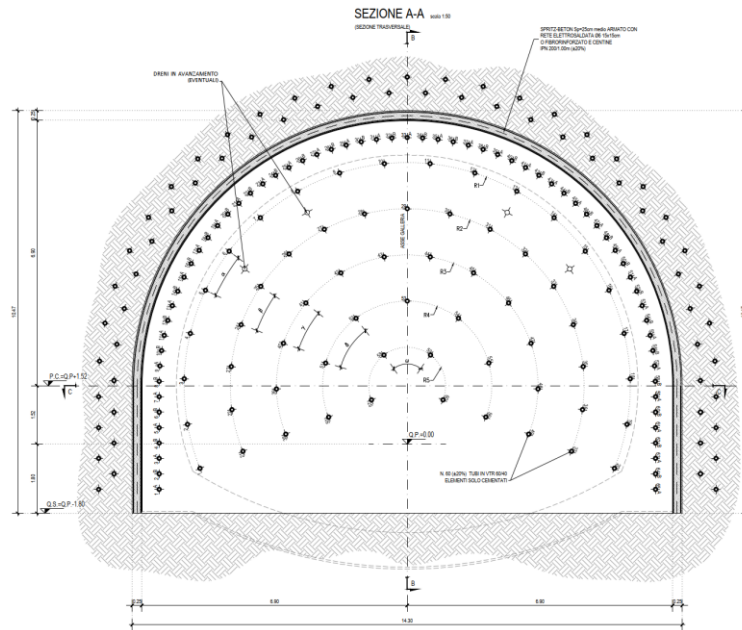
Figura 6 - Sezione tipo C1: scavo e consolidamento tipologico
