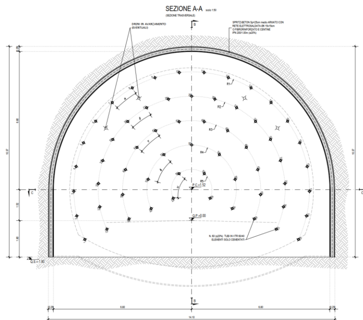
Figura 5 Sezione tipo B1: scavo e consolidamento tipologico
