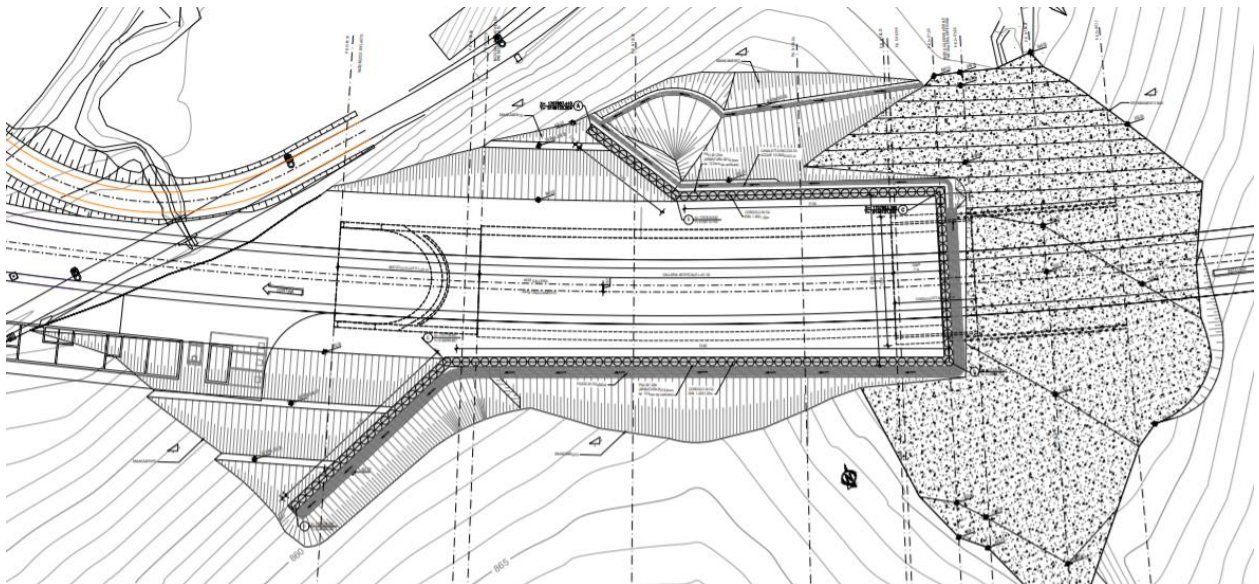
Figura 15 - Planimetria imbocco Ovest Progetto Esecutivo
