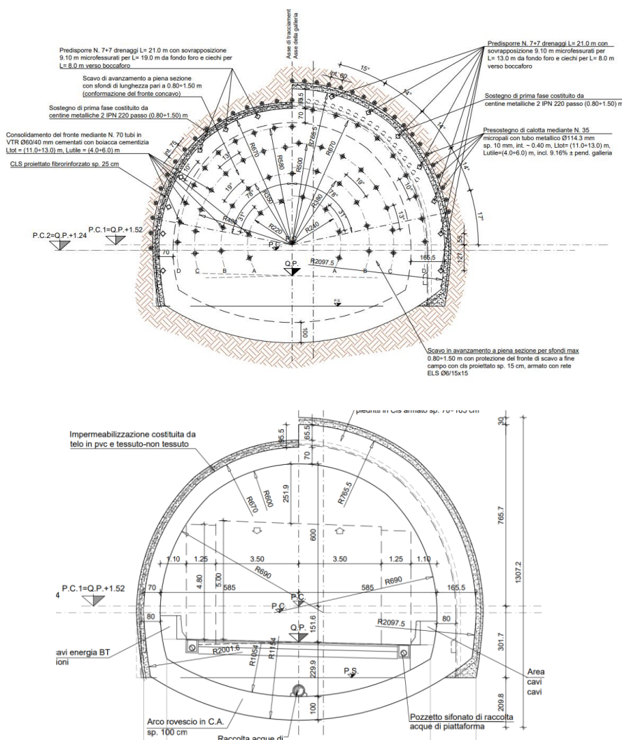
Figura 4- Sezioni tipo da progetto definitivo
