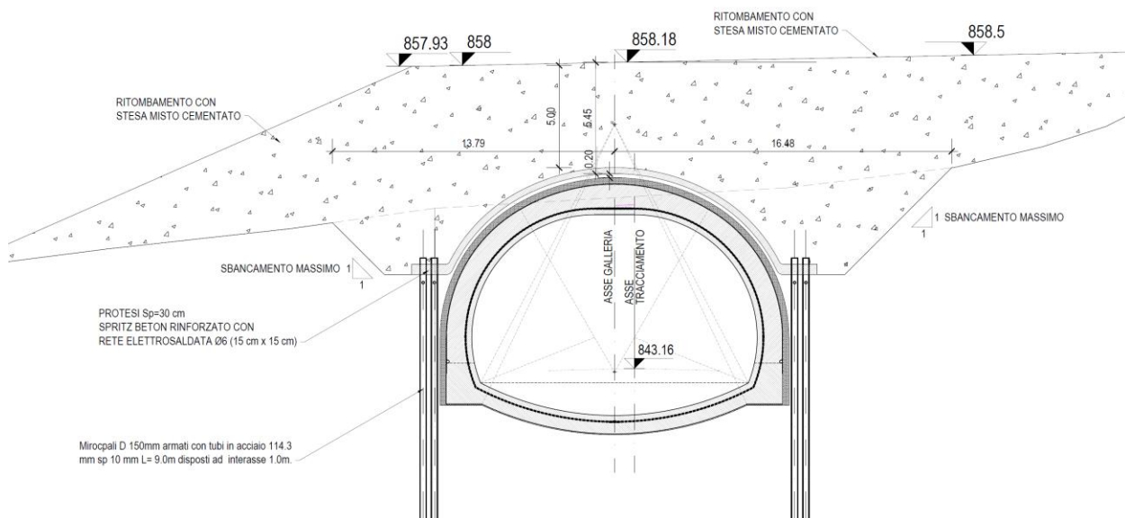
Figura 8 - Sezione tipo Protesi: scavo e realizzazione protesi
