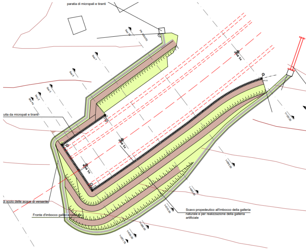
Figura 9 - Planimetria imbocco Est Progetto Definitivo
