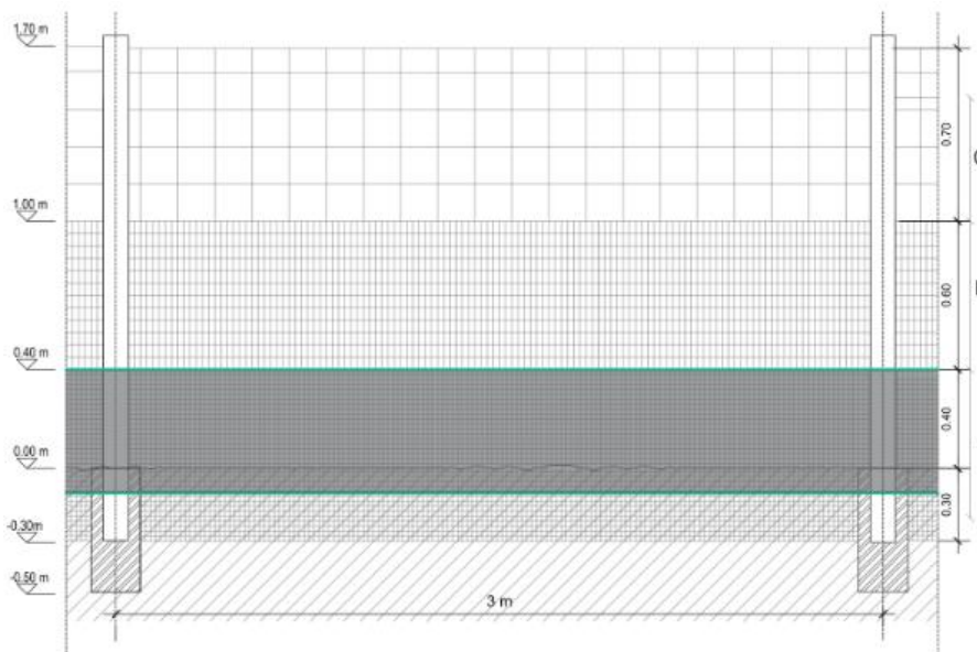
Figura 38 - Rete anti-attraversamento faunistico
