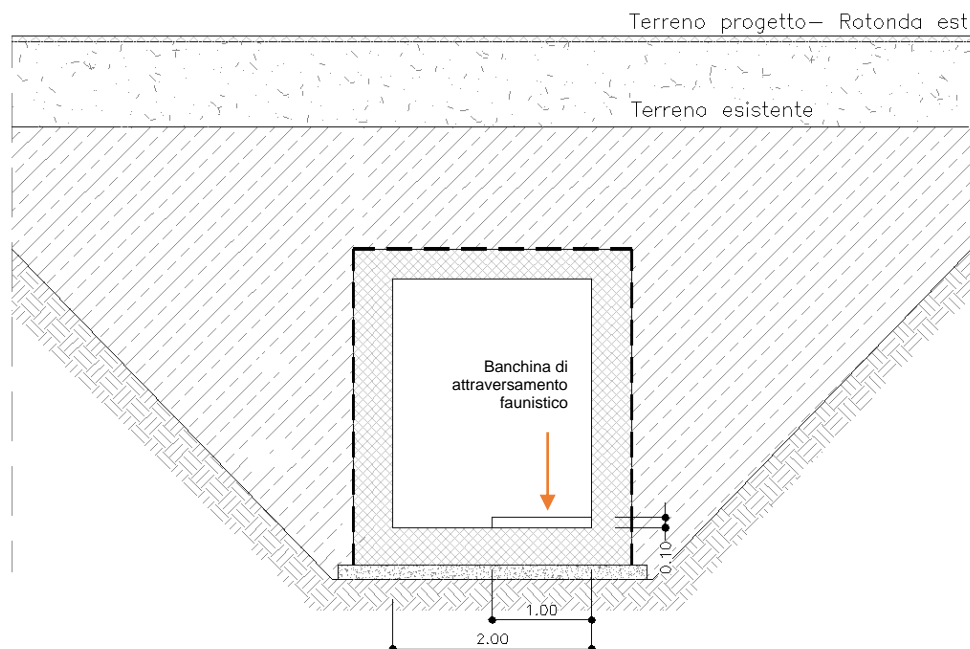
Figura 36 - Sezione scatolare con attraversamento faunistico
