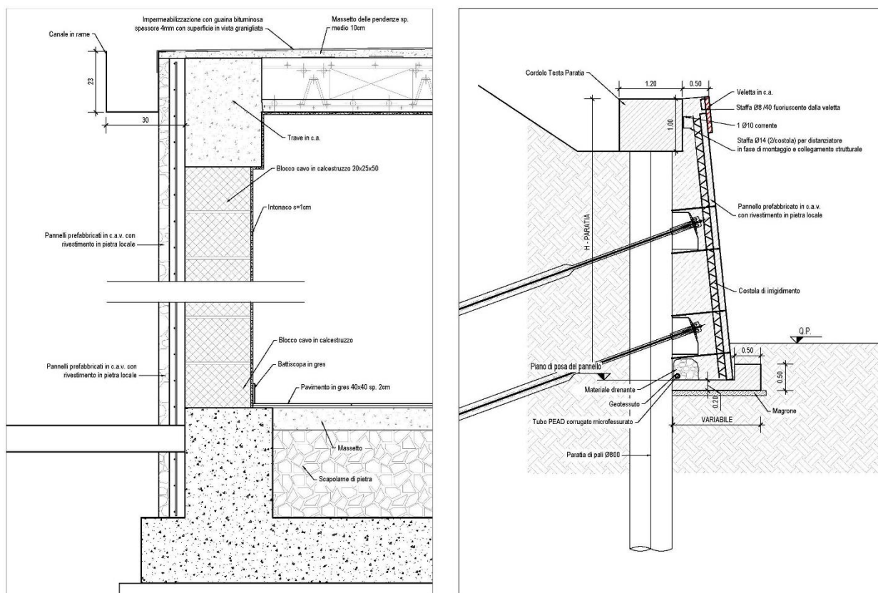
Figura 37 - Dettagli rivestimento da sinistra: fabbricato tecnologico e opere di sostegno della galleria
