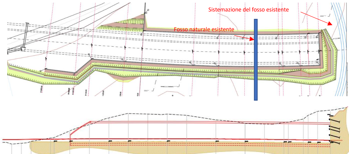
Figura 13 - Planimetria imbocco Ovest Progetto Definitivo
