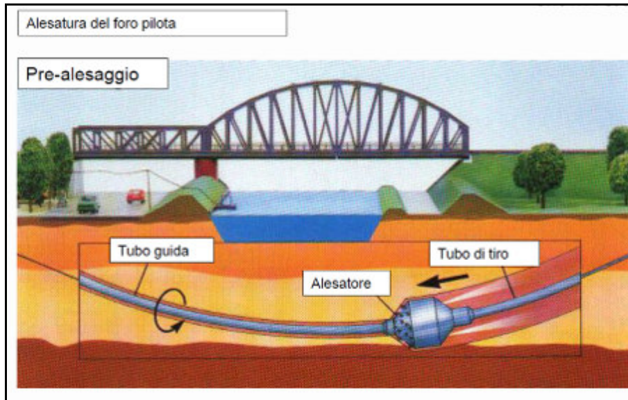
In figura: realizzazione alesatura del foro pilota (immagine reperita dal sito SNAM RETE GAS)
