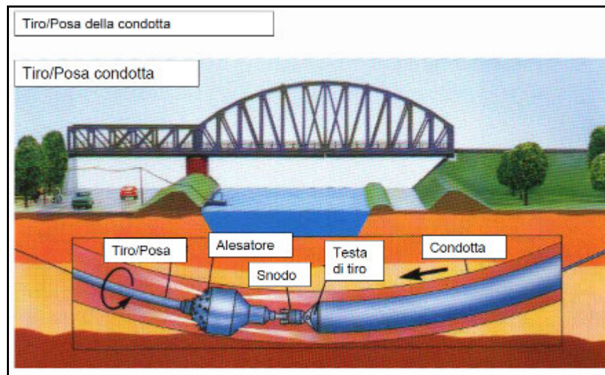
In figura: realizzazione tiro/posa della condotta (immagine reperita dal sito SNAM RETE GAS)
