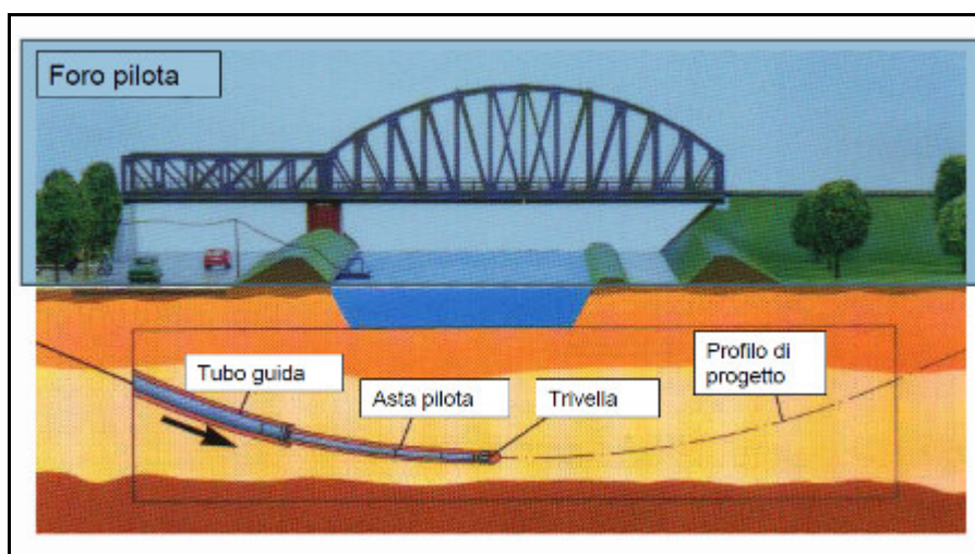
In figura: realizzazione foro pilota (immagine reperita dal sito SNAM RETE GAS)
