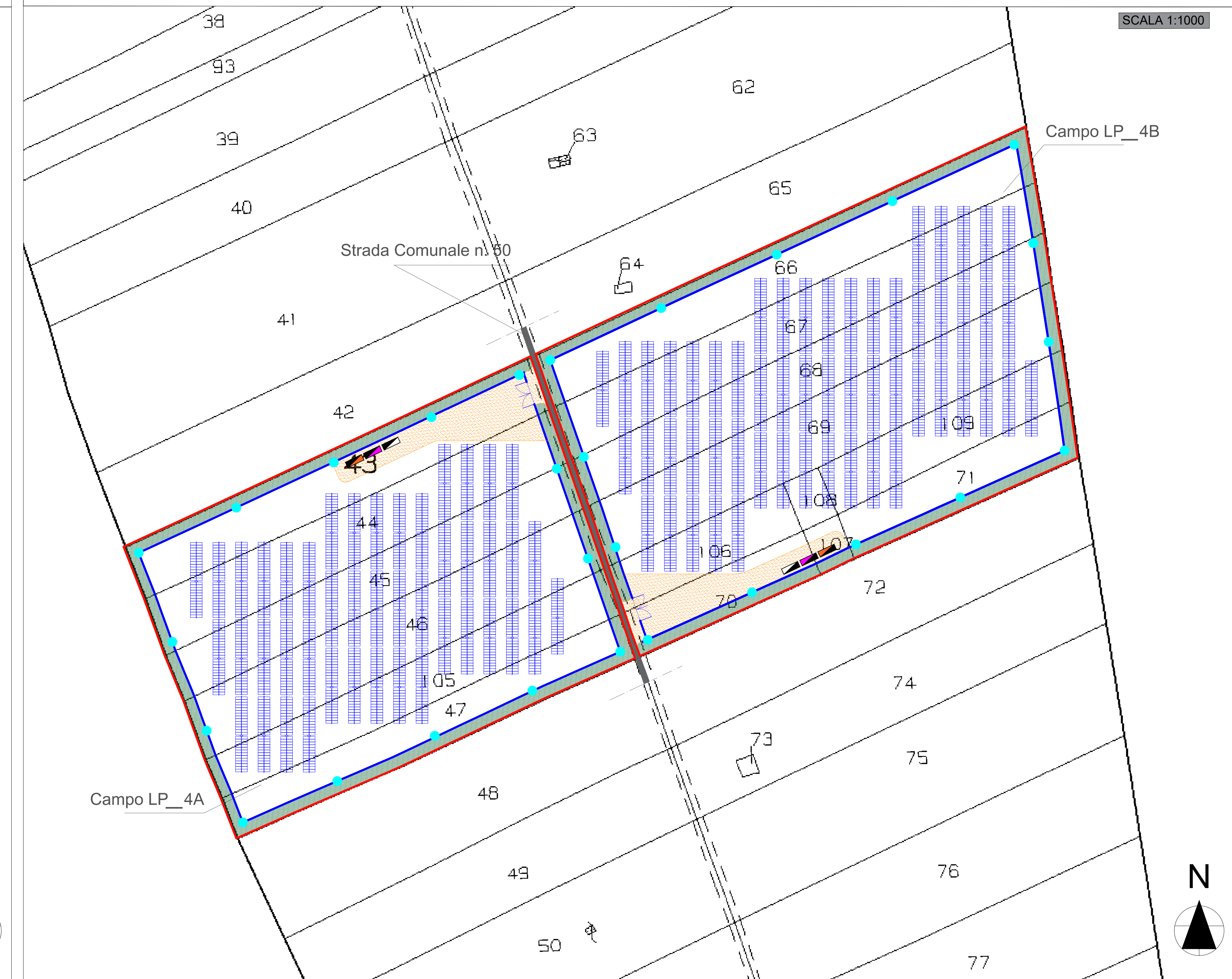
Planimetria Catastale area LP_4 (Fg. 122 Comune di Brindisi) - Stato di Progetto
