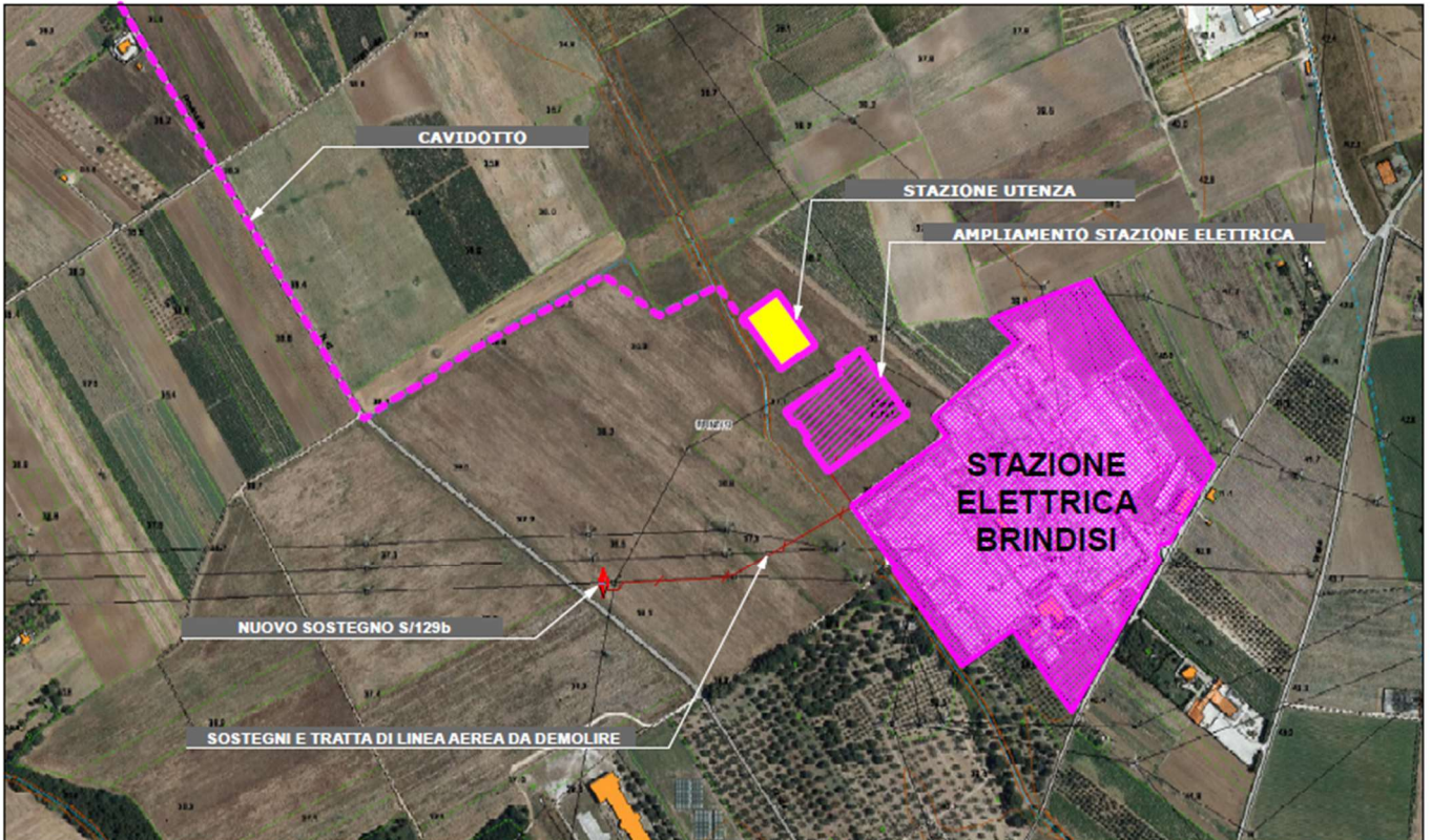
Rappresentazione su ortofoto sezione terminale elettrodotto in MT
