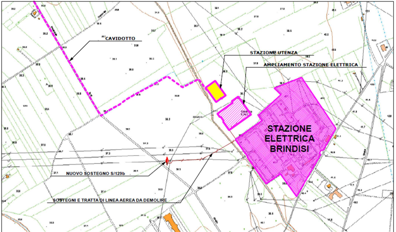
Rappresentazione su CTR sezione terminale elettrodotto in MT con immissione in Stazione di Utenza
