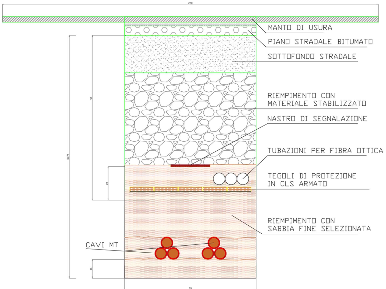
Fig. 15c: Particolare della posa elettrodotto interrato su strada asfaltata pubblica
