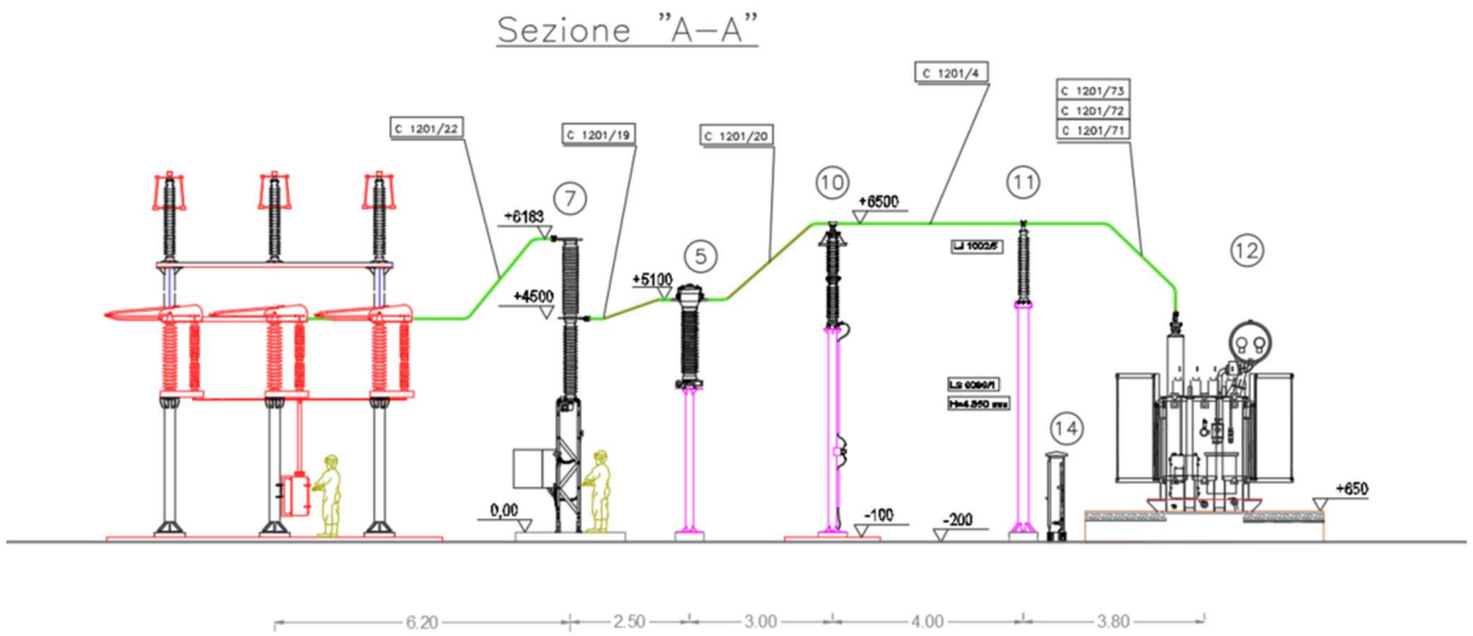
Sezione longitudinale dello Stallo Trasformatore in Stazione di Utanza
