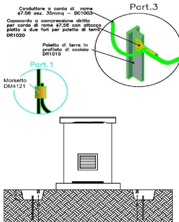
Particolari dell'impianto di terra: da interfacciare all'impianto di terra della CP
