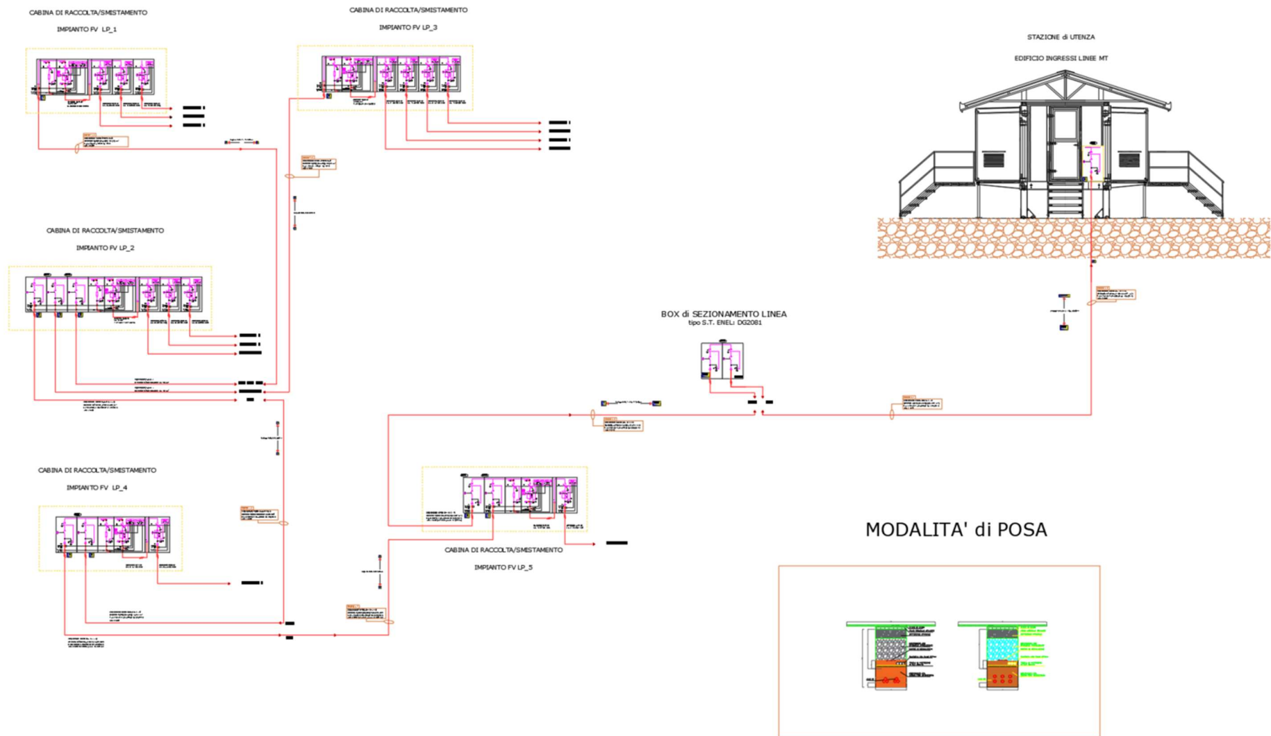
Schema a blocchi della raccolta e vettoriamento energia dai campi fotovoltaici alla S.U. condivisa
