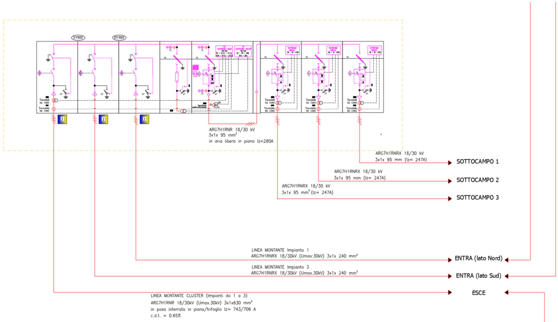
Esempio di schema elettrico per allestimento e collegamento tipico di “Cabina di raccolta/vettoriamento” verso RTN (rif. Norme CEI 0-16)
