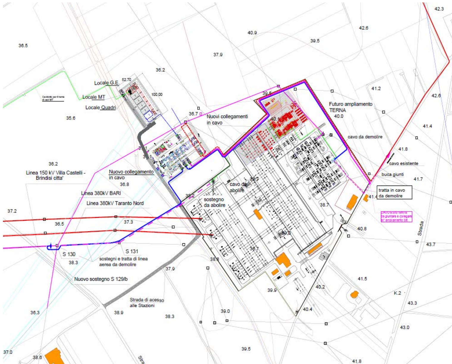
Corografia : Rappresentazione della SE esistente 380/150 kV “Brindisi Pignicelle” e le Opere di Rete da realizzare
