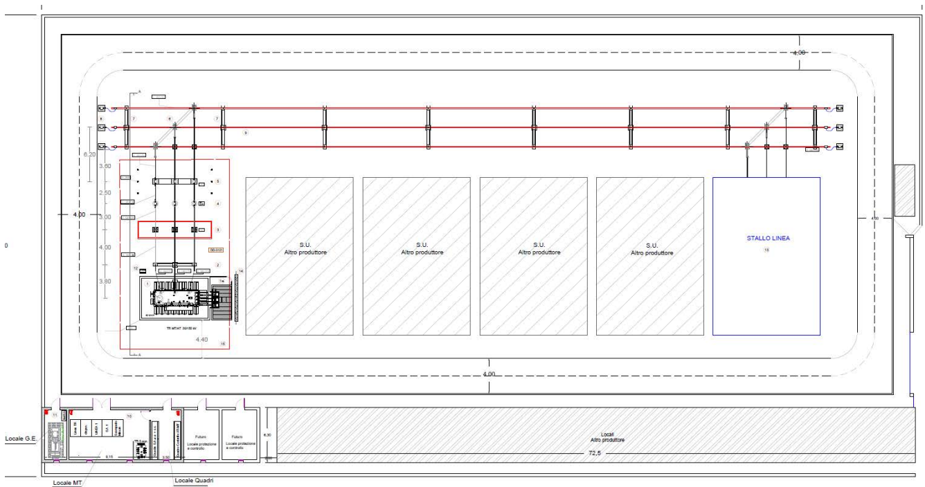
Pianta elettromeccanica della Stazione di Utenza condivisa (rilievo della sezione di pertinenza, Sbarre Parallelo e Stallo Linea RTN)
