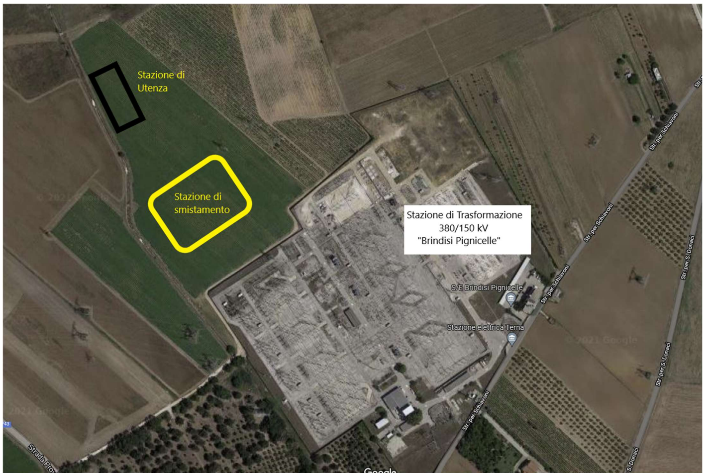
Rappresentazione della S.E. 380/150 kV "Brindisi Pignicelle" ed area delle Stazioni di Smistamento ed Utanza condivisa
