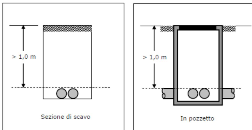
Fig. 16 Profondità minima dei cavidotti
