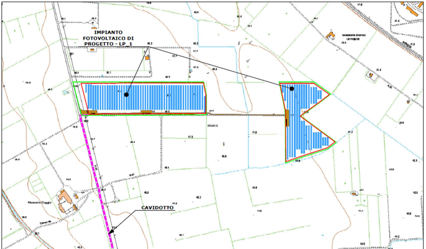
Area 1: unità di produzione energetica da fonte solare - estratto catastale Comune di Brindisi Foglio 40 -
