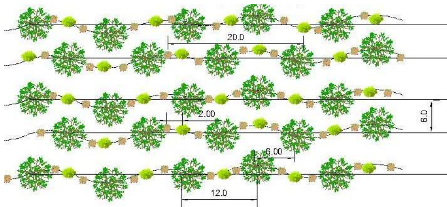
Figura 4: Schema di impianto con andamento a onda
