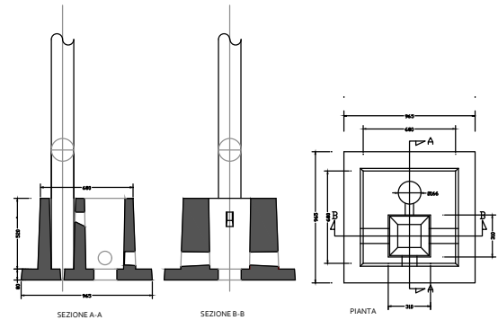
Particolare plinto di fondazione per palo Video-Sorveglianza
