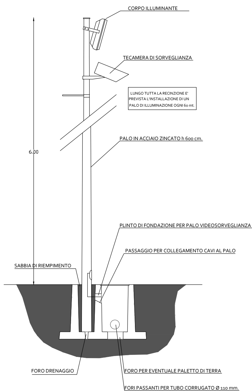
Sezione palo di sorveglianza ed allarme
