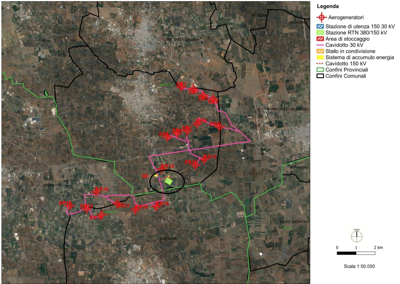
Fig.2: Inquadramento su ortofoto dell'area di impianto
