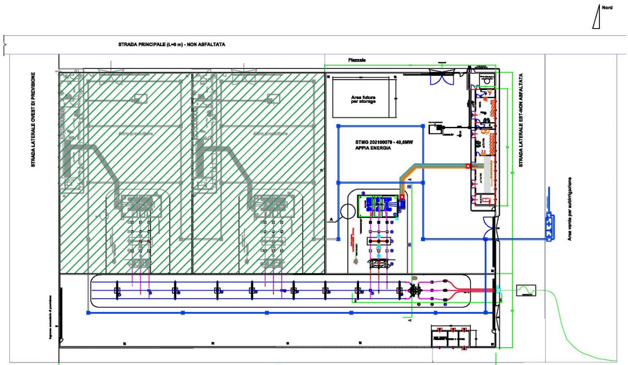
Fig.25 Planimetria SSE con area a sbarre
