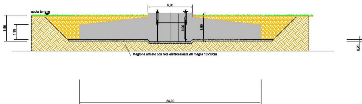
Fig.19 - Tipologia plinto di fondazione
