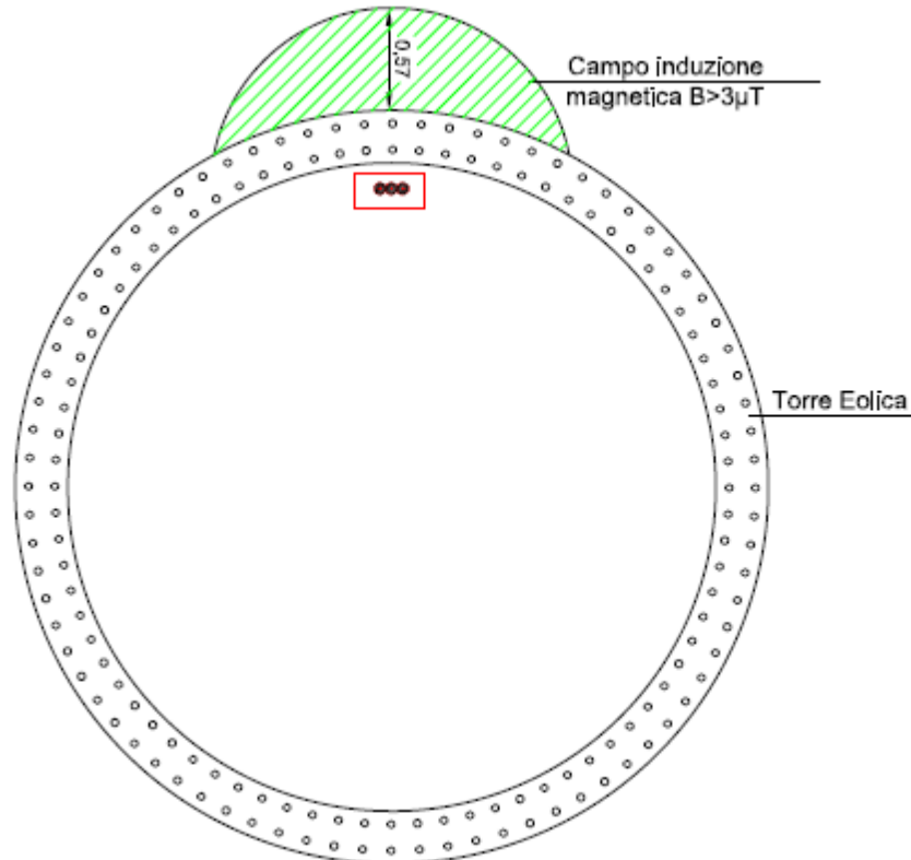
Fig.4 - Valore di induzione magnetica nell'intorno della torre in acciaio
