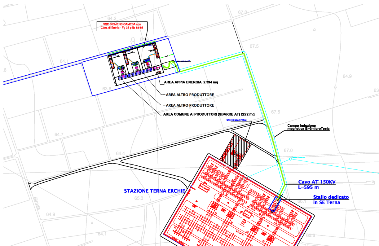
Fig. 8 - DPA nell'intorno del cavo AT 150 kV da SSE utente a SE Terna
