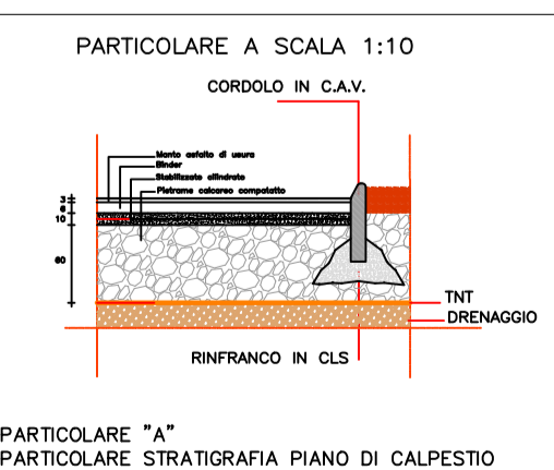
PARTICOLARE "A" PARTICOLARE STRATIGRAFIA PIANO DI CALPESTO
