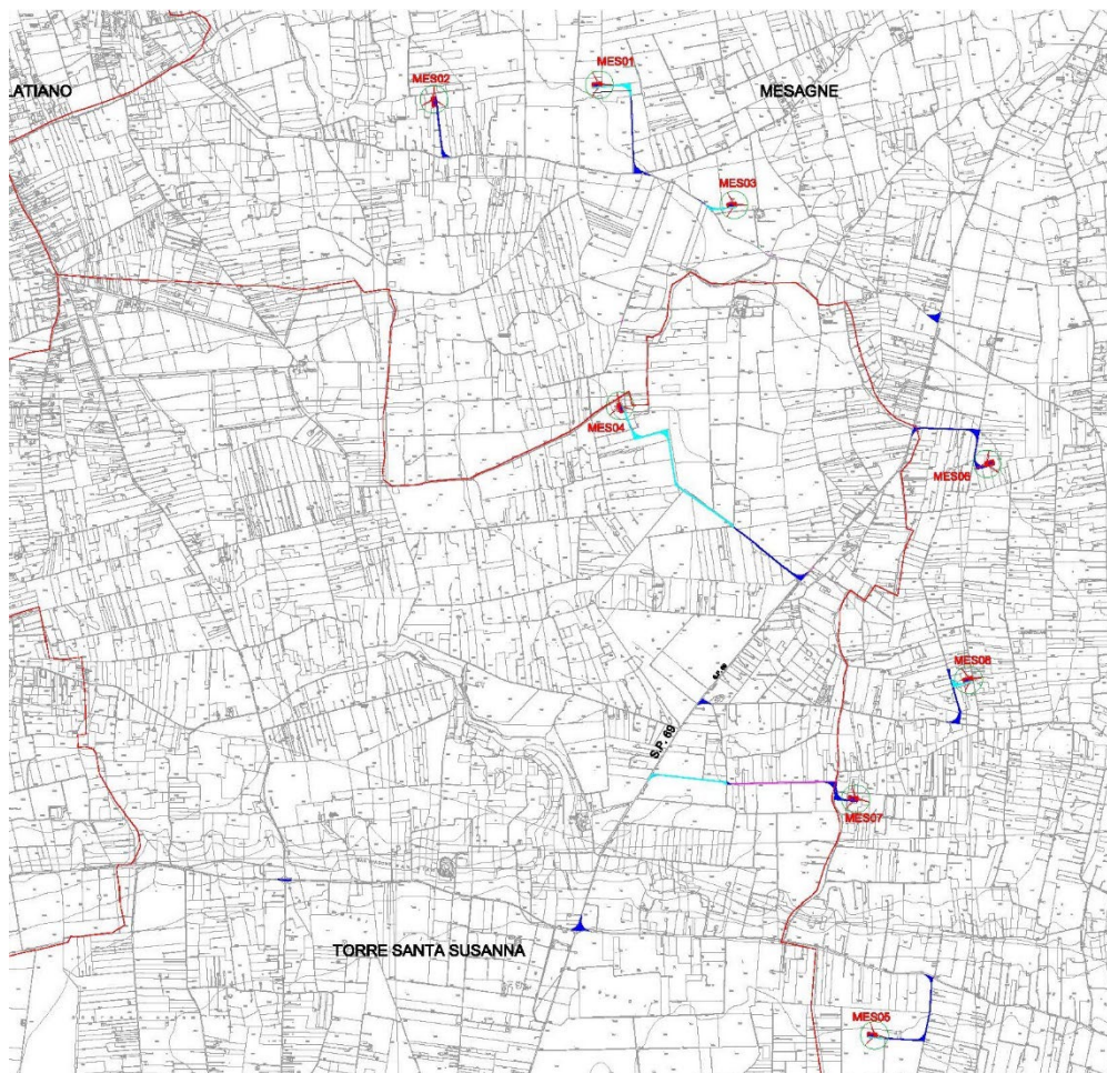
Geometria di impianto – Gli aerogeneratori sono posti su file
