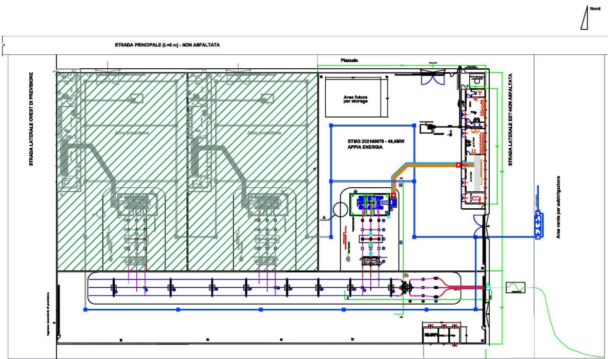
Planimetria SSE APPIA ENERGIA Tratteggiata in verde area destinata ad altri produttori
