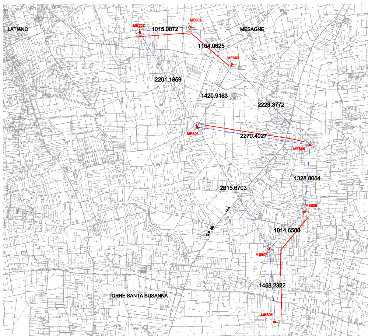
Indicazione della distanza tra aerogeneratori
