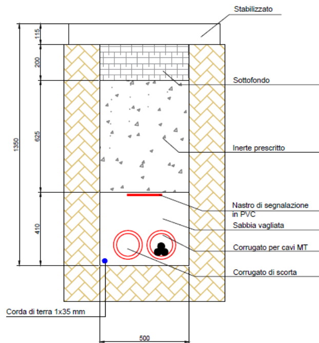
Figura 11: Sezione tipica di posa della linea in cavo
