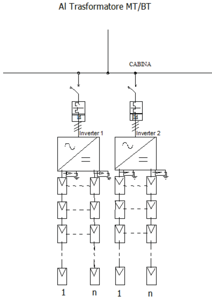
Figura 10: schema unifilare di principio dell'impianto fotovoltaico
