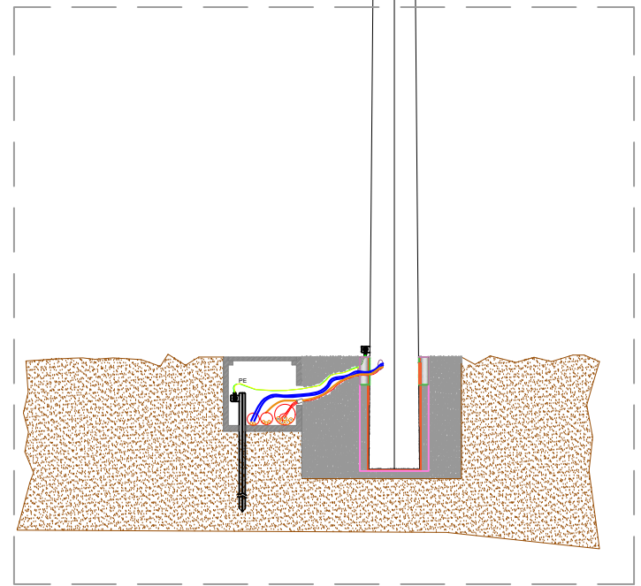
PARTICOLARE B
