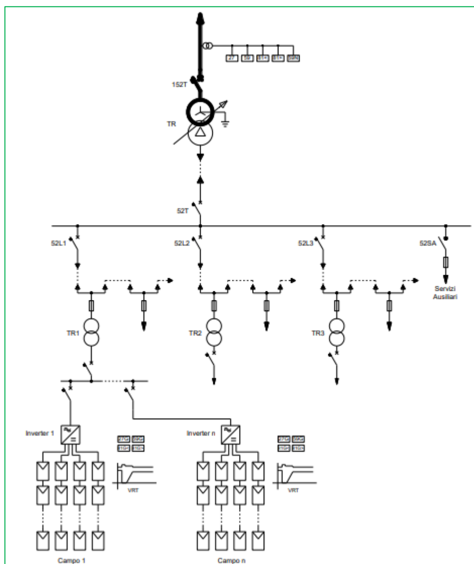
Figura 3- Schema di principio con evidenza delle protezioni di rete
