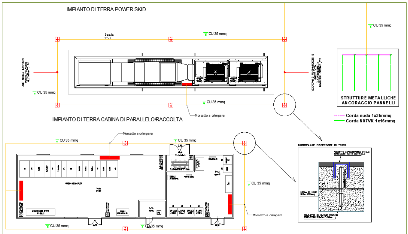
Figura 2-schema di impianto di terra
