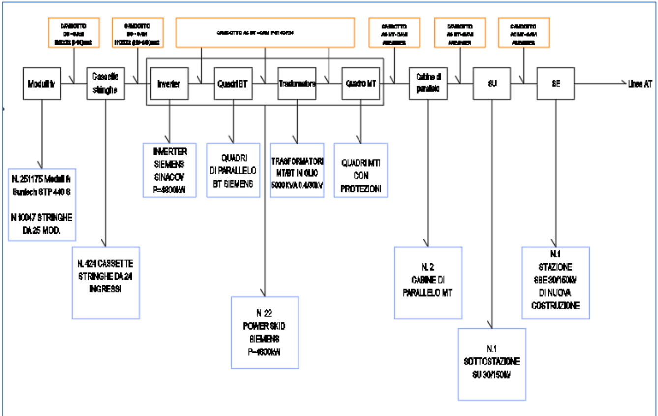
Figura 3 - Schema a blocchi impianto
