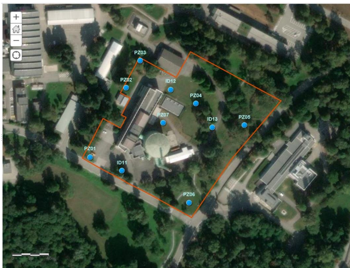
Figura 9–3 - Ubicazione dei punti di monitoraggio per le acque sotterranee
