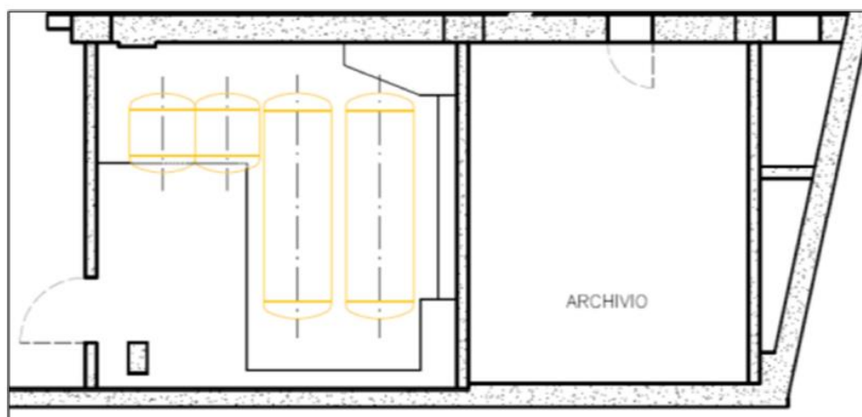
Figura 6–28 Locali interrati 21n (annesso A)
