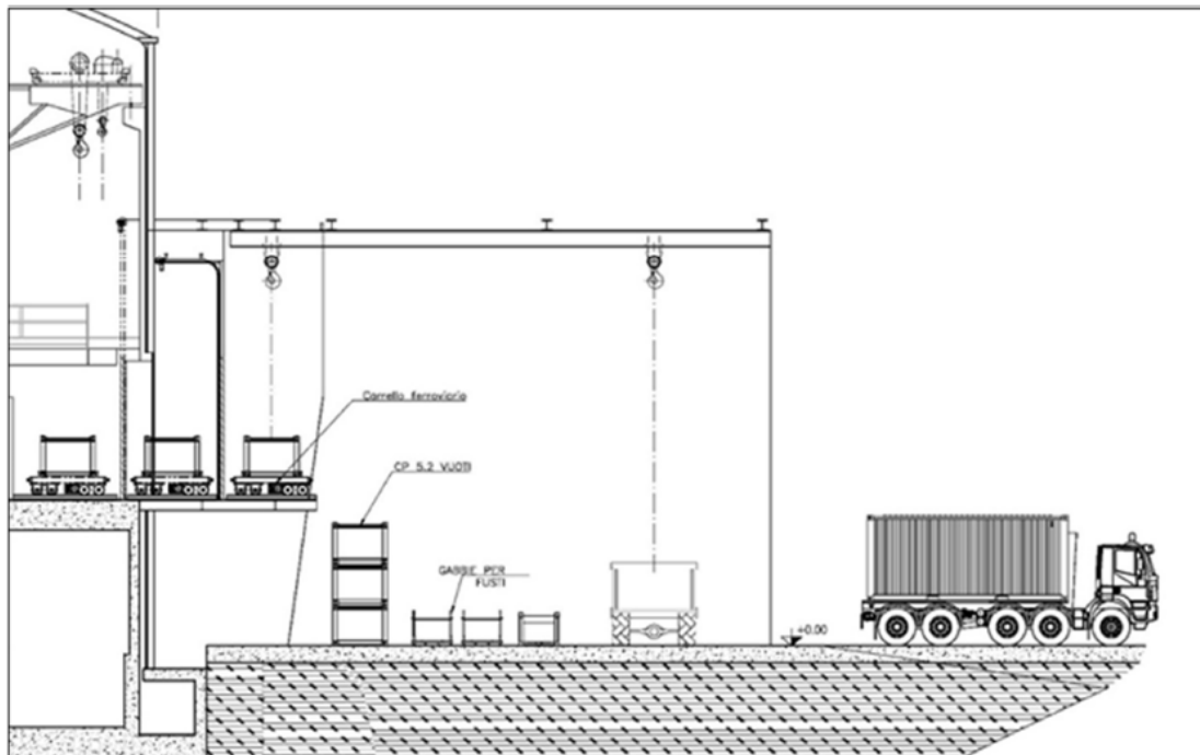
Figura 6-18 Layout sistemazione accesso lato Sud al Contenitore Stagno (vista)
