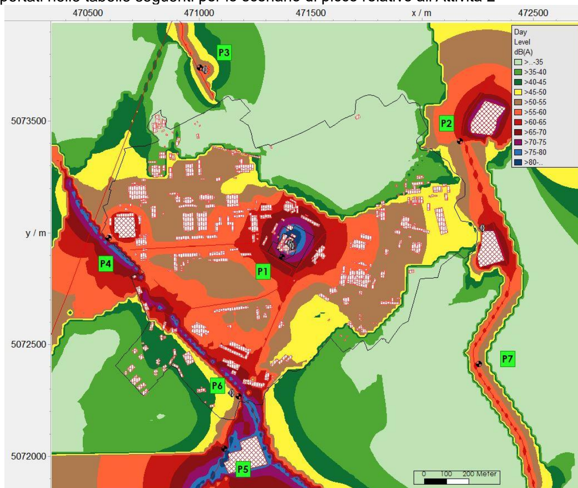
Figura 7-21 Scenario di cantiere – Attività 2 “Predisposizione aree di transito per rifiuti radioattivi – Adeguamento Edificio 21B-21G e deferrizzazione cls”
