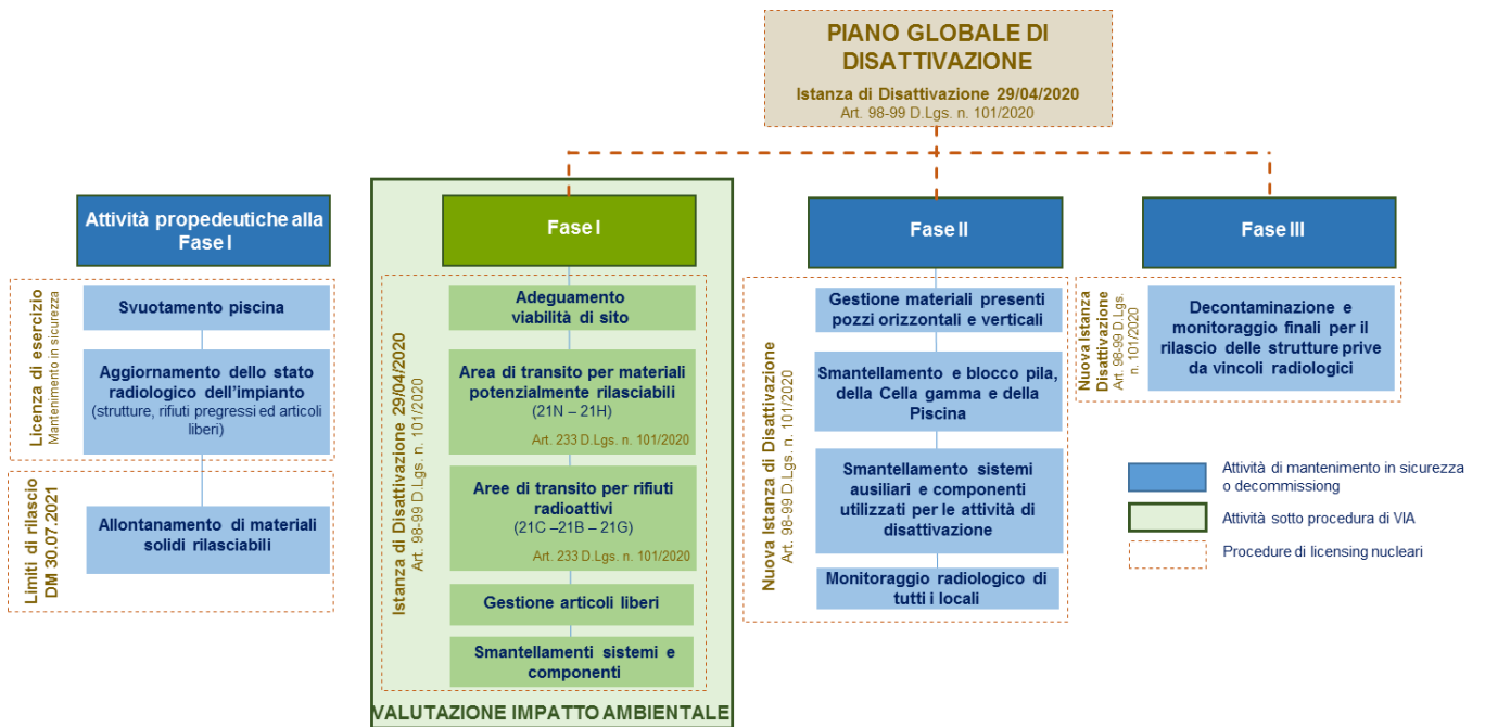
Figura 2–3 Schema delle fasi di decommissioning dell’impianto ISPR1
