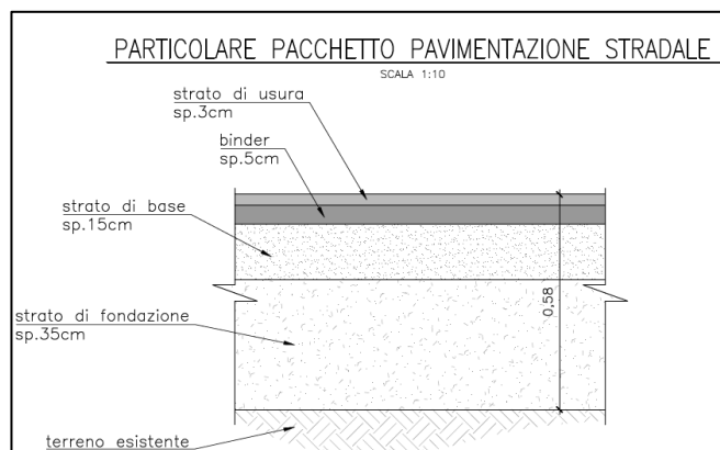
Figura 6–2 Tipologico dei pacchetti stradali
