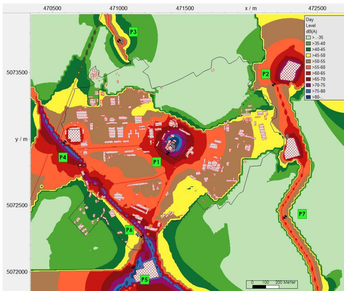
Figura 7-18 Scenario di cantiere – Attività 2 "Predisposizione aree di transito per rifiuti radioattivi – Adeguamento Edificio 21B-21G e deferrizzazione cis"
