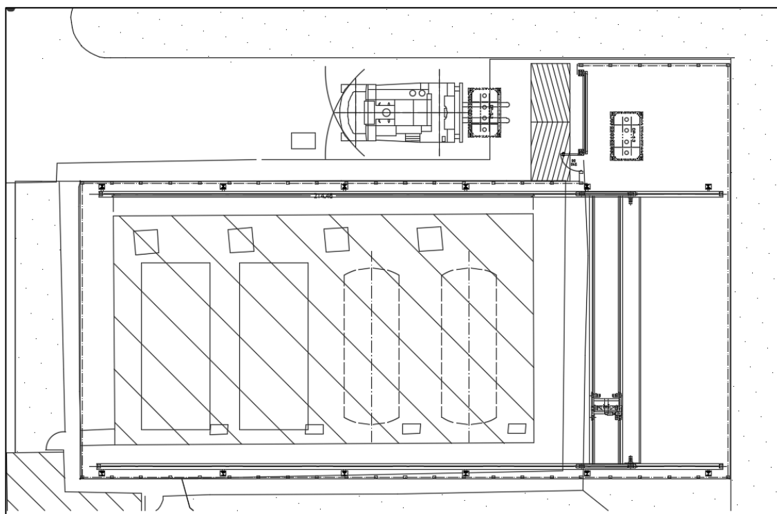
Figura 6–23 Facility di smantellamento edificio 21f – Pianta
