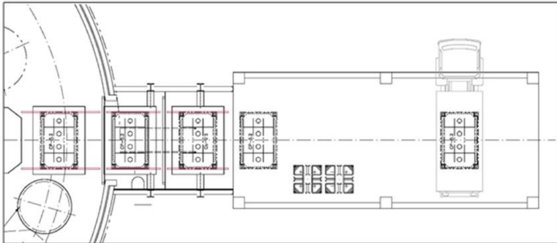
Figura 6-17 Layout sistemazione accesso lato Sud al Contenitore Stagno (pianta)
