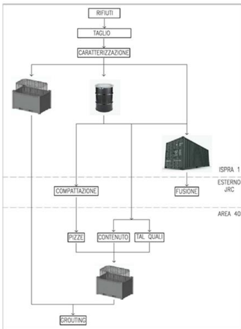
Figura 6–31 Schema di gestione dei rifiuti
