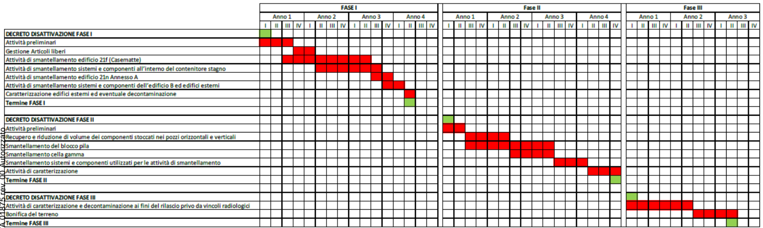
Figura 2–2 Cronoprogramma delle attività di disattivazione dell’impianto Ispra1 (fonte: Piano Globale di Disattivazione)
