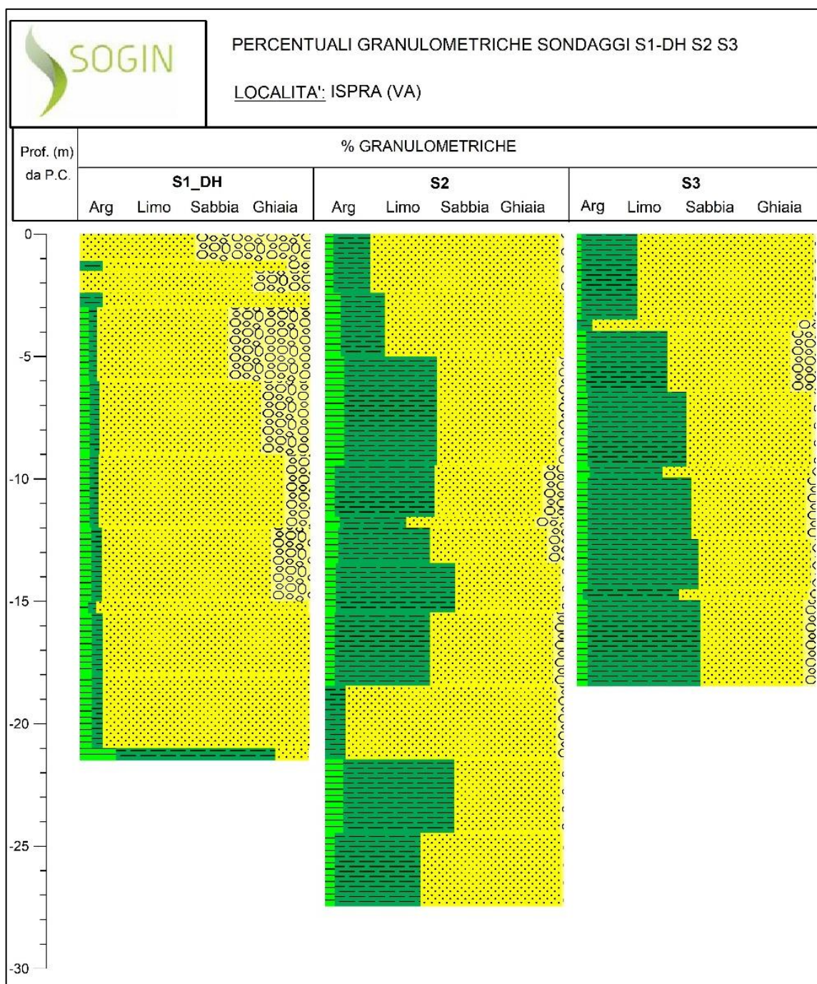
Figura 7-5 Distribuzione granulometrica nei sondaggi S1-DH, S2 e S3 del 2020
