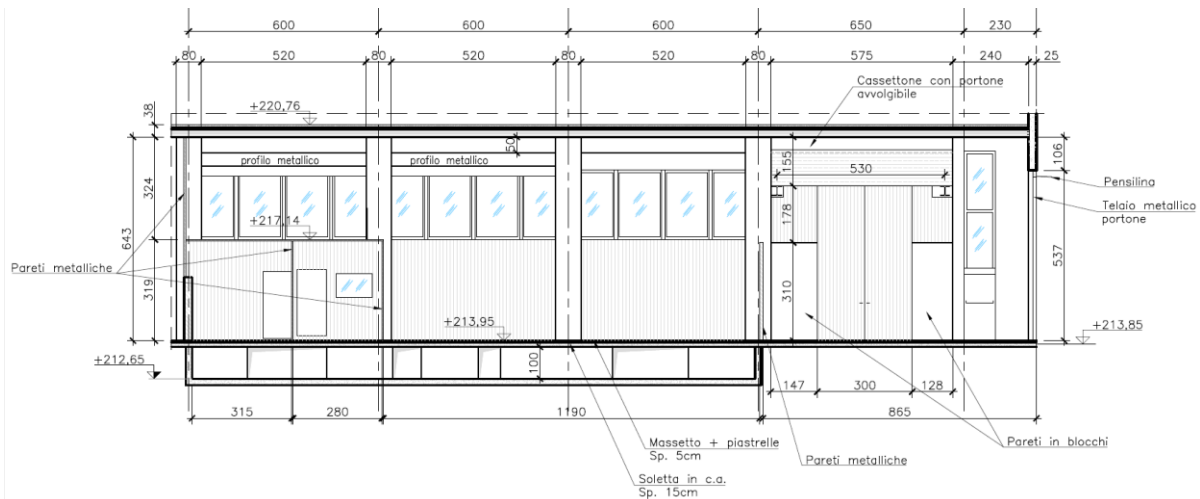
Figura 6-7 Sezione C-C edificio 21n – Ante Operam
