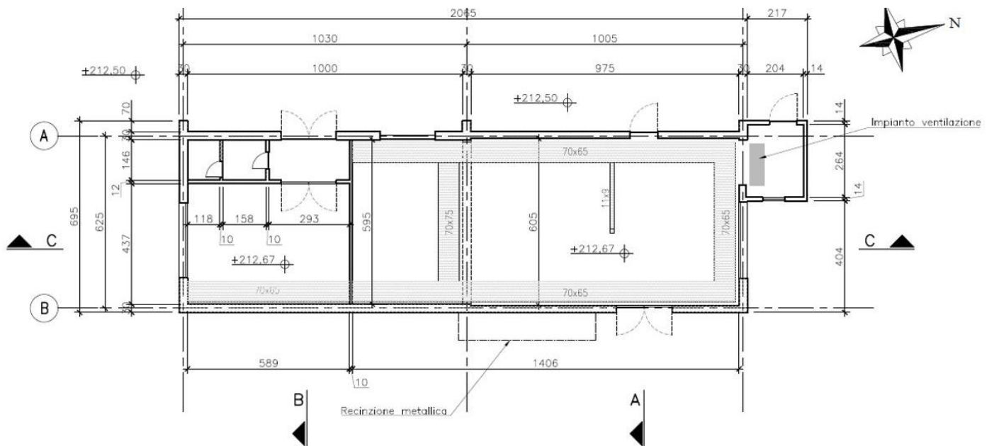
Figura 6–10 Pianta dell'edificio 21h - Ante Operam
