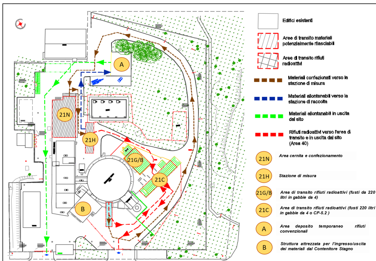
Figura 6-29 Waste route per la gestione dei rifiuti prodotti dagli smantellamenti
