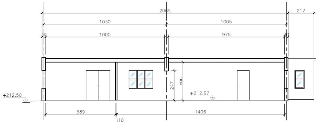
Figura 6–11 Sezione C-C edificio 21h – Ante Operam
