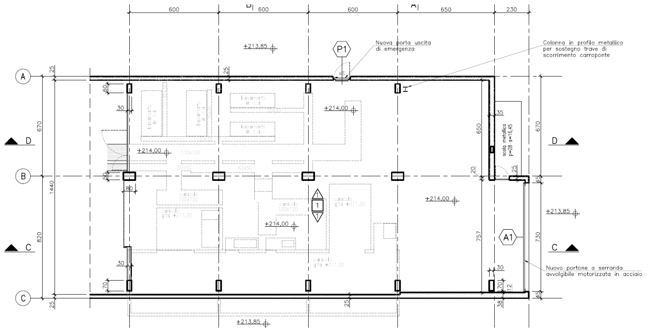
Figura 6-8 Pianta dell'edificio 21n - Post Operam
