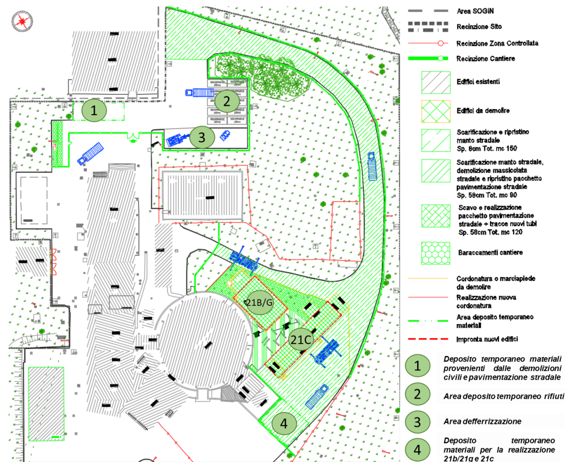
Figura 6-15 Adeguamenti edifici 21b/21g e 21c – Cantierizzazione
