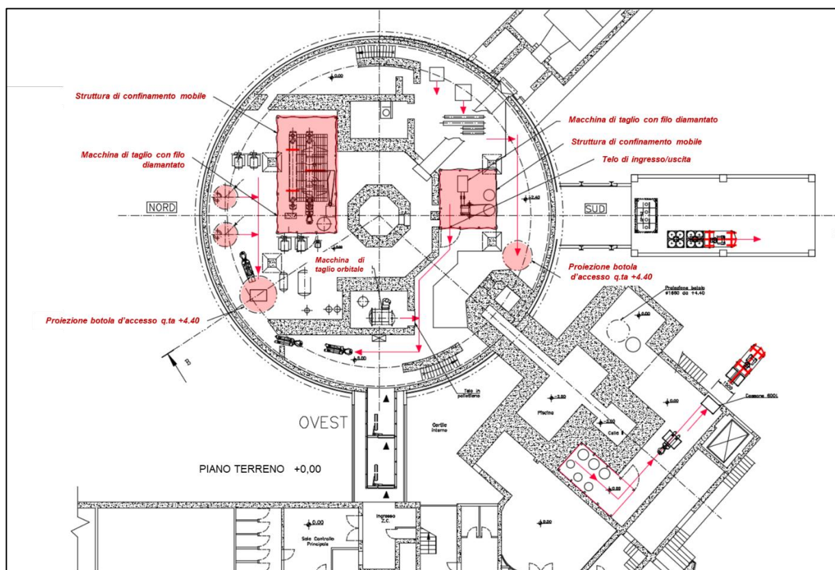
Figura 6–26 Strutture di confinamento mobili a quota +0.00m
