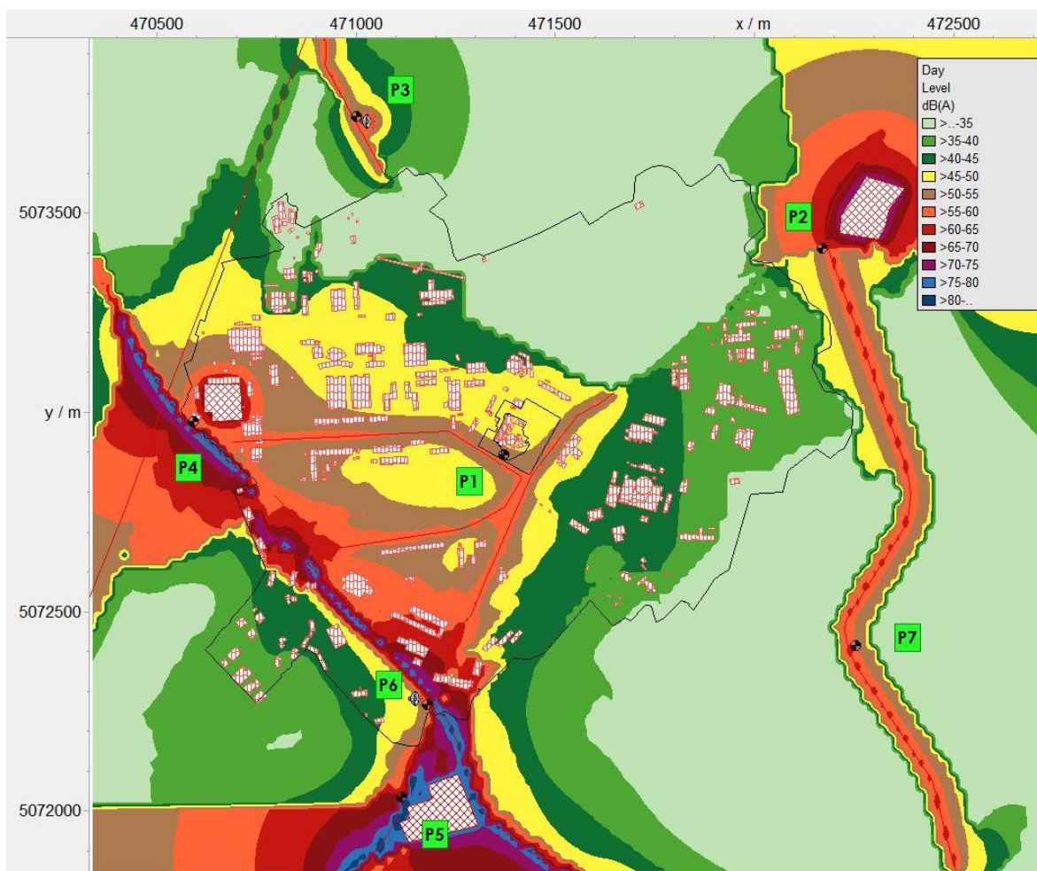
Figura 7-17 Scenario ante operam
