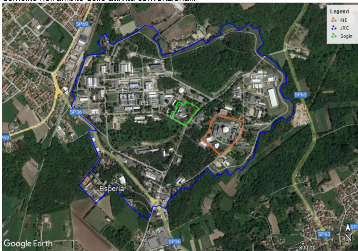
Figura 7–39 Ubicazione del Complesso INE rispetto al sito SOGIN di ISPRA-1
