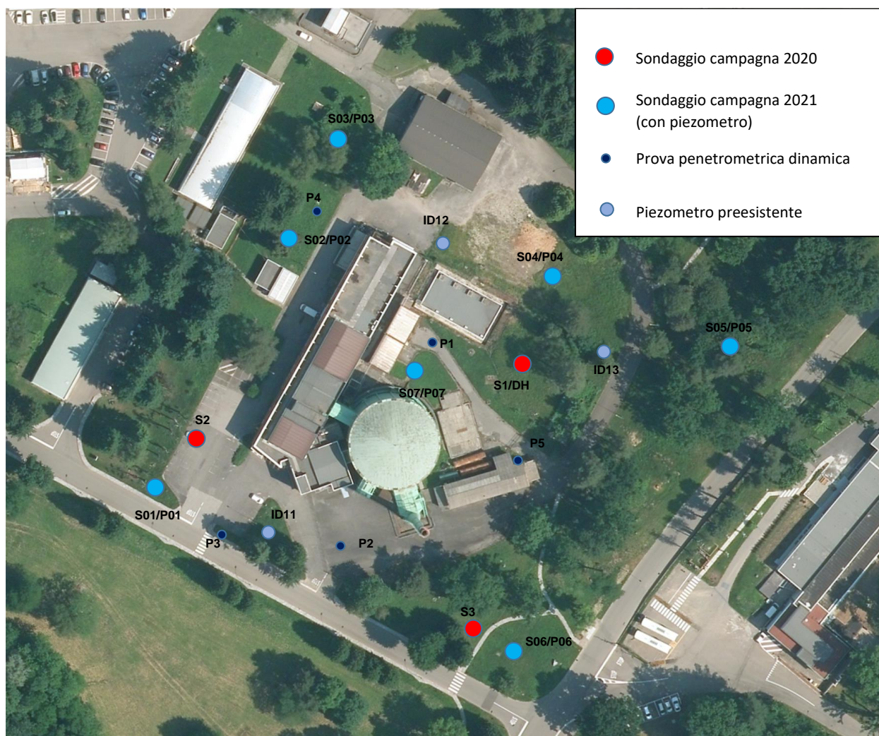
Figura 7-4 Indagini effettuate sul sito
