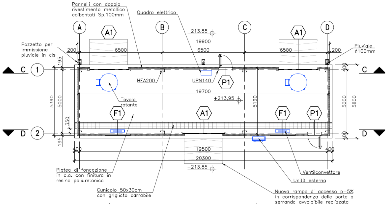
Figura 6–12 Pianta dell'edificio 21h - Post Operam
