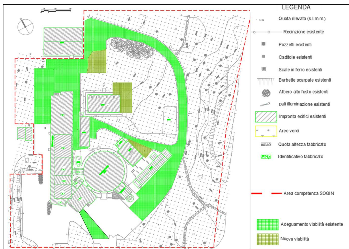
Figura 6-1 rifacimento della viabilità esterna
