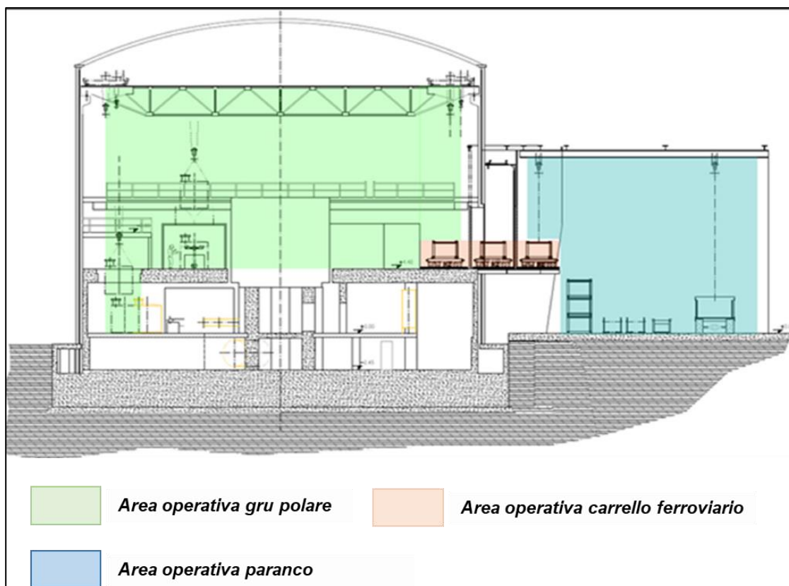
Figura 6–16 Aree operative mezzi di movimentazione per accesso al Contenitore Stagno
