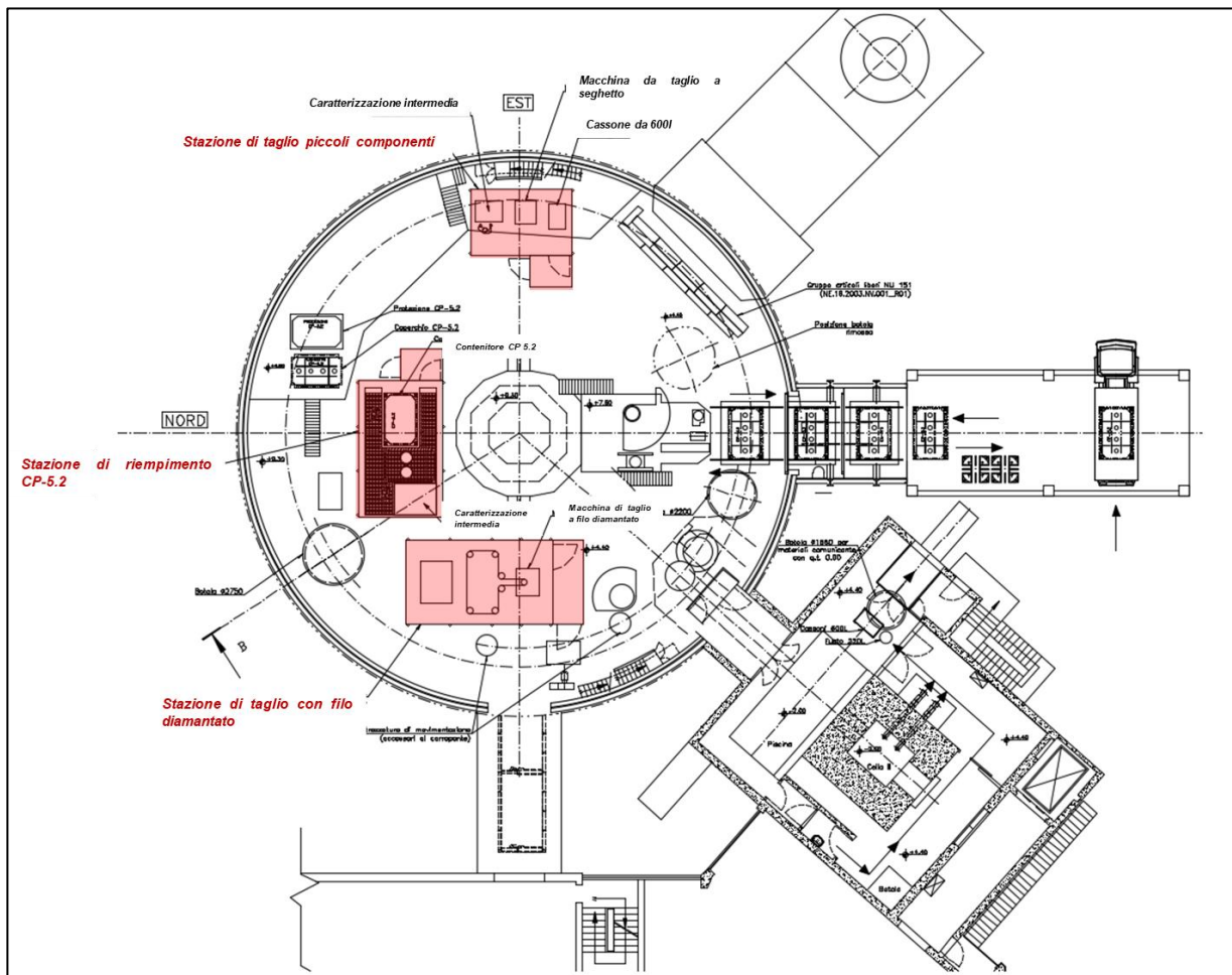
Figura 6–19 Ubicazione delle sezioni di lavoro confinate all'interno del Contenitore Stagno
