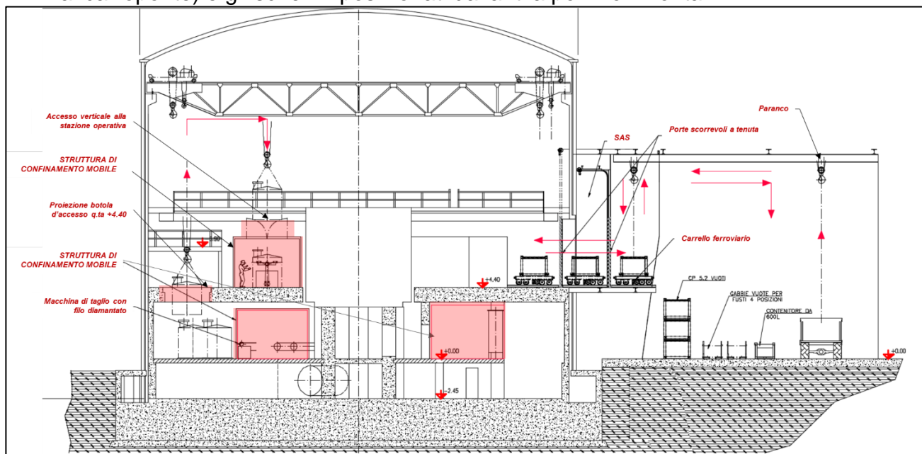
Figura 6-27 Layout smantellamenti interni al Contenitore Stagno
