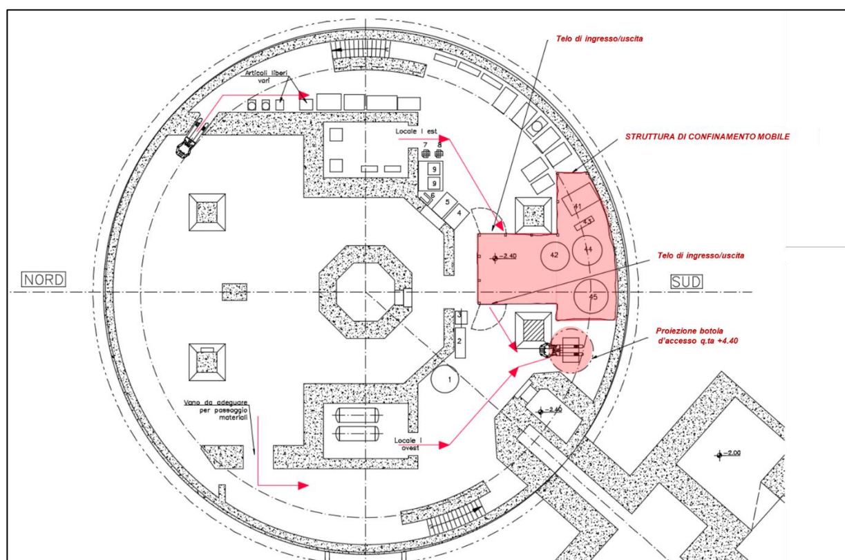
Figura 6–25 Strutture di confinamento mobili a quota -2.50 m
