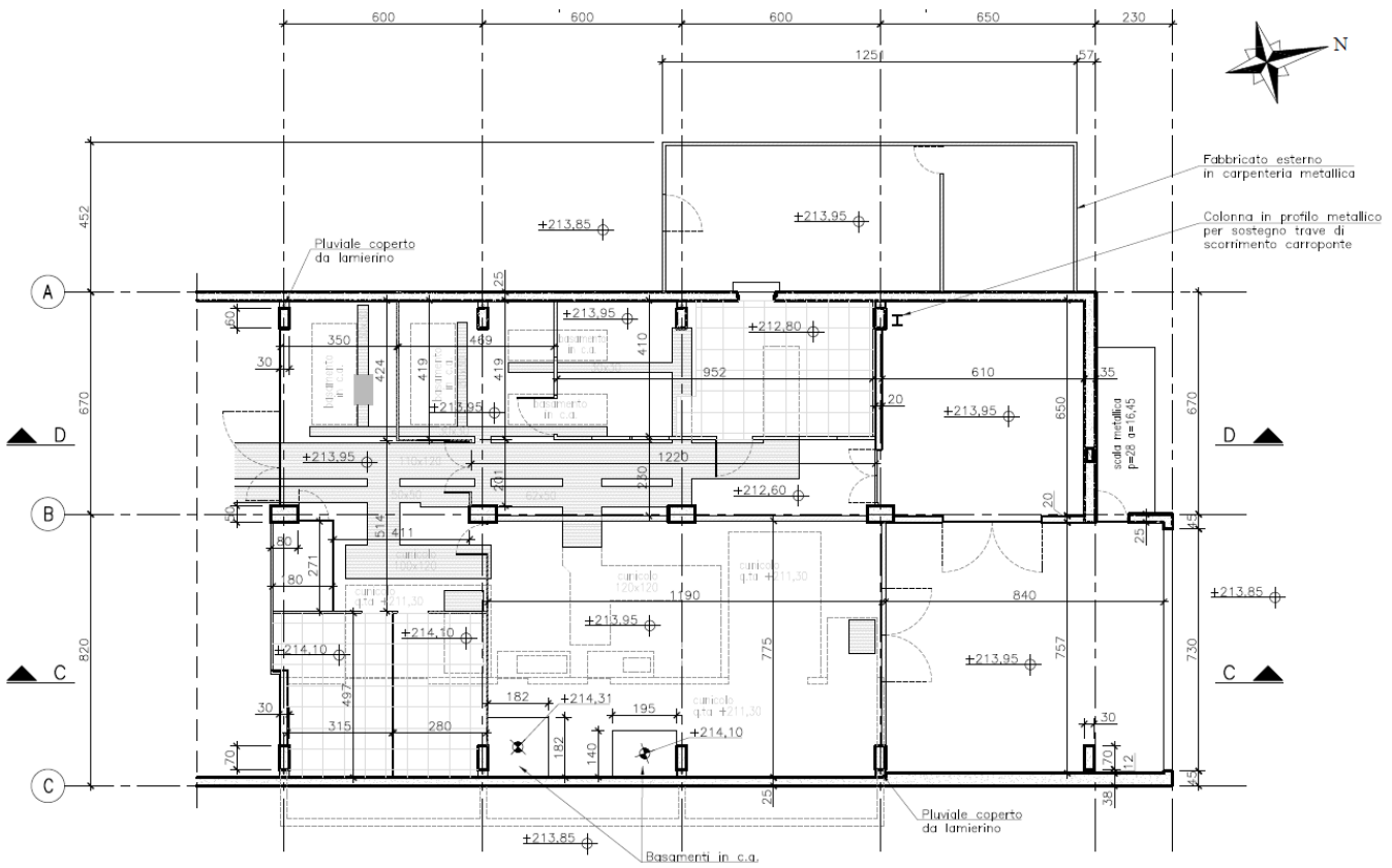
Figura 6-6 Pianta dell'edificio 21n - Ante Operam
