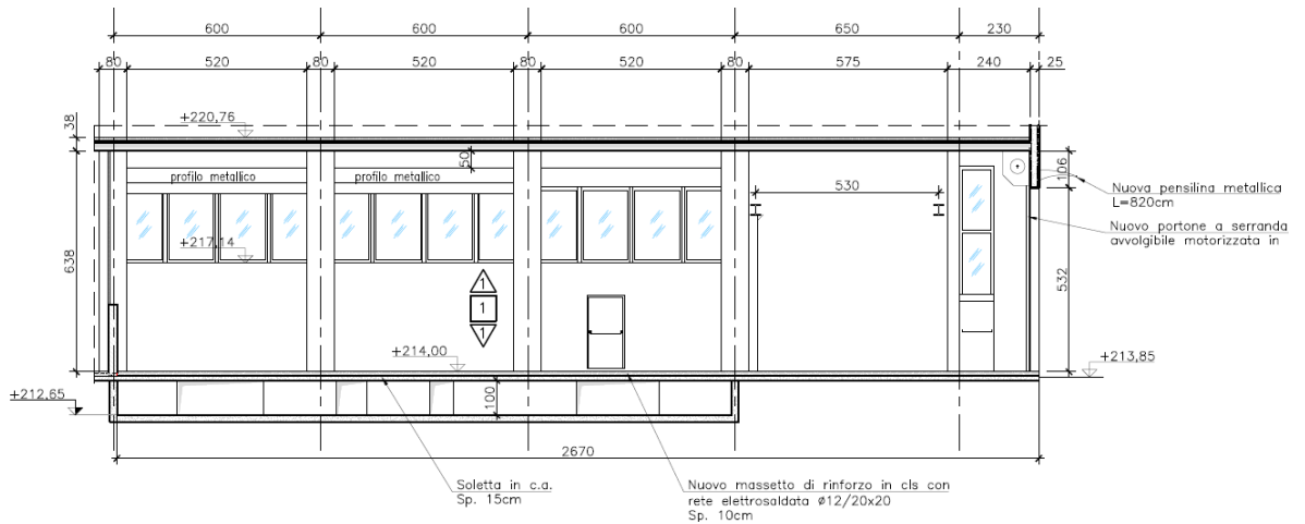
Figura 6-9 Sezione C-C edificio 21n – Post Operam
