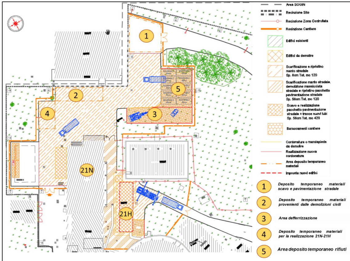
Figura 6-3 Adeguamenti edifici 21n e 21h – Cantierizzazione
