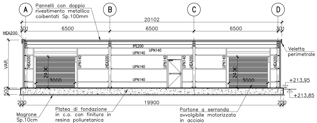
Figura 6–13 Sezione C-C edificio 21h – Post Operam
