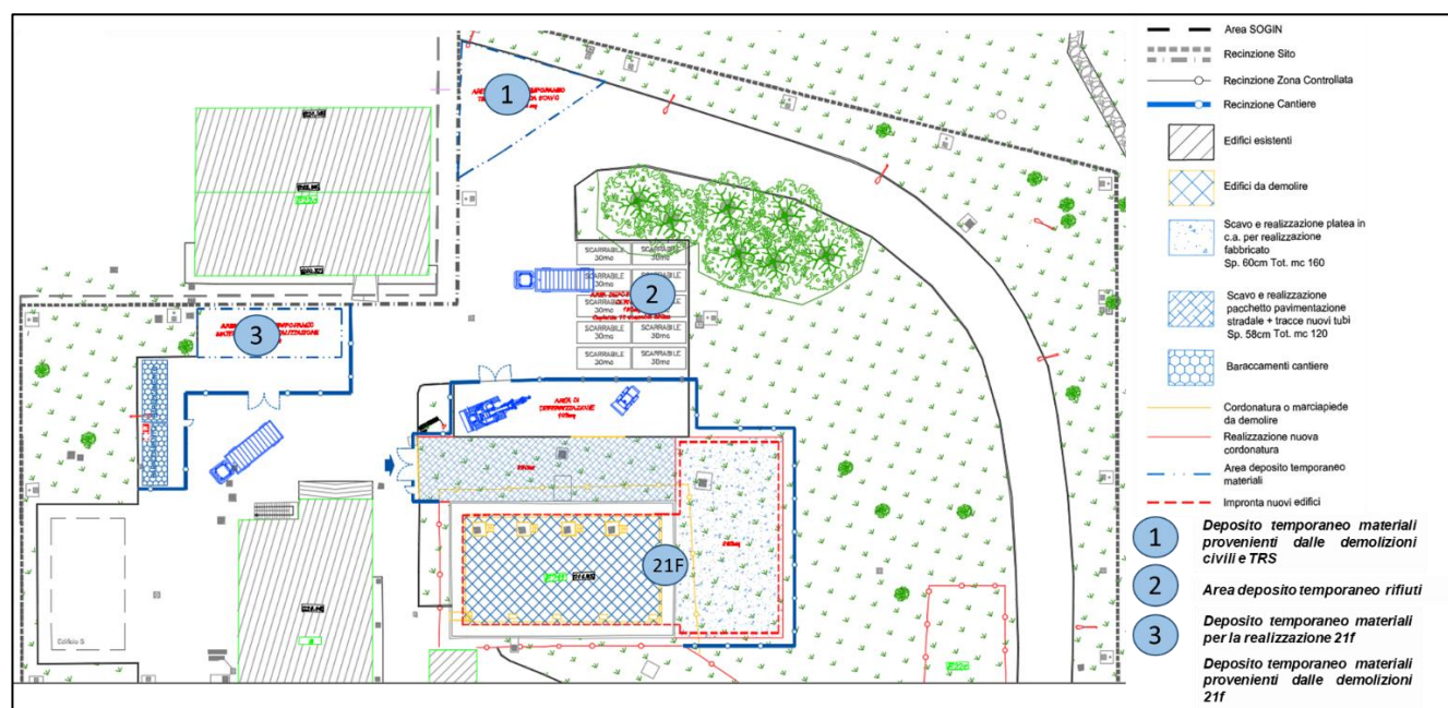
Figura 6–22 Smantellamento edificio 21F – Cantierizzazione
