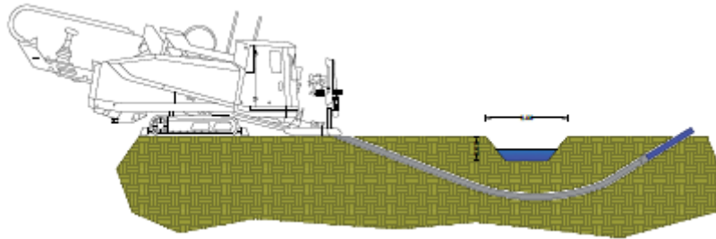
Figura 2: Risoluzione interferenza con Spingitubo
