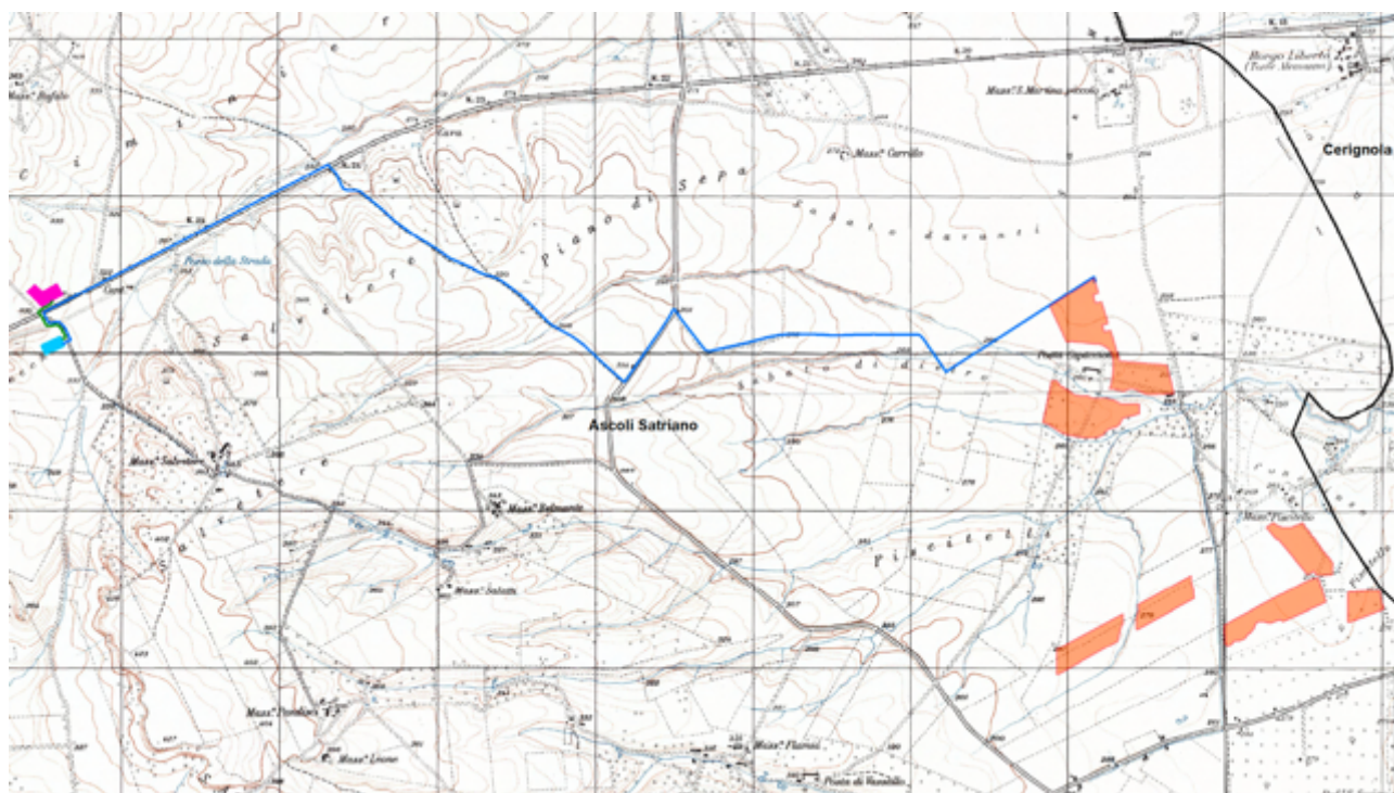
Tavola n. 2 : Impianto con caratteristiche tecniche di connessione alla rete.
