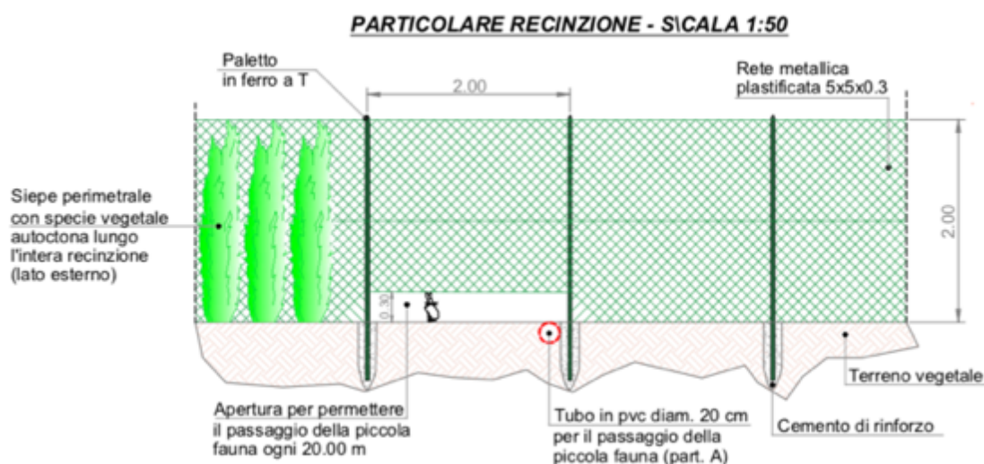
Tavola n. 4: particolare recinzione
