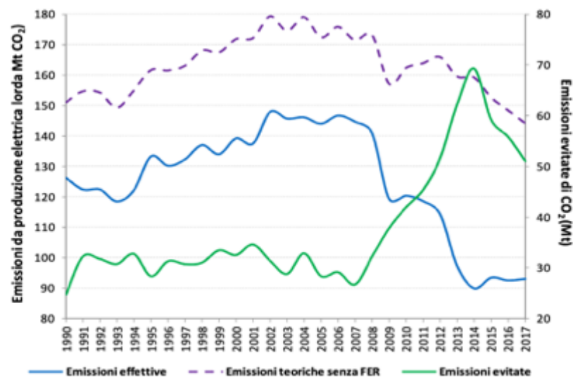
Figura 2.6 - Andamento delle emissioni effettive per la produzione lorda di energia elettrica e delle emissioni teoriche per la produzione di energia elettrica da fonti rinnovabili con equivalente produzione da fonti fossili.
