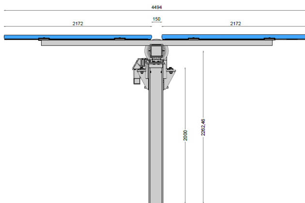
PROSPETTO LATERALE TRACKER - SF7 BI FACIAL
