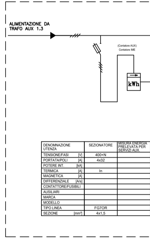
QUADRO CONTATORE SERVIZI AUX CABINA SC3
