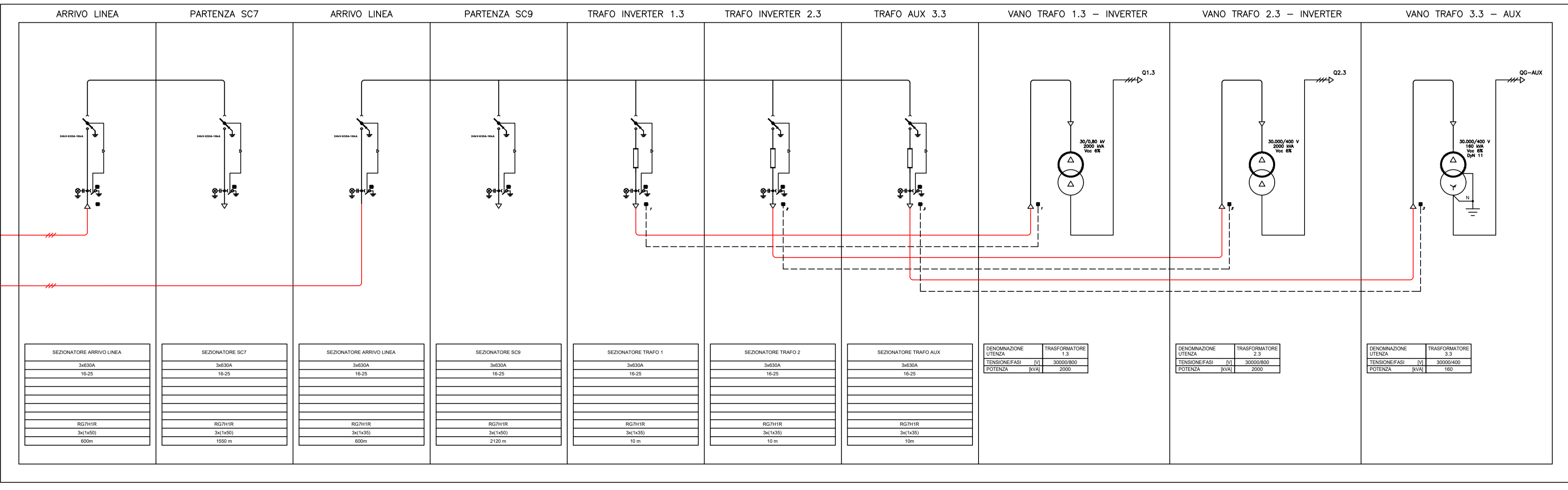
CABINA SOTTOCAMPO 3 - SC3
