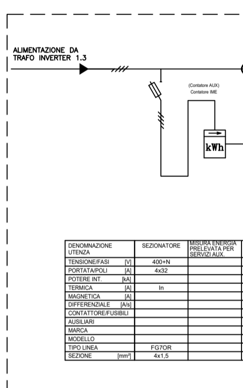
QUADRO CONTATORE PRODUZIONE 1.3 CABINA SC3
