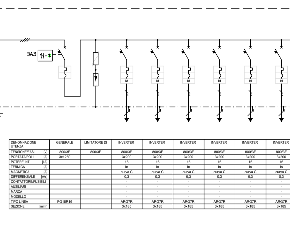
QUADRO SERVIZI AUX CABINA SC3 - LINEE PRIVILEGIATE
