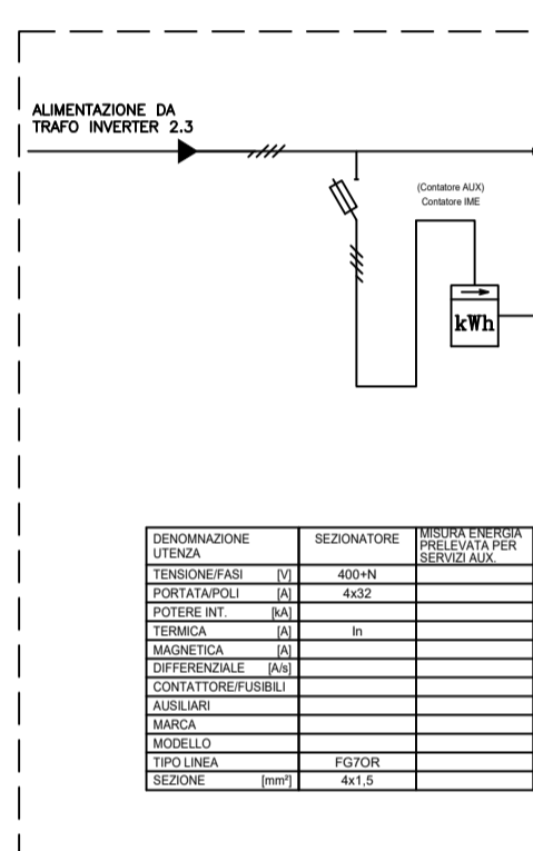
QUADRO SERVIZI AUX CABINA SC3
