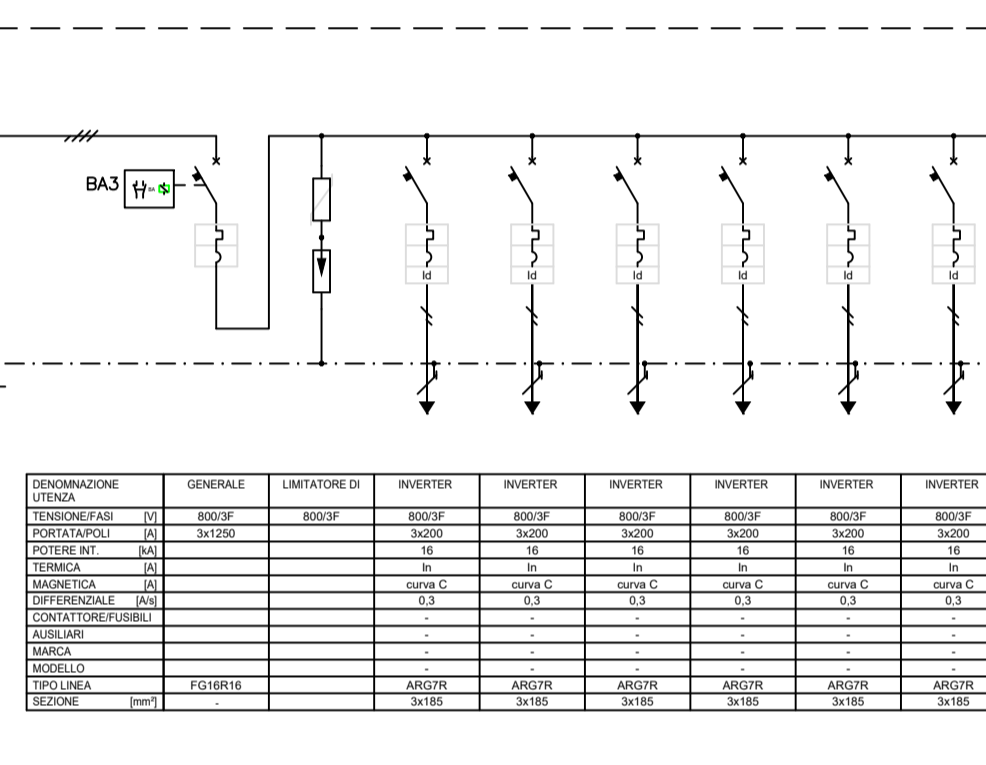
QUADRO CONTATORE SERVIZI AUX CABINA SC3
