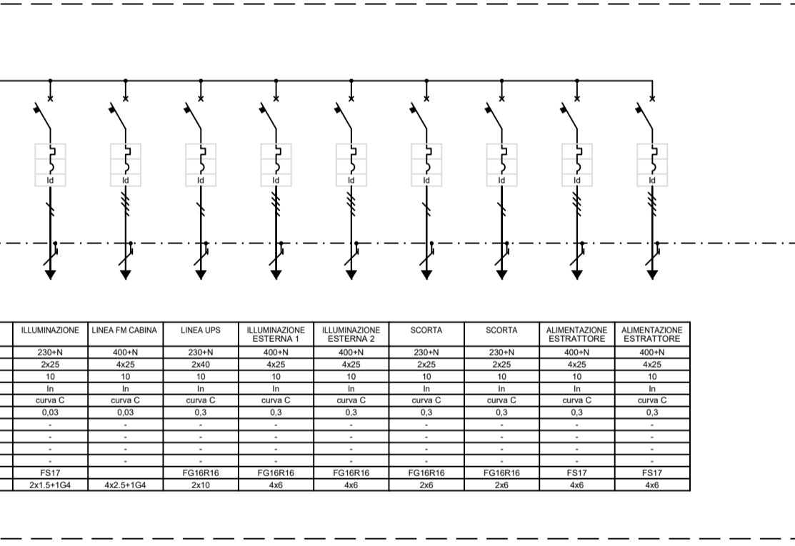
CABINA SOTTOCAMPO 3 - SC3
