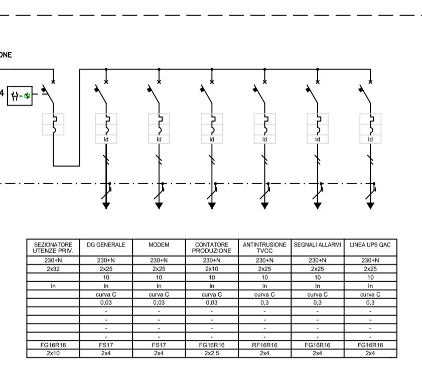
QUADRO SERVIZI AUX CABINA SC7 - LINEE PRIVILEGIATE
