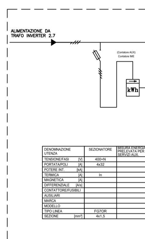
QUADRO CONTATORE PRODUZIONE 2.7 CABINA SC7
