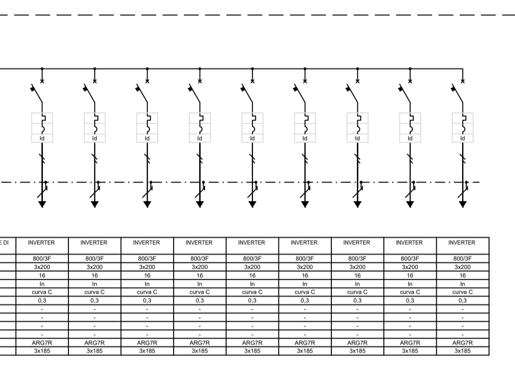
QUADRO SERVIZI AUX CABINA SC7
