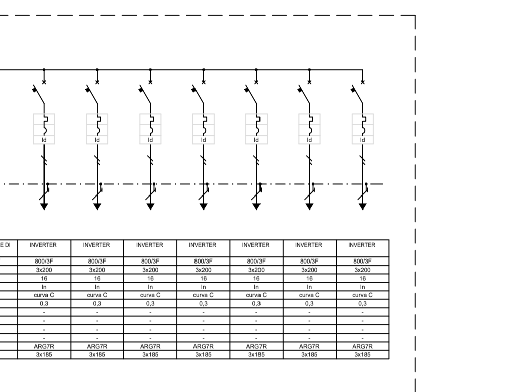
QUADRO SERVIZI AUX CABINA SC7 - LINEE PRIVILEGIATE
