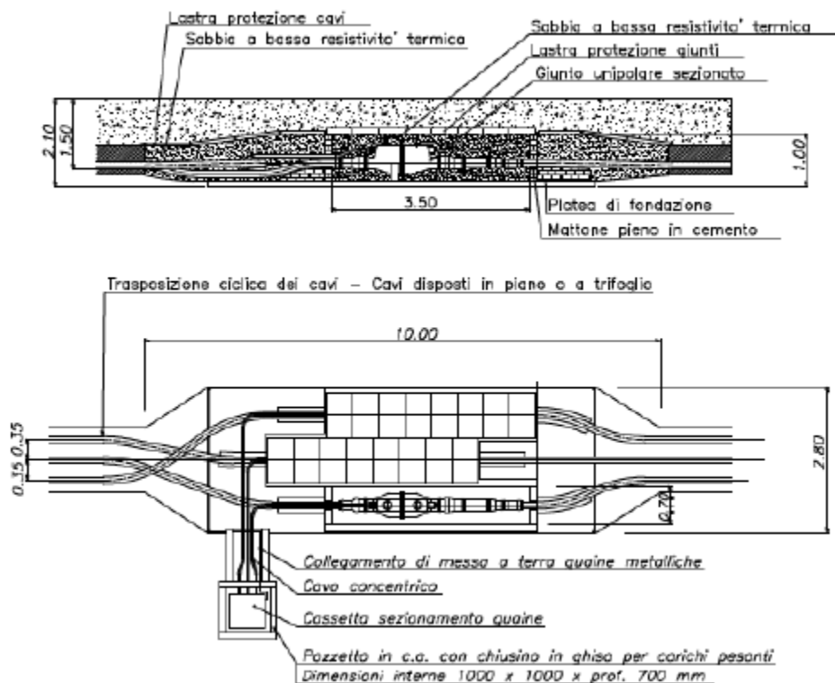
PARTICOLARE BUCA GIUNTI
