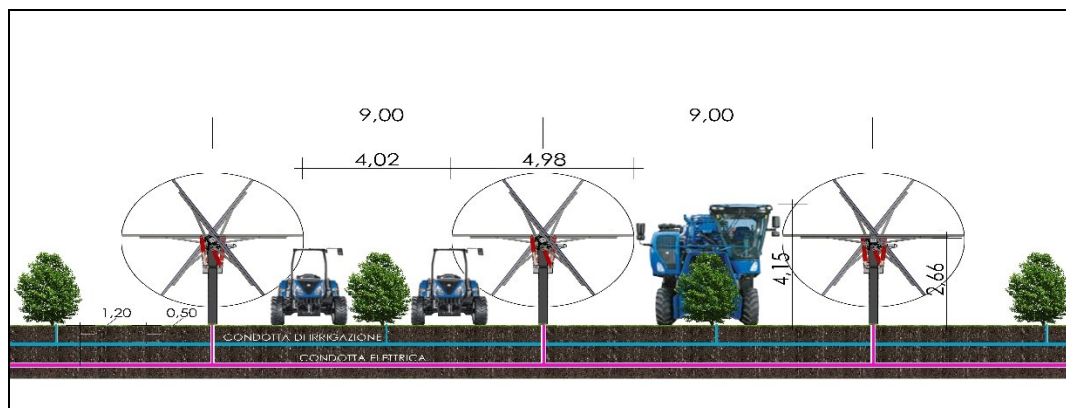
Profilo dell'interfila dell'impianto olivicolo (larghezza m. 9.0)
