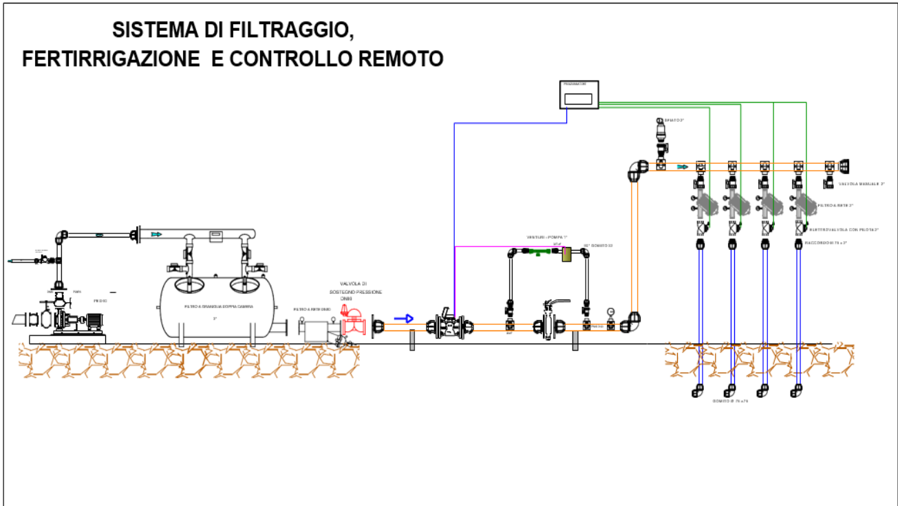
Tav. n. 3 - Sistema di filtraggio, fertirrigazione e controllo remoto
