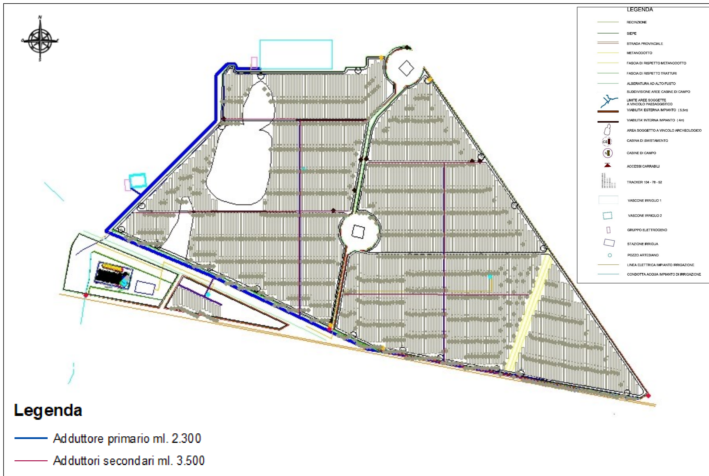
Tav. n. 2 - Schema irriguo Oliveto
