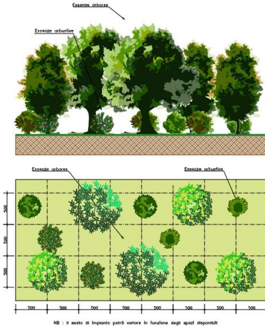
Figura 4-2 MODULO A – Filari alberati: sesto d’impianto e sezione tipologica
