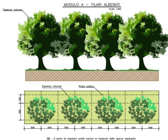
Figura 4-1 MODULO A – Filari alberati: sesto d'impianto e sezione tipologica
