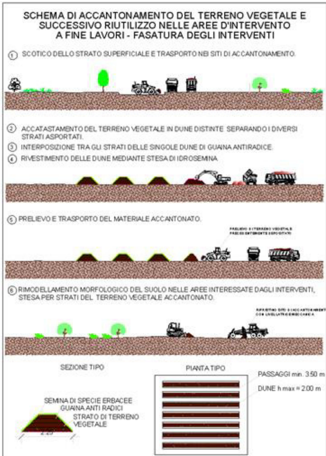
Figura 4-3 – schema di accantonamento del terreno vegetale
