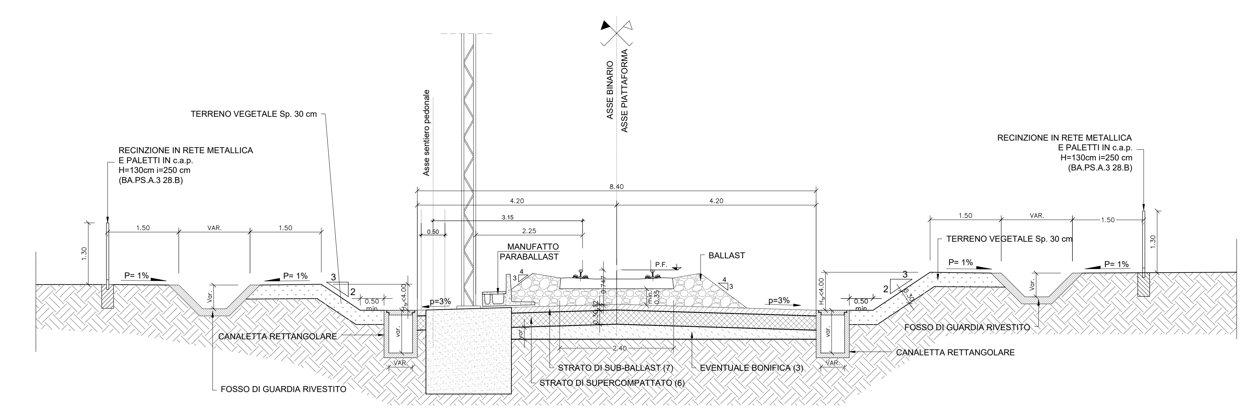
SEZIONE TIPO A SINGOLO BINARIO IN TRINCEA - H/tr<1,00 m SCALA 1:50
