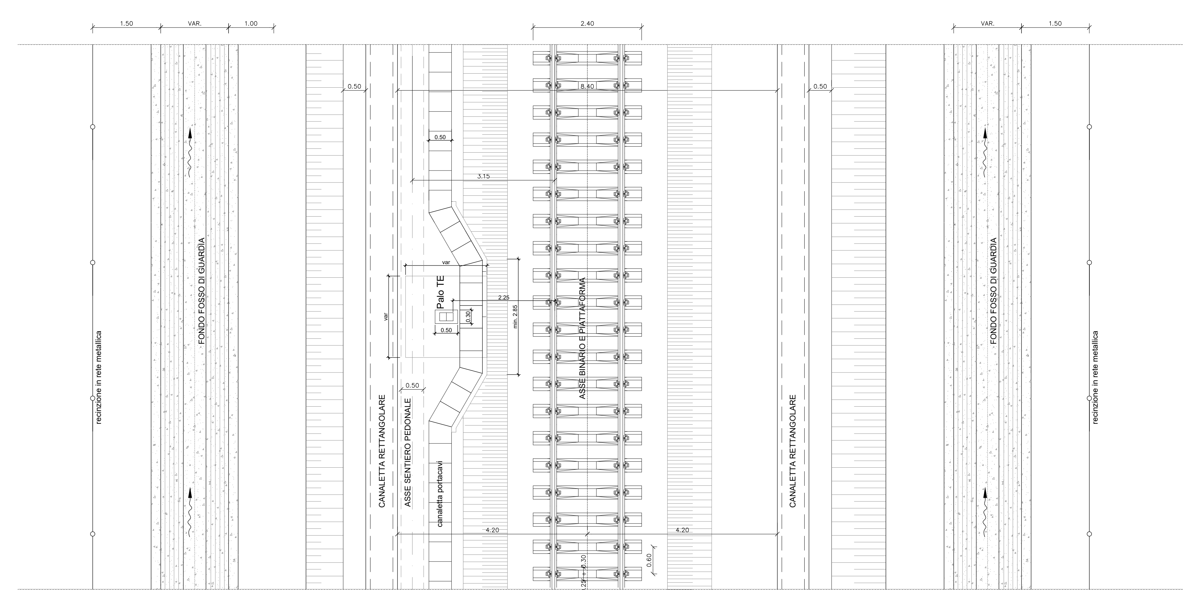
PIANTA PER SEZIONE TIPO A SINGOLO BINARIO IN TRINCEA - H/tr<1,00 m SCALA 1:50
