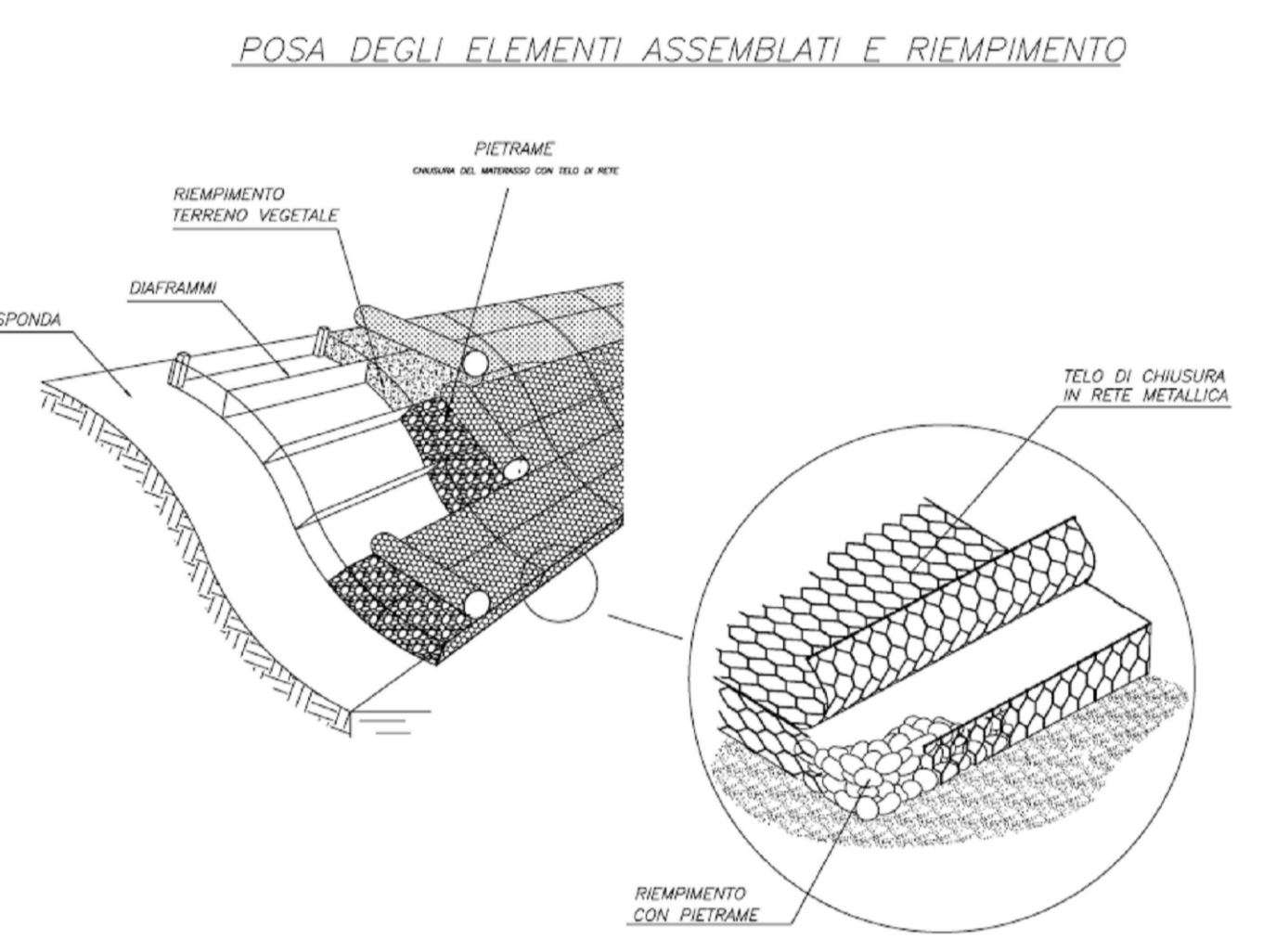
Particolare posa materassi tipo reno
