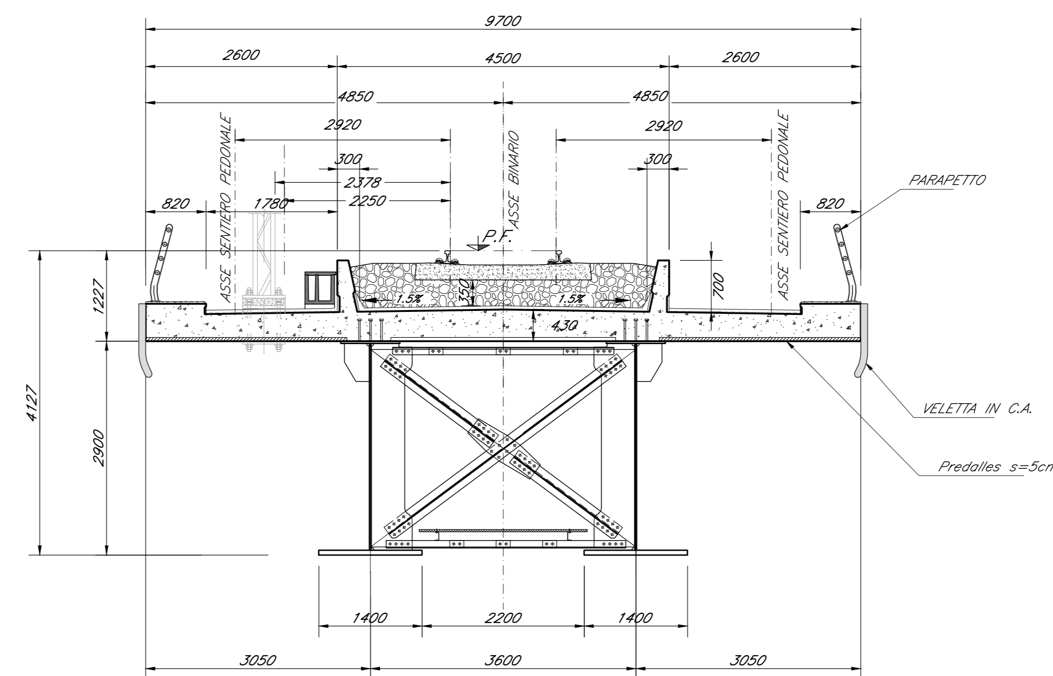
SEZIONE TRASVERSALE B-B
