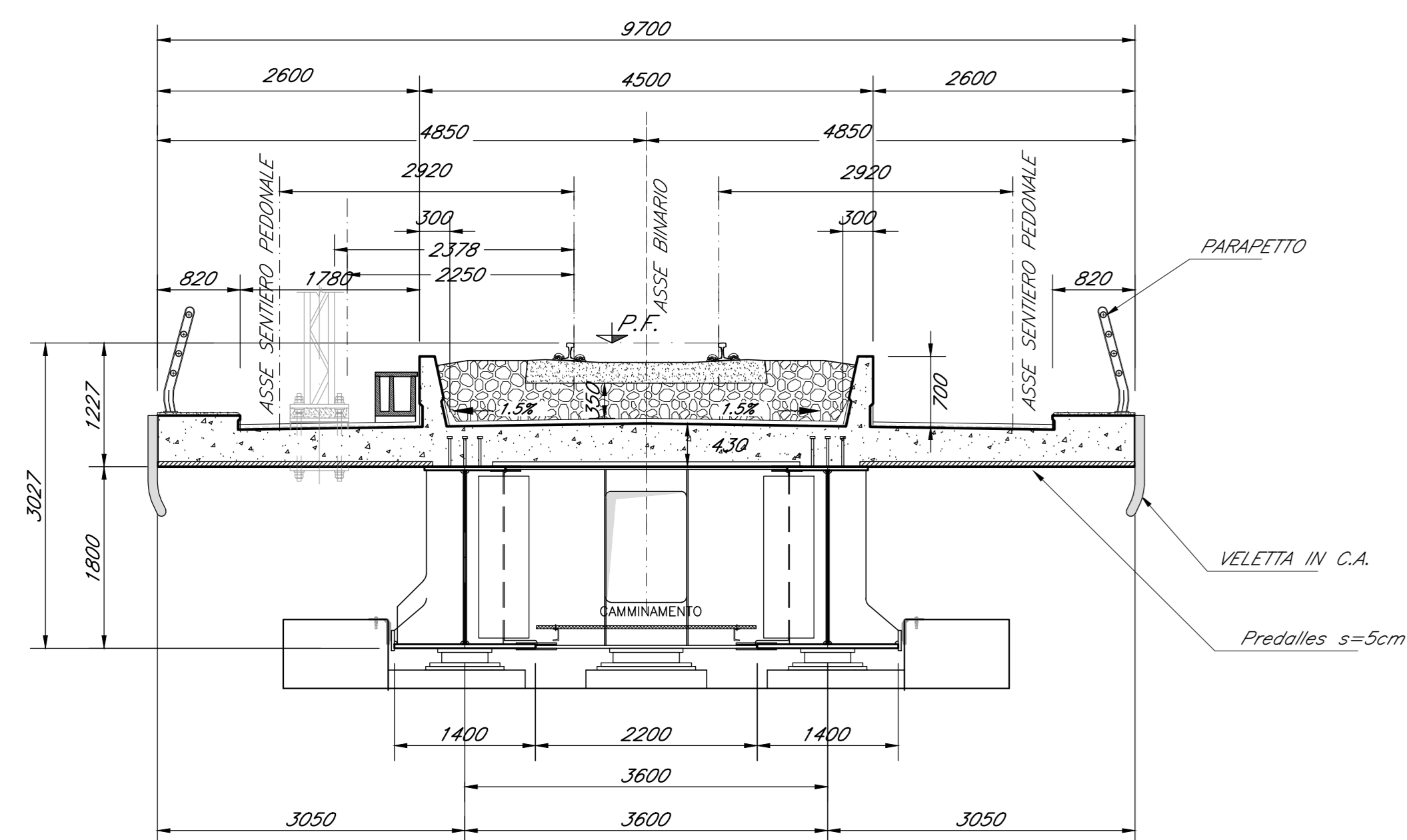
SEZIONE TRASVERSALE A-A
